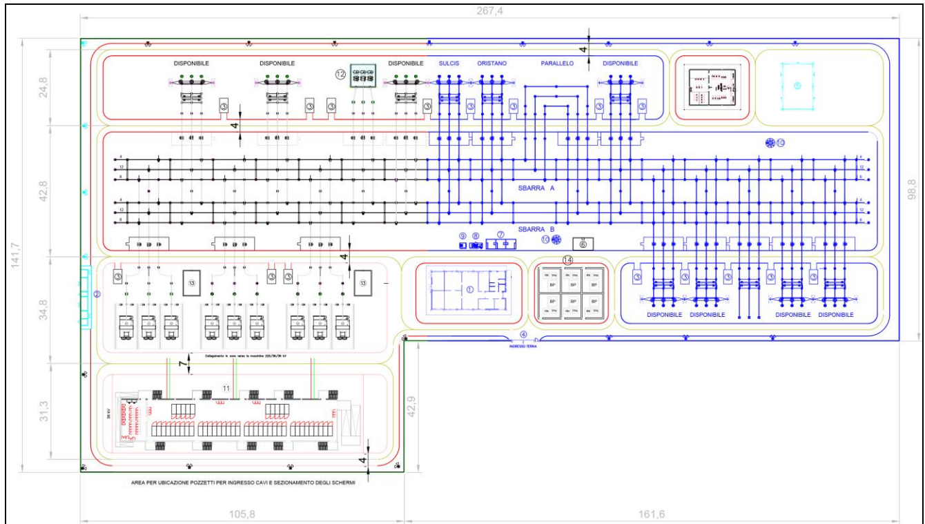
Fig2: Stazione RTN
