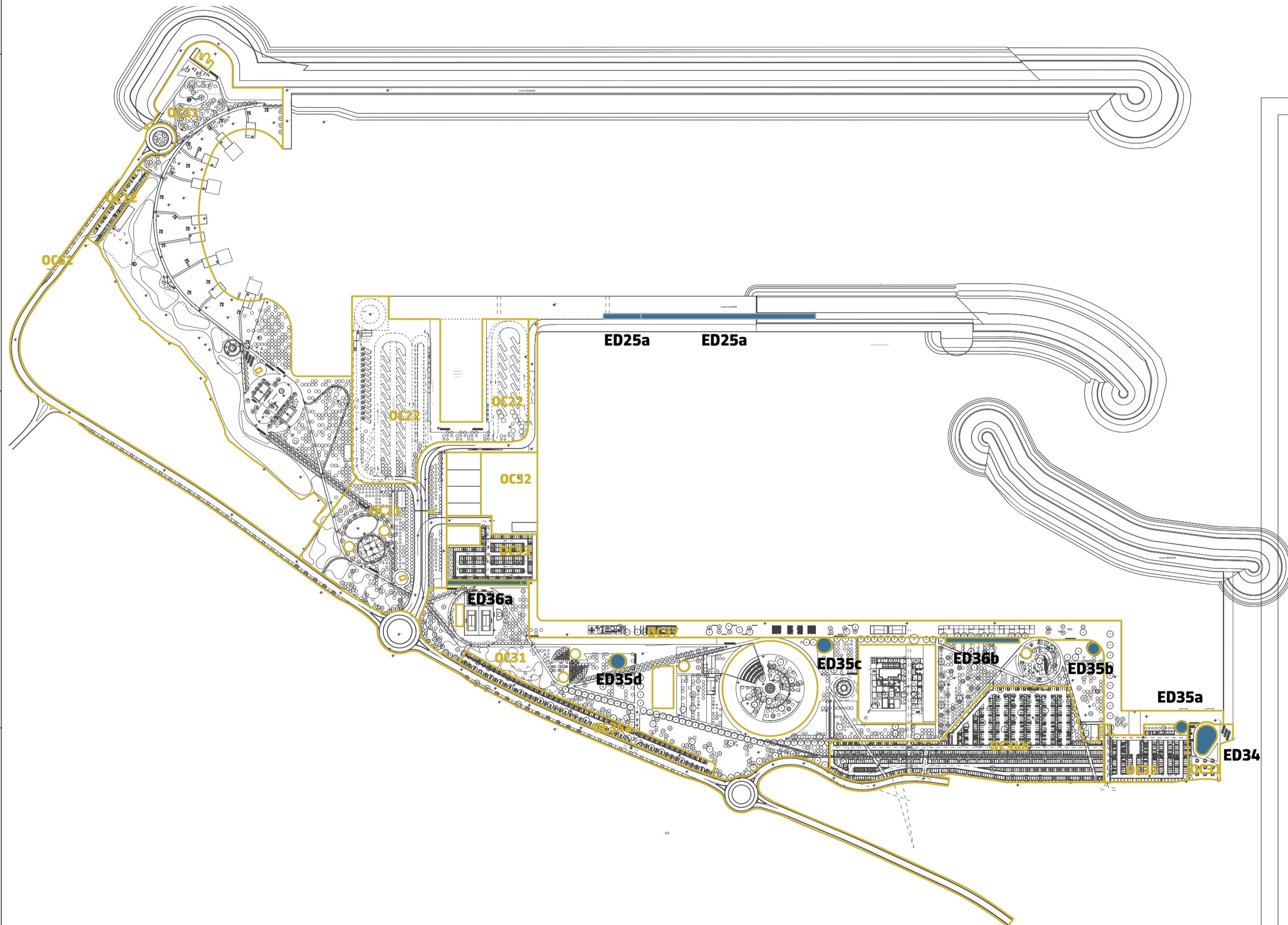
Planimetria generale SERVIZI ALLA MARINA scala 1:4.000
