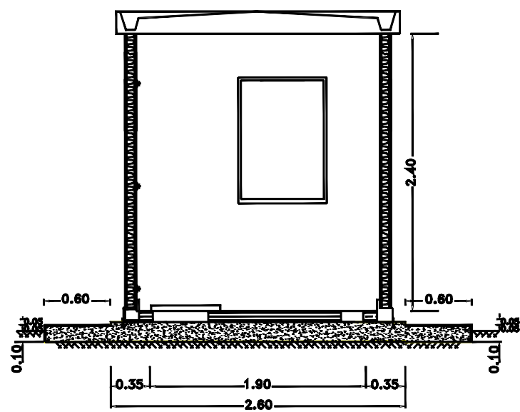
SEZ. A-A
