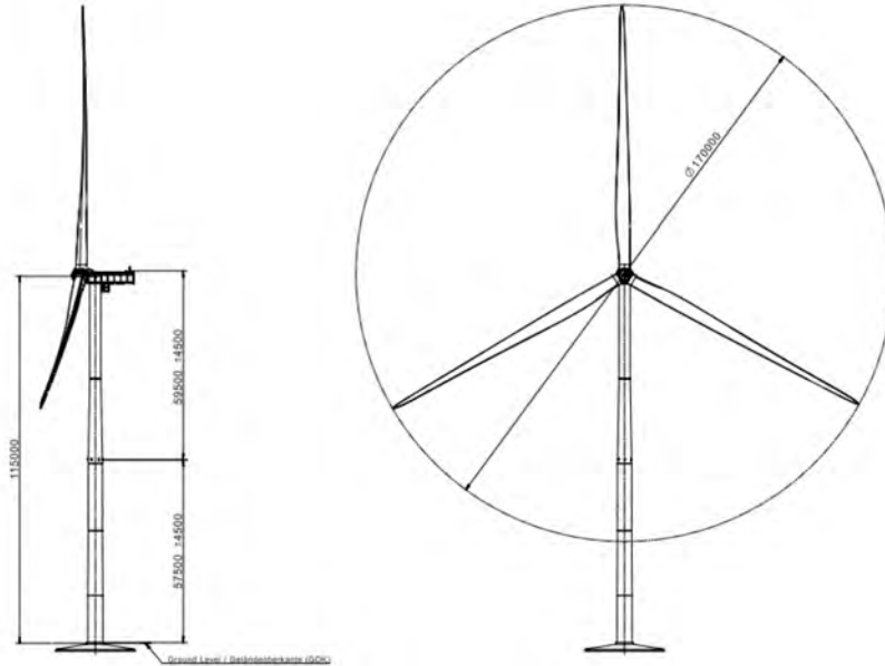
Figura 3 modello SG 6.0-170-115
