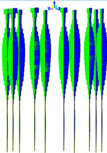
Shear Force 3-3 Diagram (INVILUPPO_SLU+SLV+EXTREME - Max/Min)
