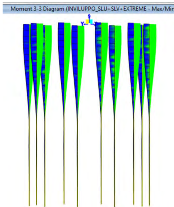
Figura 62 momento 3 pali
