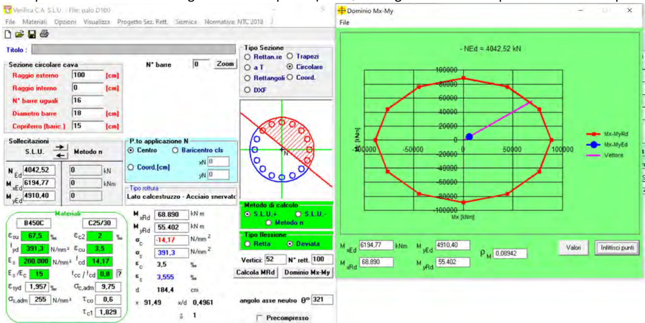
Figura 63 verifica del palo pressoflessione 1
