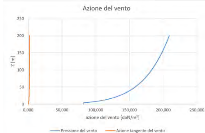
Figura 21 Andamento dell'azione del vento
