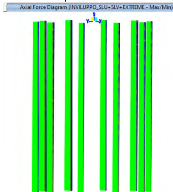
Figura 58 sforzo Normale pali
