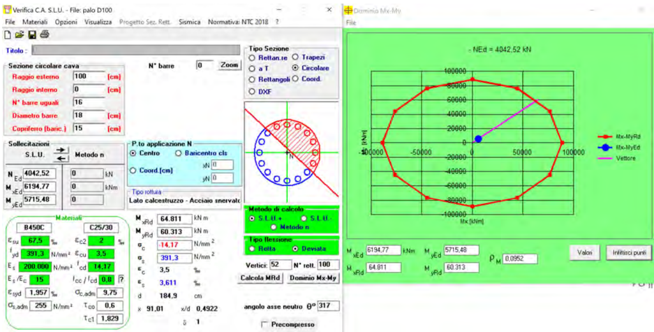
Figura 64 verifica del palo pressoflessione 2
