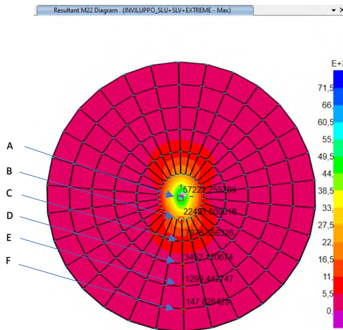
Figura 51 sezioni di riferimento
