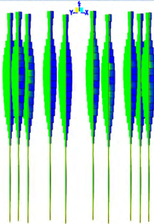
Figura 59 taglio 2 pali
