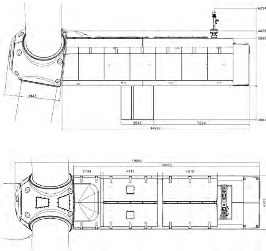
Figura 5 navicella
