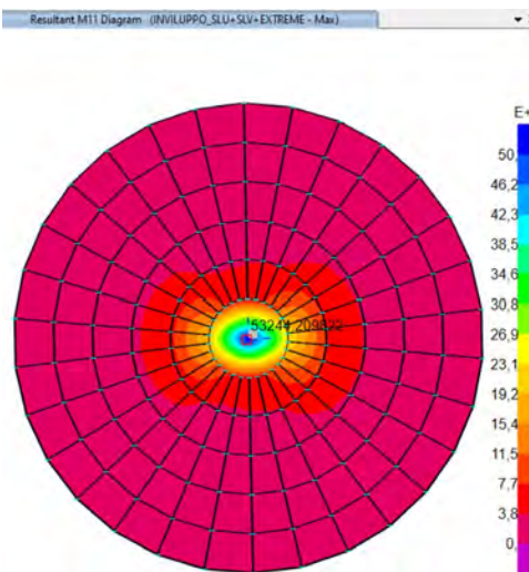
Figura 46 M11 Inviluppo SLU+SLV+EXTREME
