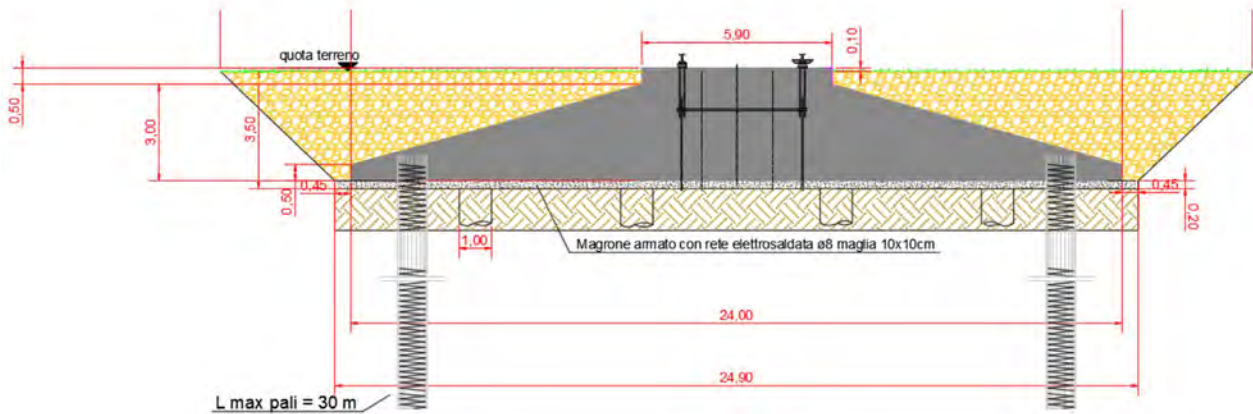
Figura 67 sezione fondazione
