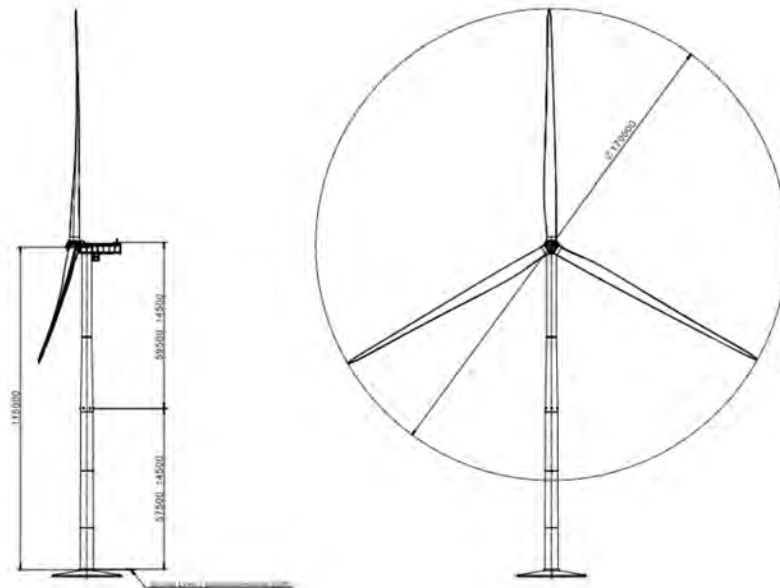
Figura 15 SG. 6.0-170 115
