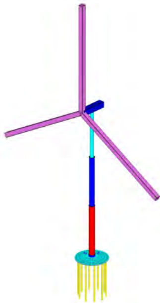
Figura 7 Modello 1 con fondazione
