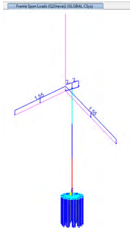
Figura 20 carico neve
