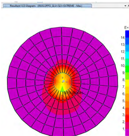
Figura 50 taglio in corrispondenza del cambio di sezione (sezione di cambio di pendenza)
