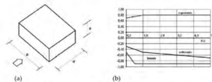
a) Parametri caratteristici di edifici a pianta rettangolare. b) Edifici a pianta rettangolare: c_p per facce sopravvento, sottovento e laterali
