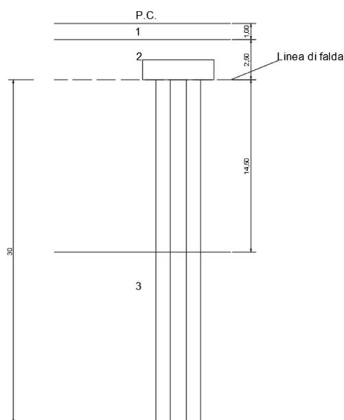
Figura 6 stratigrafia terreno (vedi relazione geologica)
