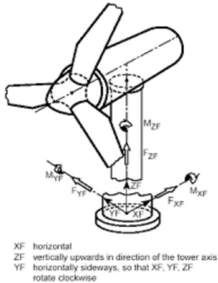
Figura 16 sistema di riferimento XYZ
