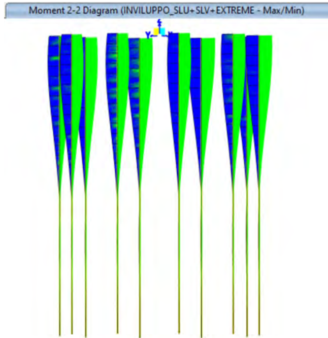
Figura 61 momento 2 pali
