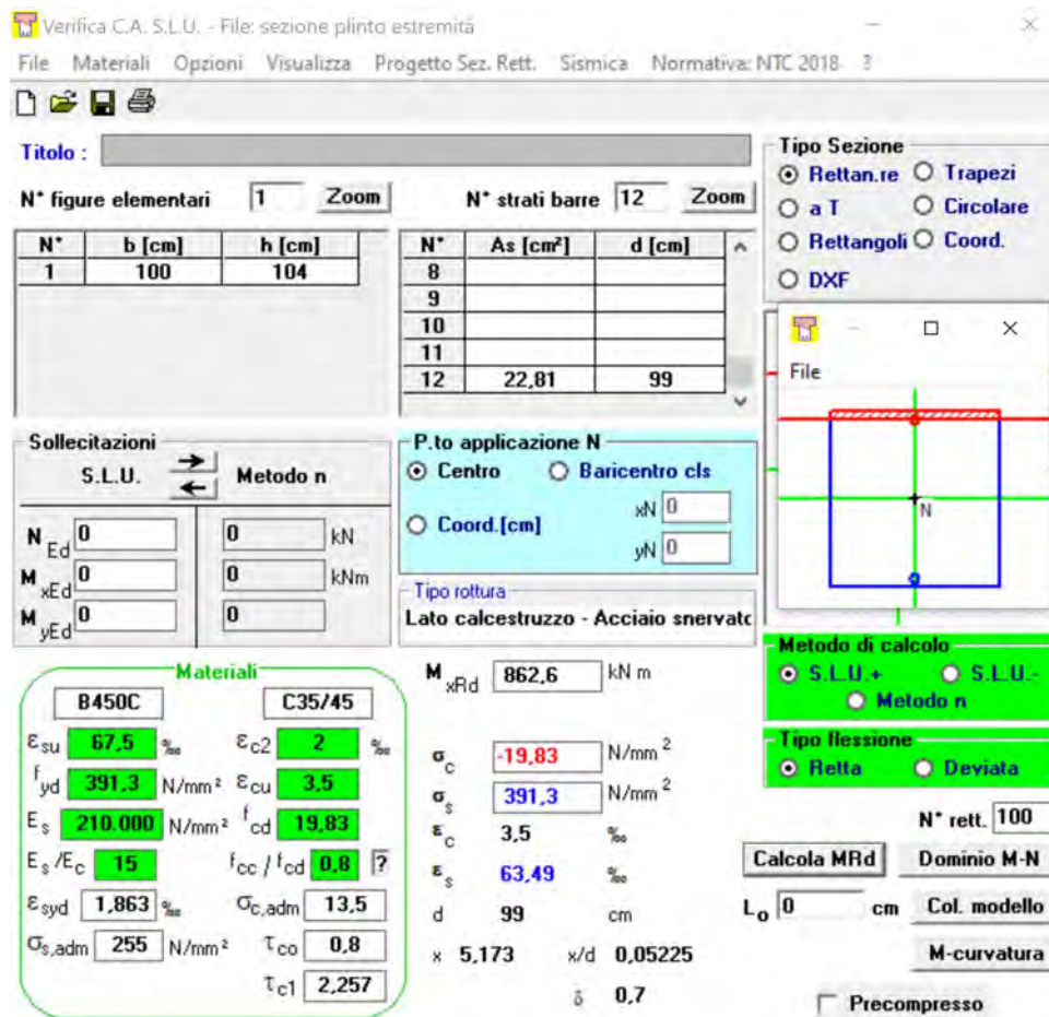
Figura 57 sezione F
