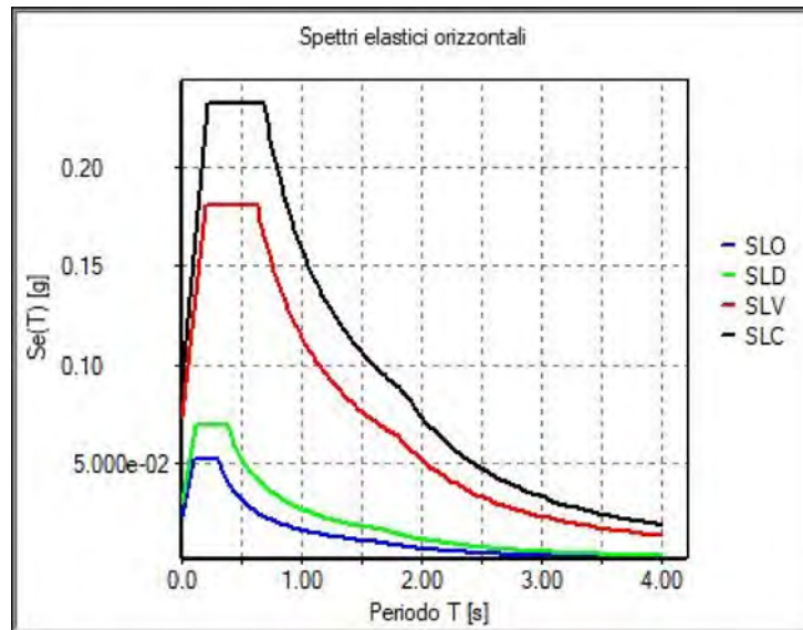
Figura 30 spettri elastici
