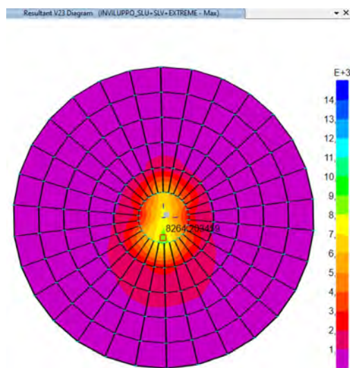
Figura 49 V23 Inviluppo SLU+SLV+EXTREME
