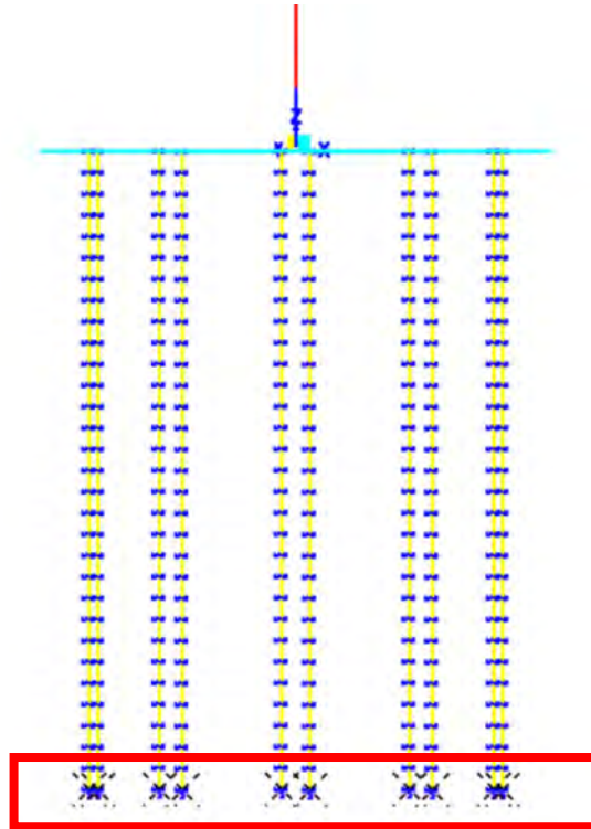
Figura 41 nodi alla punta dei pali
