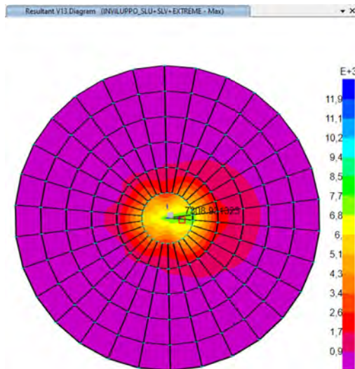
Figura 48 V13 Inviluppo SLU+SLV+EXTREME
