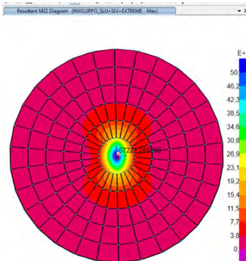
Figura 47 M22 Inviluppo SLU+SLV+EXTREME
