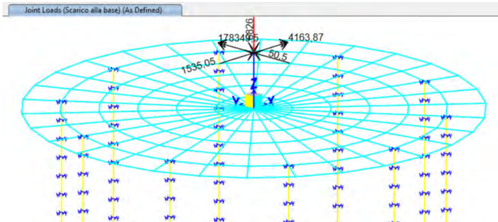
Figura 17 scarichi alla base NON Fattorializzati
