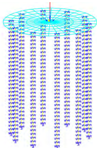
Figura 13 modello fondazione e posizione del sistema di riferimento
