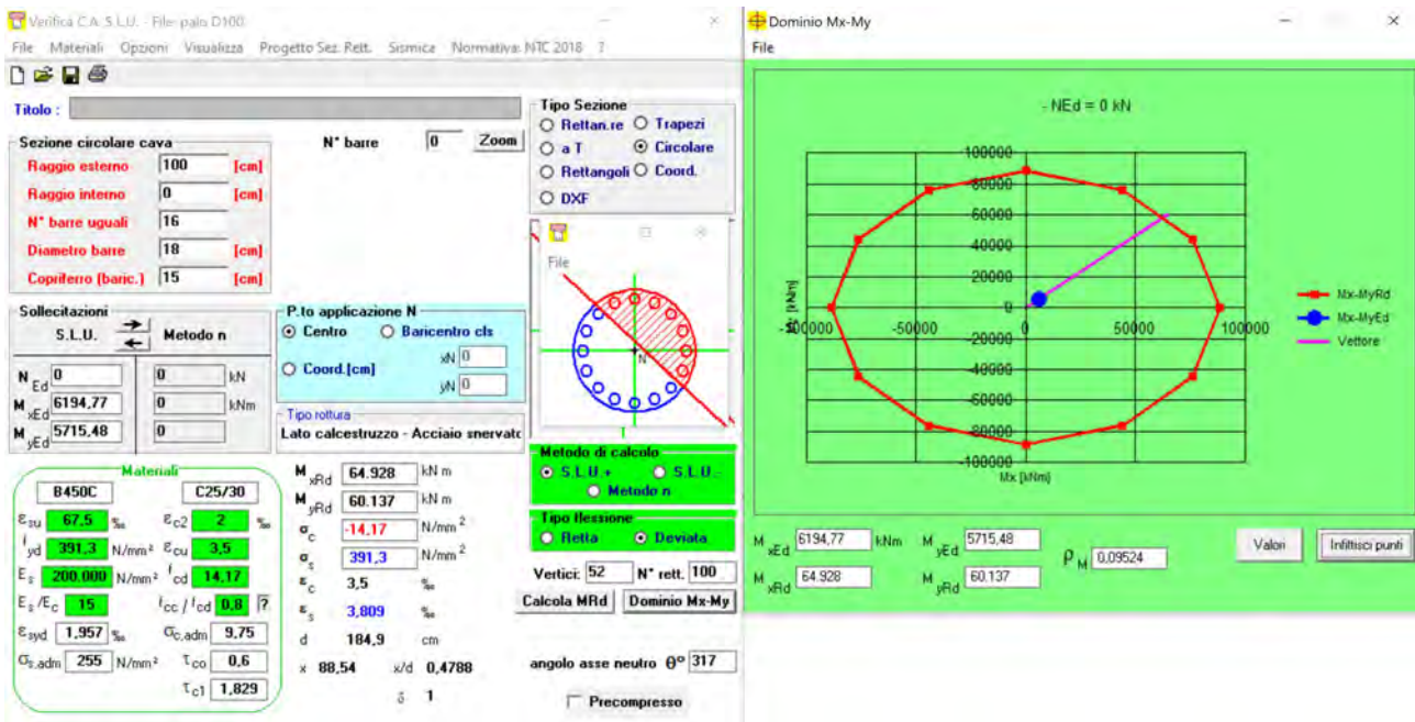
Figura 65 verifica del palo pressoflessione 3
