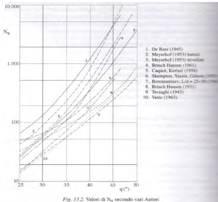
Figura 68 valori di N_q
