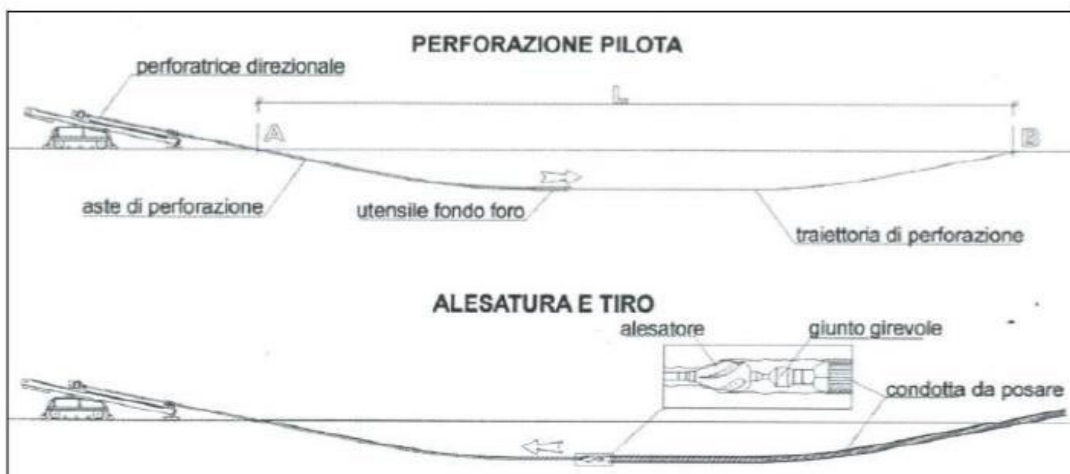
Schematico di Trivellazione Orizzontale Controllata
