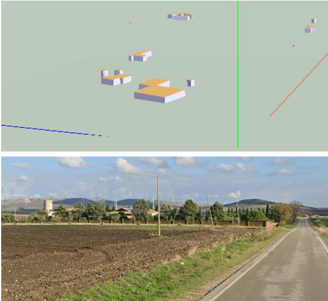
Figura 3-6 Esempio di modellazione 3D del terreno – Cantiere Mobile
