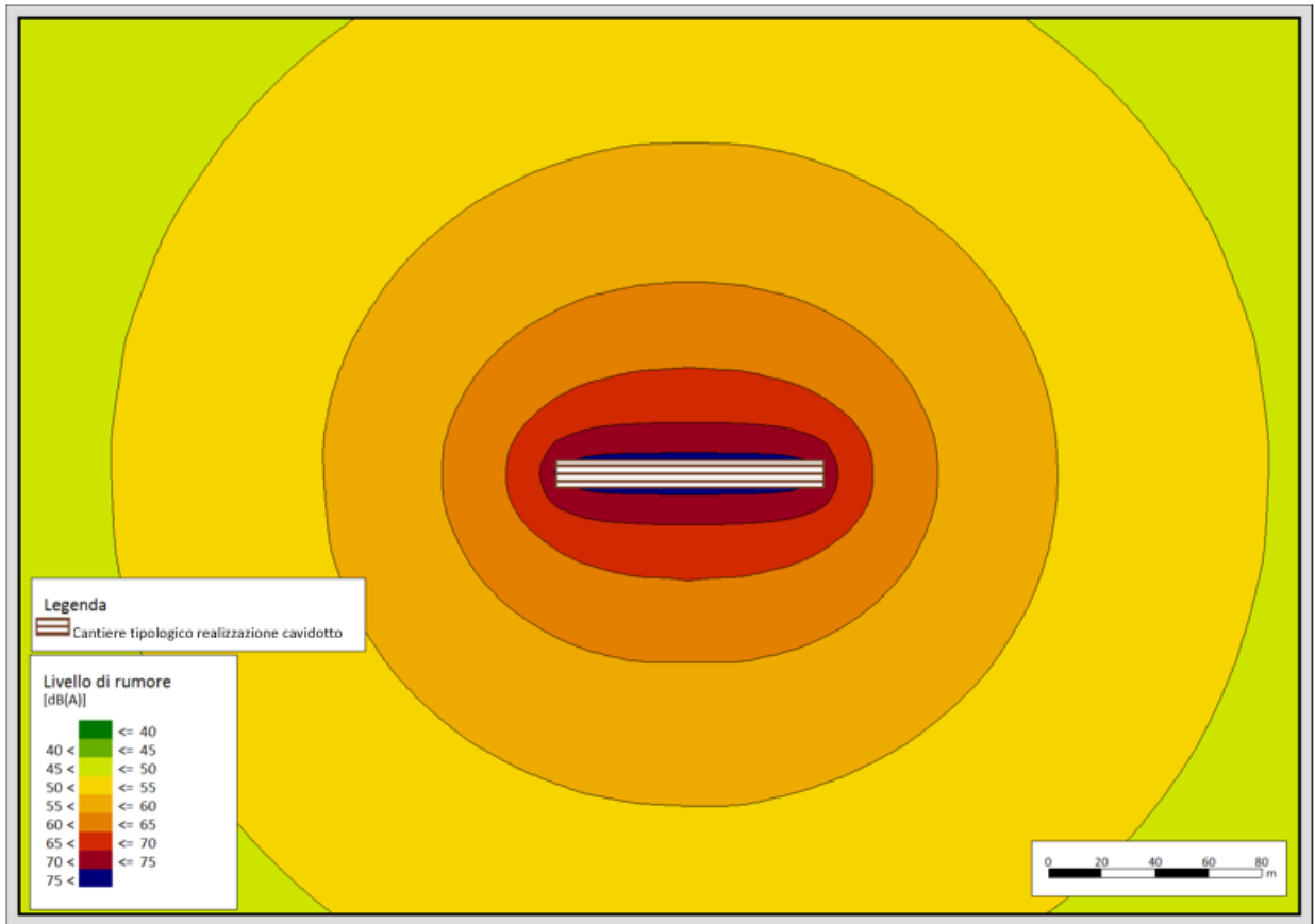
Figura 3-7 Mappatura acustica in planimetria: cantiere mobile connesso alla realizzazione del cavidotto
