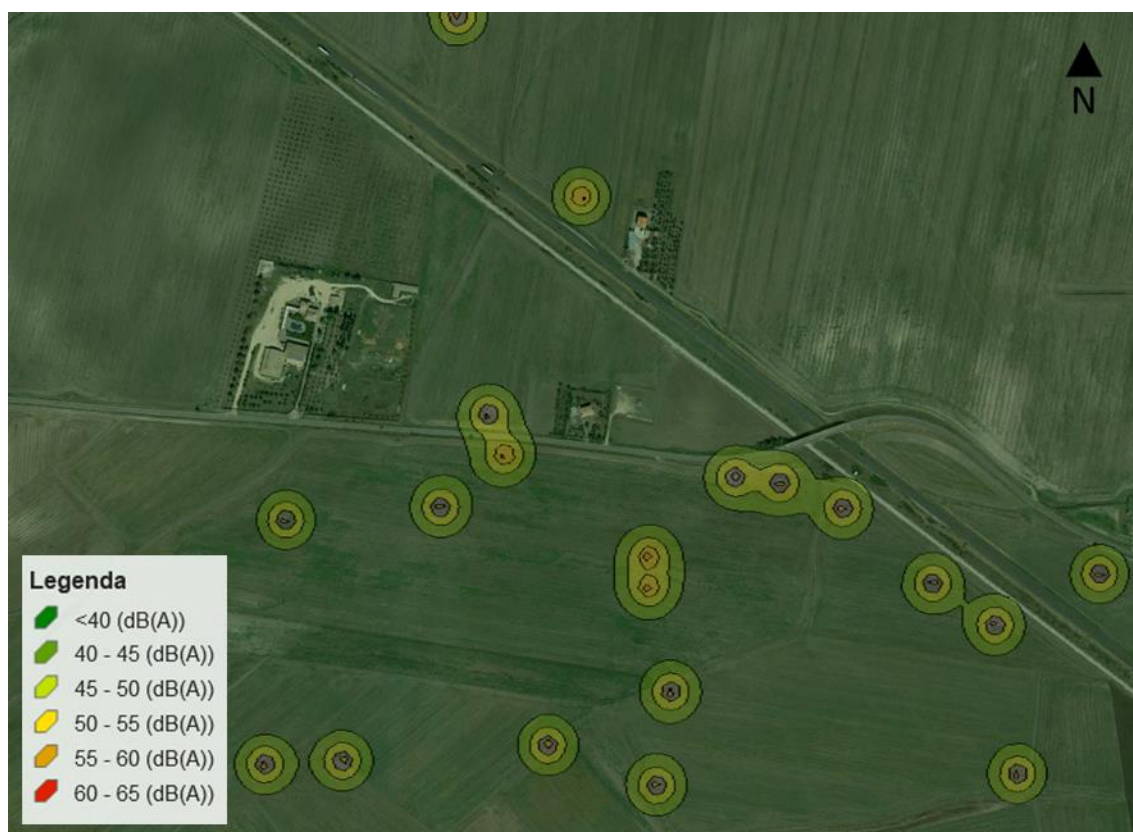
Figura 4-5 Stralcio mappa rumore - Fase di Esercizio
