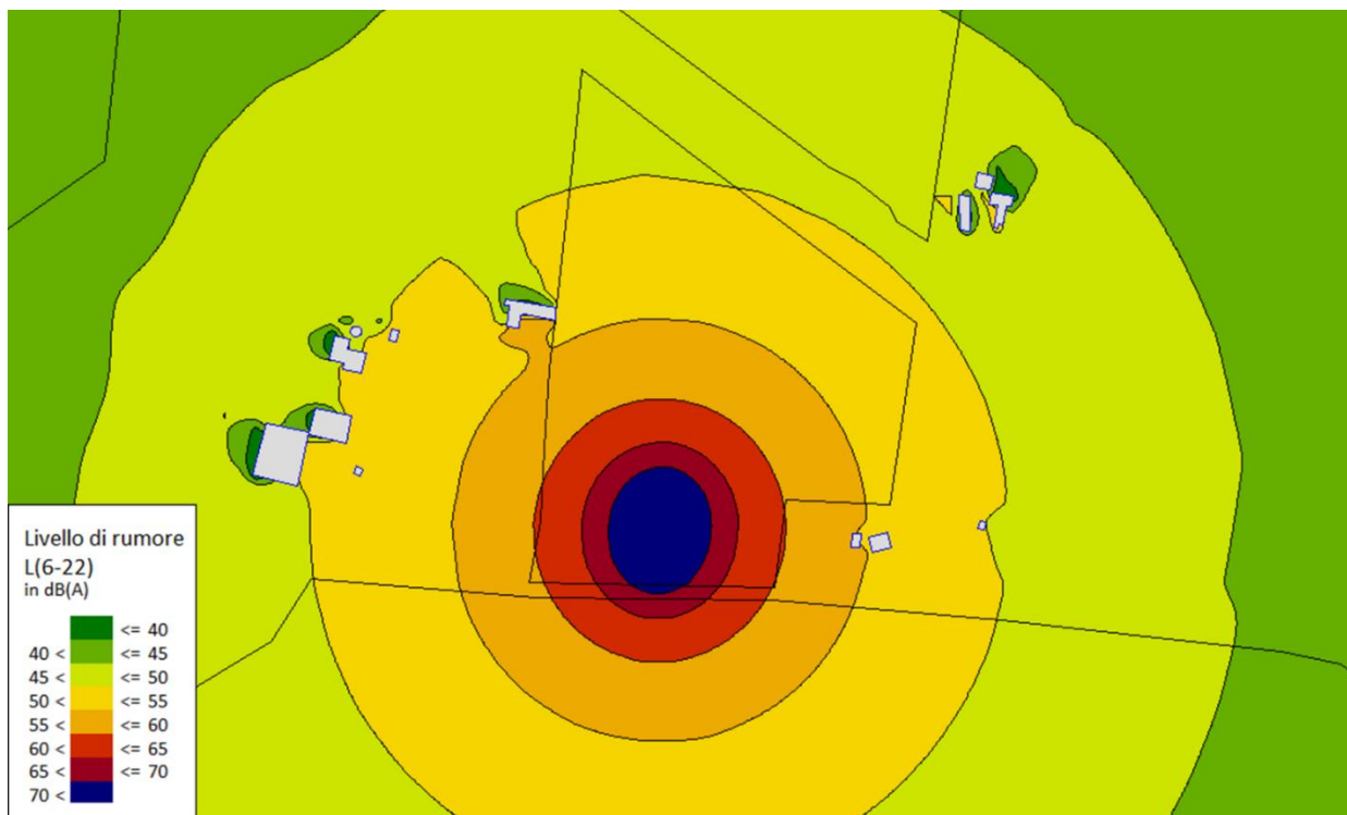
Figura 3-3 Stralcio mappa rumore Cantiere Base
