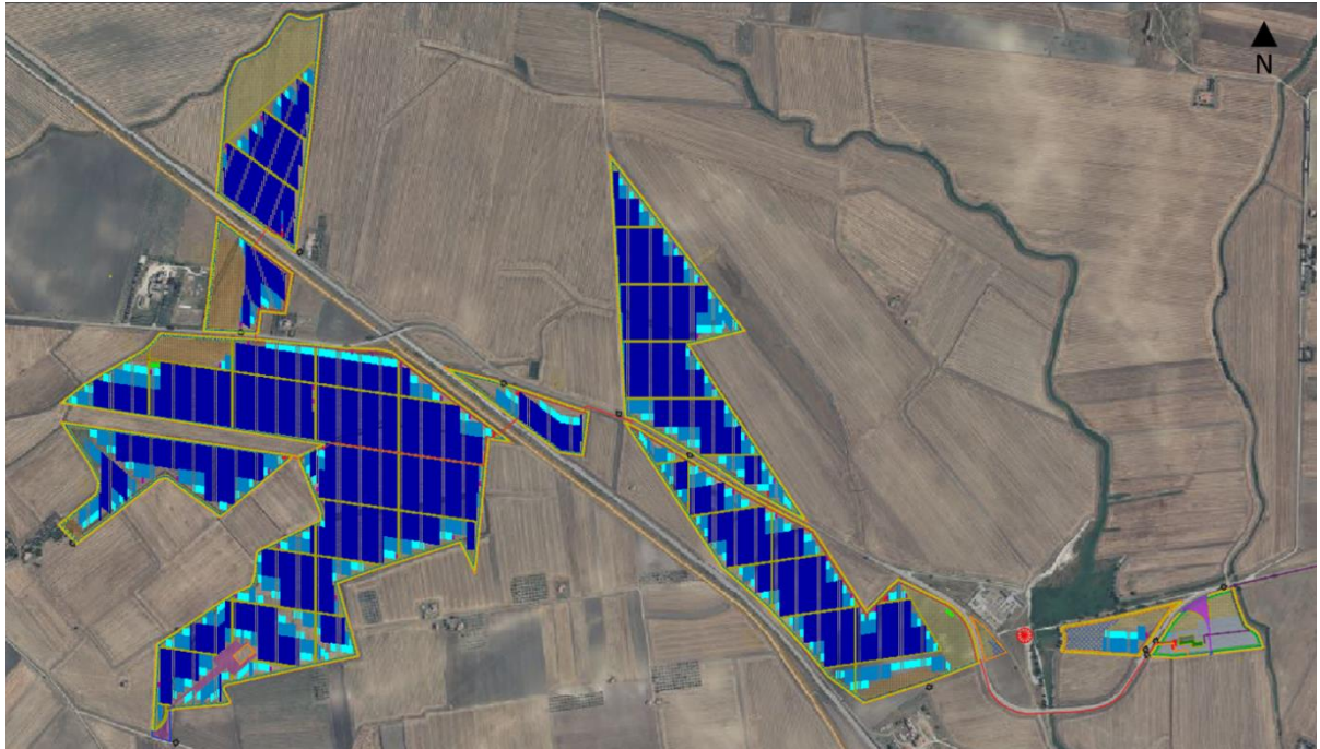
Figura 4-2 Layout impianto agrovoltaiico con posizione cabine inverter
