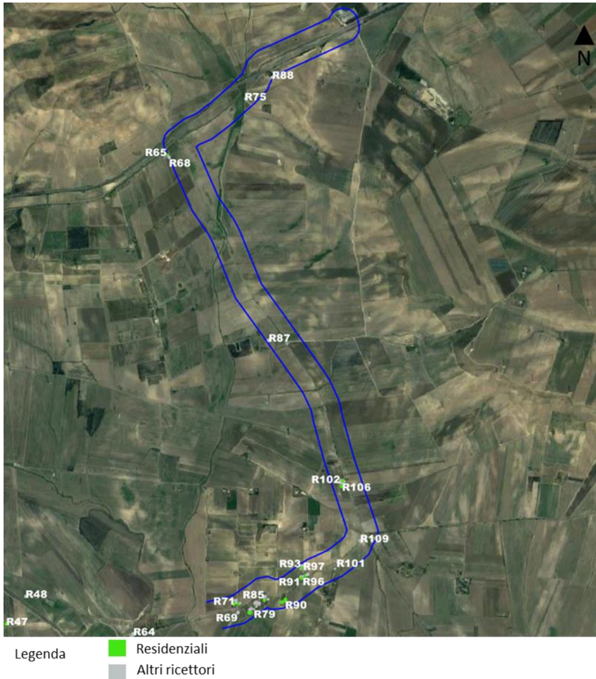
Figura 3-5 Localizzazione scenario di simulazione Cantiere Mobile
