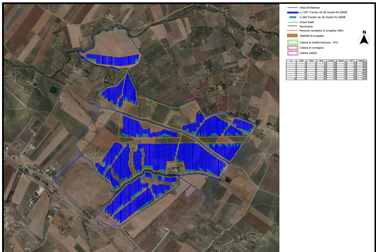
Layout impianto su base ortofoto - "Impianto fotovoltaico Erice 57"
