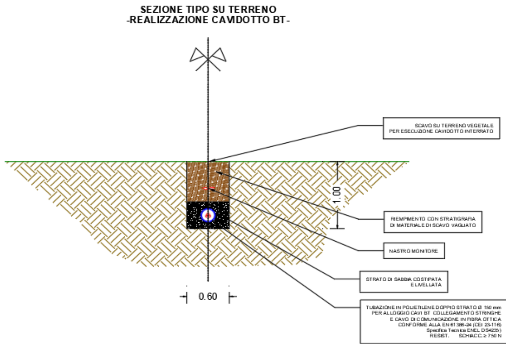
Figura 1.4 Particolare sezione tipo cavo interrato BT
