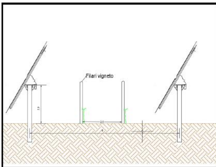
Figura 10 – Dettagli interfila con vigneto
