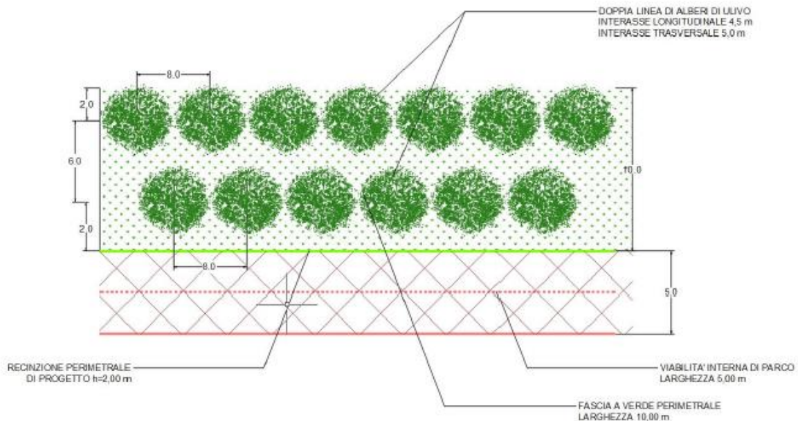
Figura 9 – Dettagli fascia perimetrale
