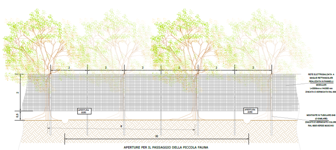
Figura 7 – Prospetto recinzione perimetrale con mitigazione
