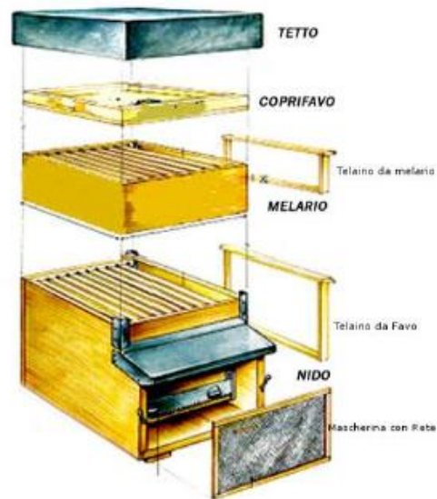
Figura 11 – Componenti dell'arnia
