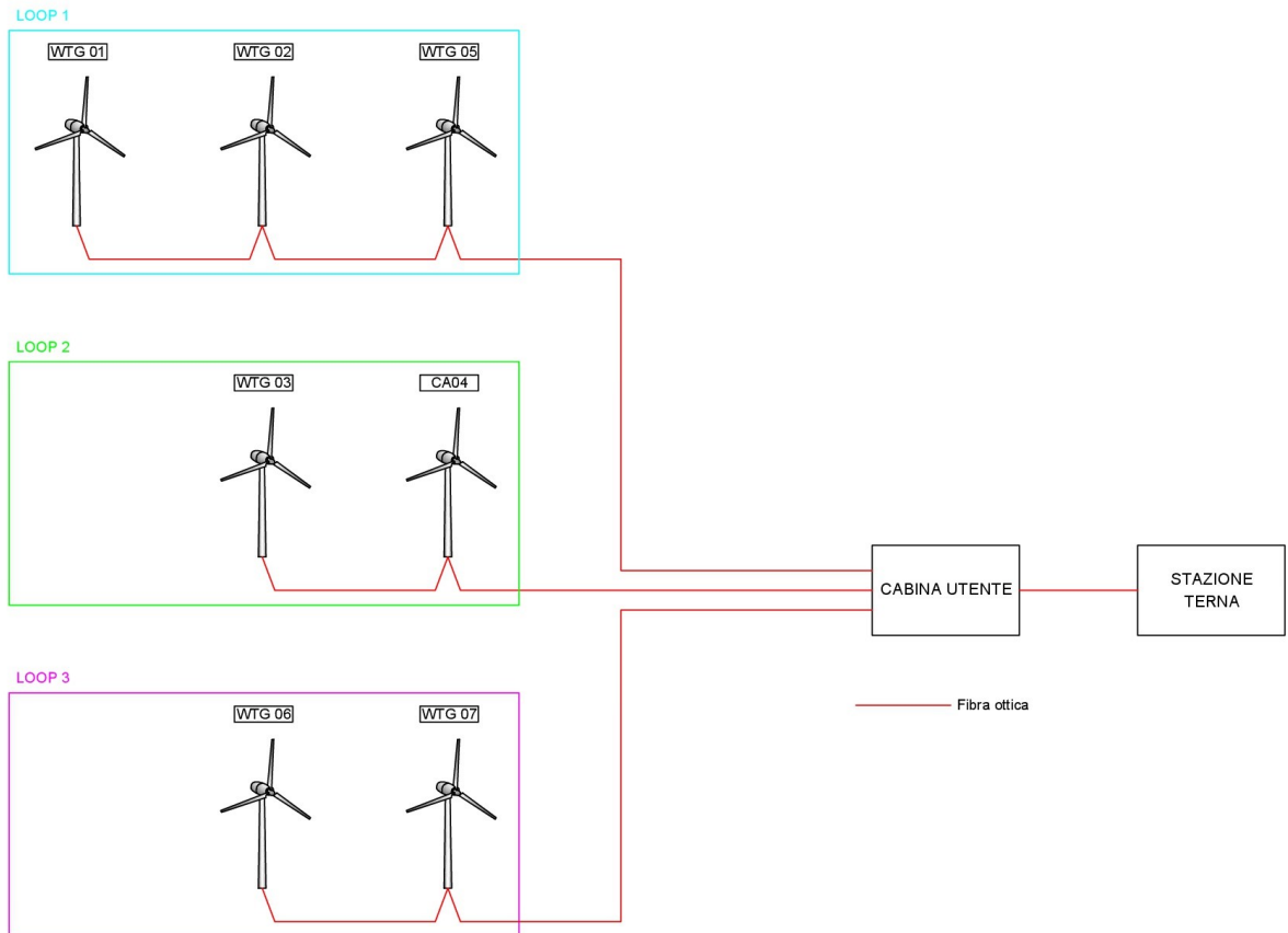
Figura 3 - Schema fibra ottica
