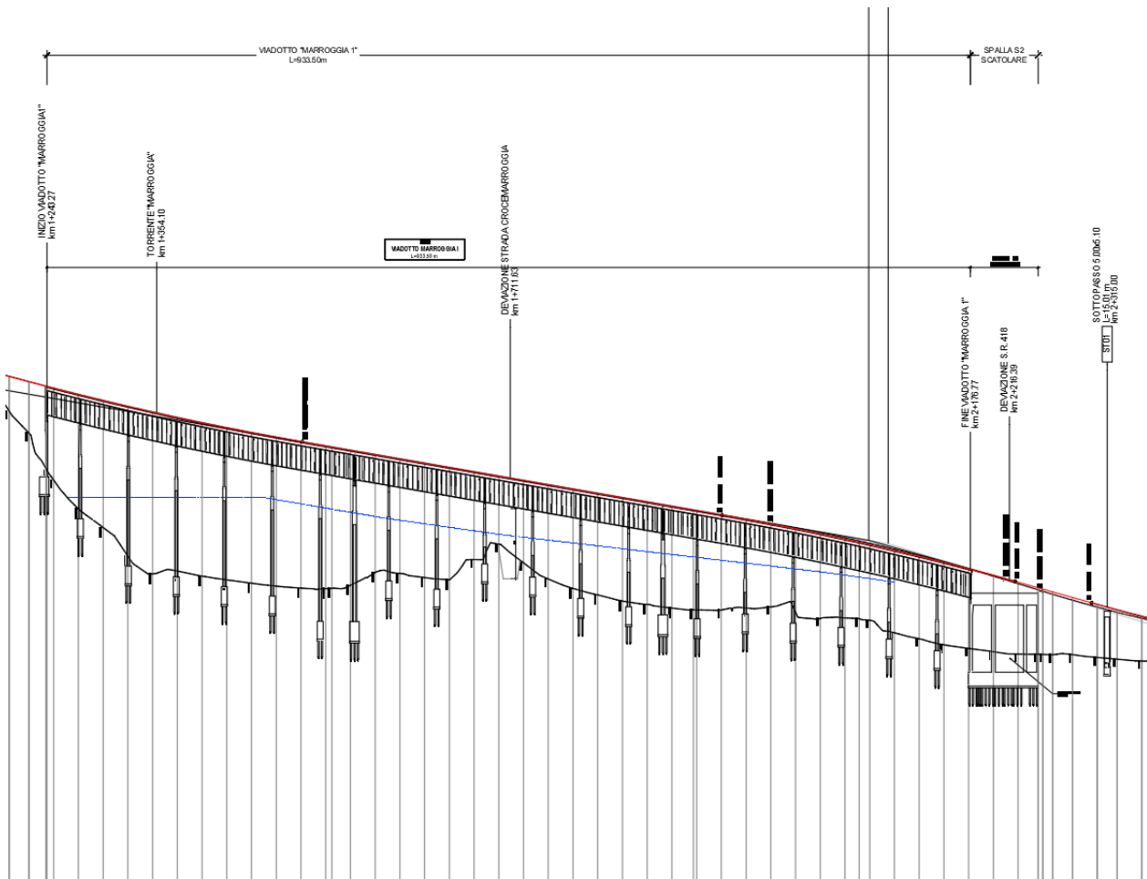
Figura 7 - Stralcio profilo del Viadotto Marroggia.
