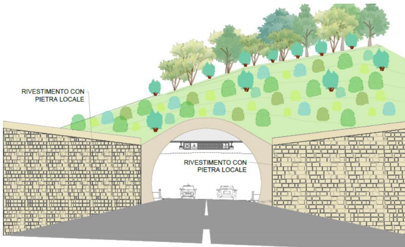
Figura 12 – Sezione di imbocco Galleria artificiale Romanella.
