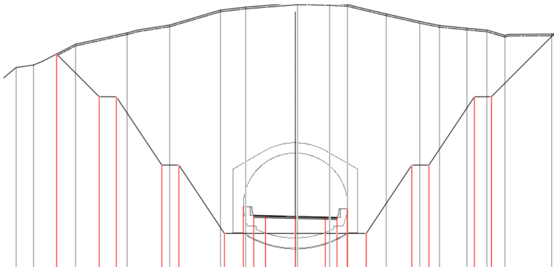
Figura 11 – Sezione trasversale di scavo GA
