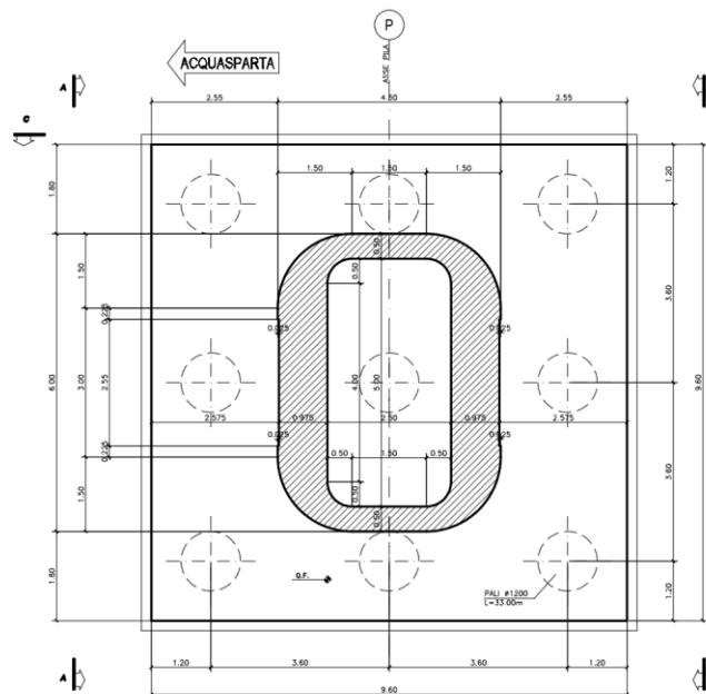
Figura 17: Sezione pila doppia
