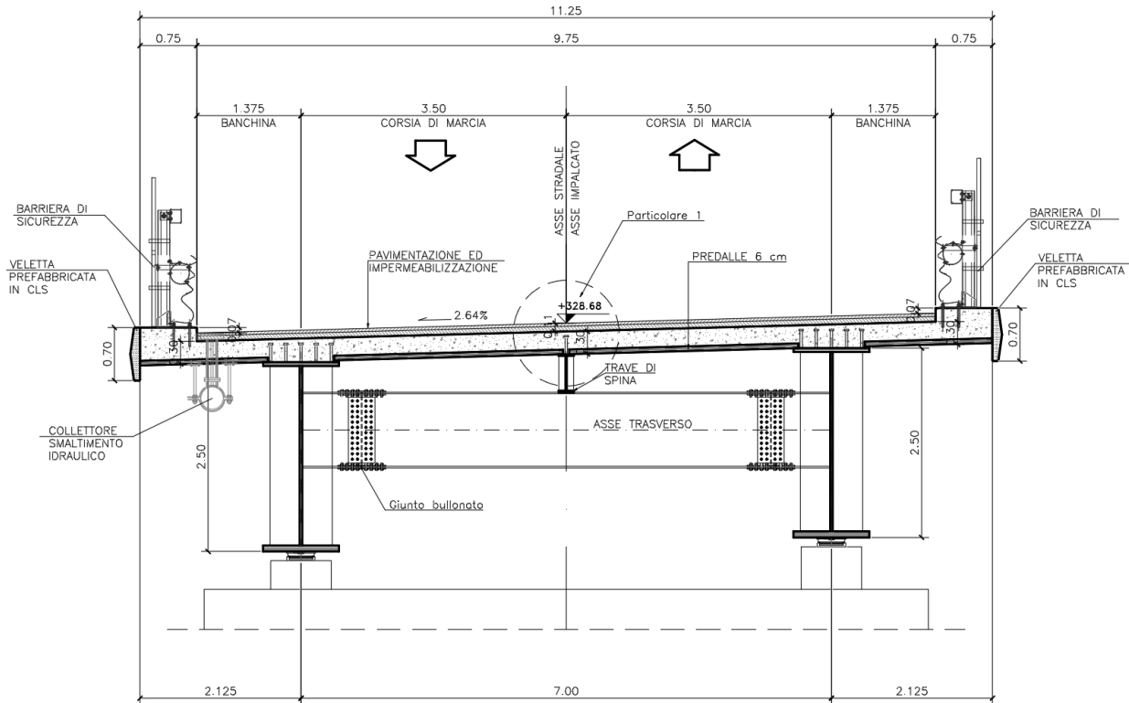
Figura 15 - Sezione Trasversale dell'impalcato del Viadotto Marroggia 1.
