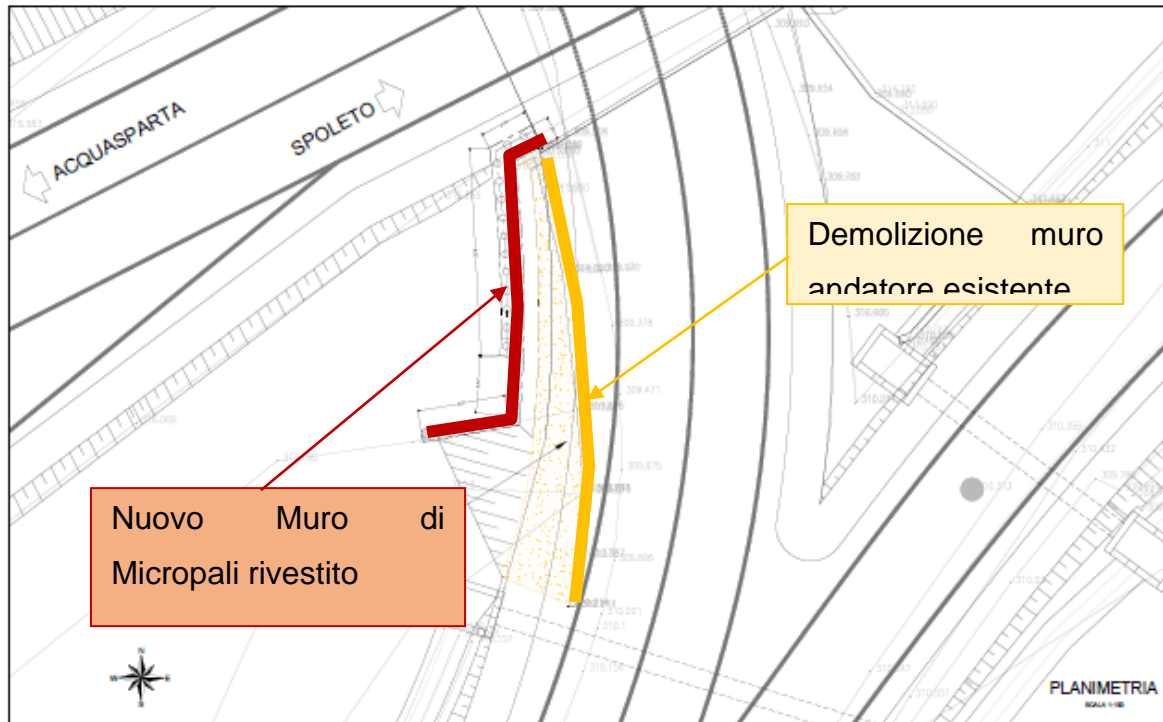
Figura 20 - Stralcio Planimetrico dello Svincolo di Baiano con l'evidenza della porzione del muro da demolire e del nuovo da costruire.
