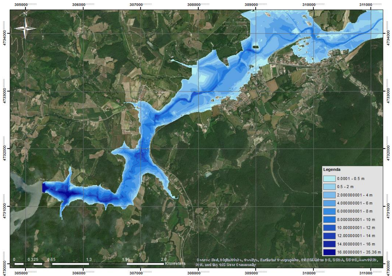
Figura 26. Tiranti massimi asincroni Ante operam -Configurazione a)
