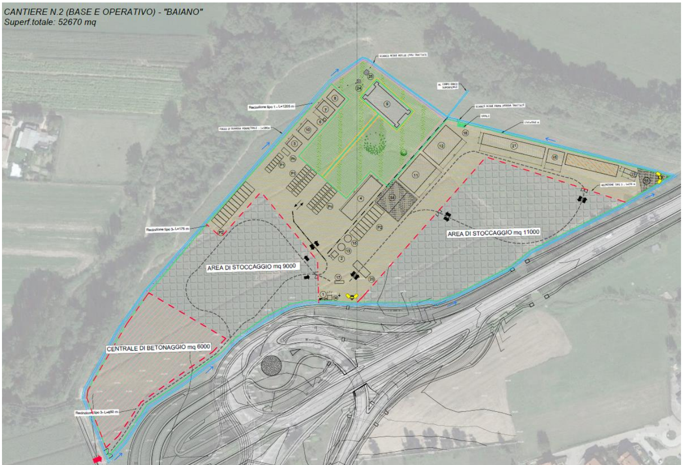
Figura 39 - Layout del cantiere 2 (Base e Operativo) in ambito Svincolo di Baiano.
