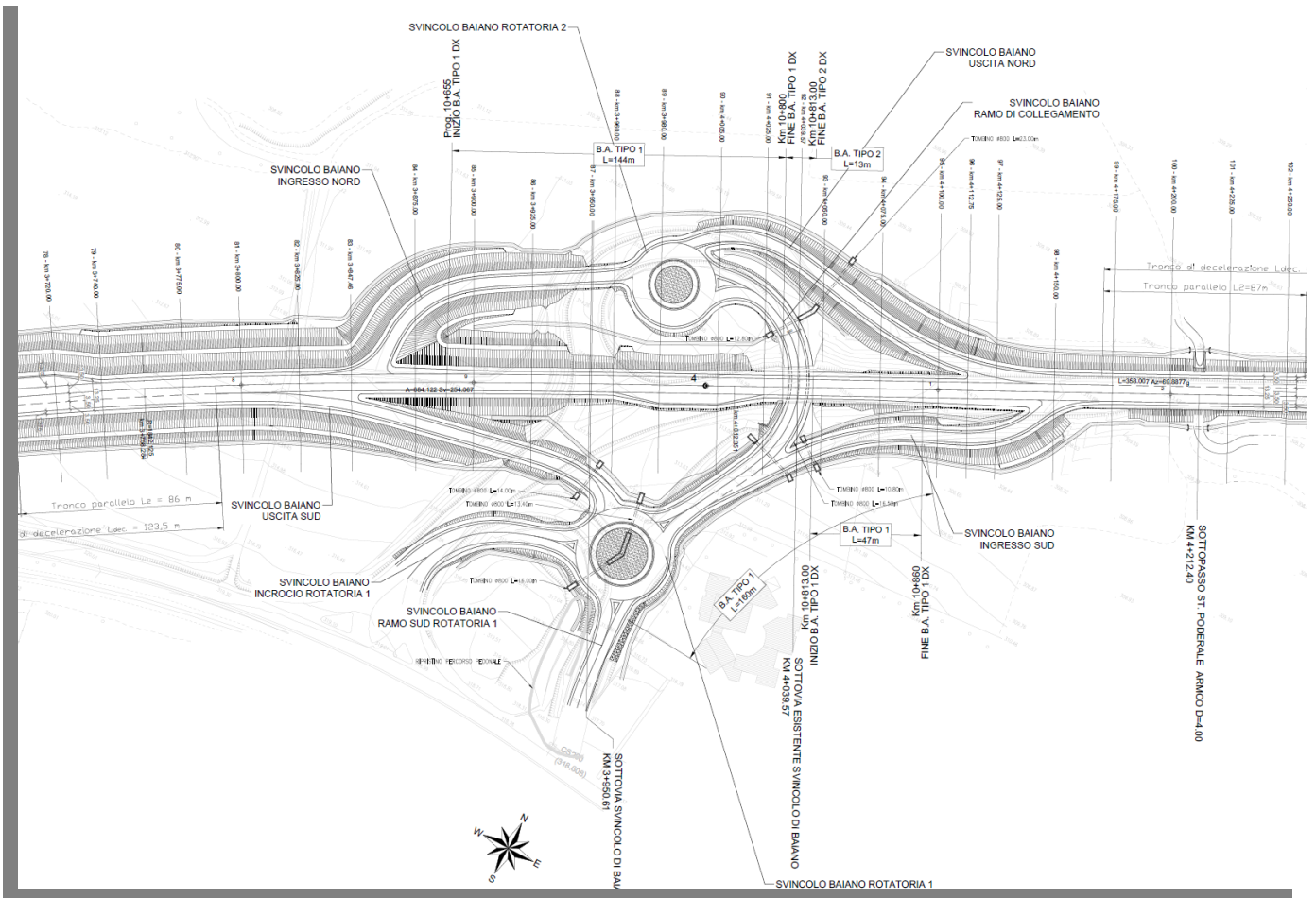
Figura 10 - Configurazione di progetto dello Svincolo di Baiano.
