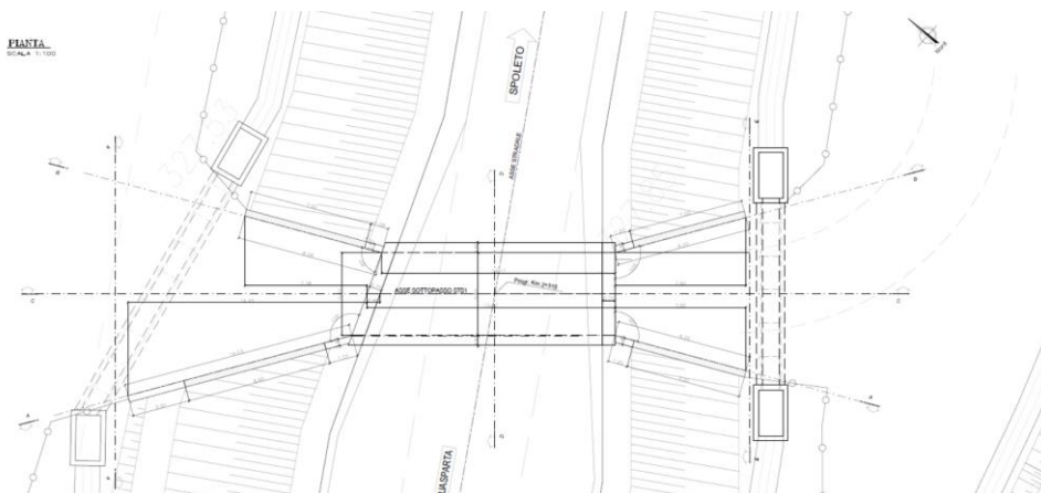
Figura 21 - Stralcio planimetrico Sottopasso Km 2+315.00.
