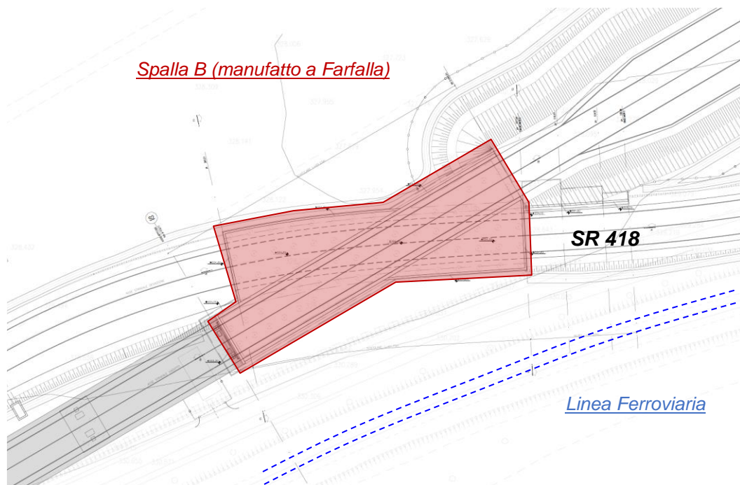
Figura 18 - Planimetria della Spalla B del Viadotto Marroggia.
