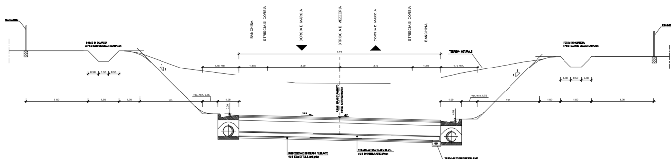
Figura 6 - Sezione Tipo in trincea.
