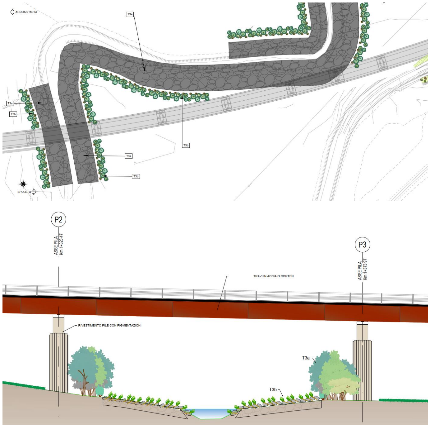
Figura 36 - Stralcio planimetrico e sezione di alcuni degli interventi di mitigazione ambientale e paesaggistica in ambito Torrente Marroggia.
