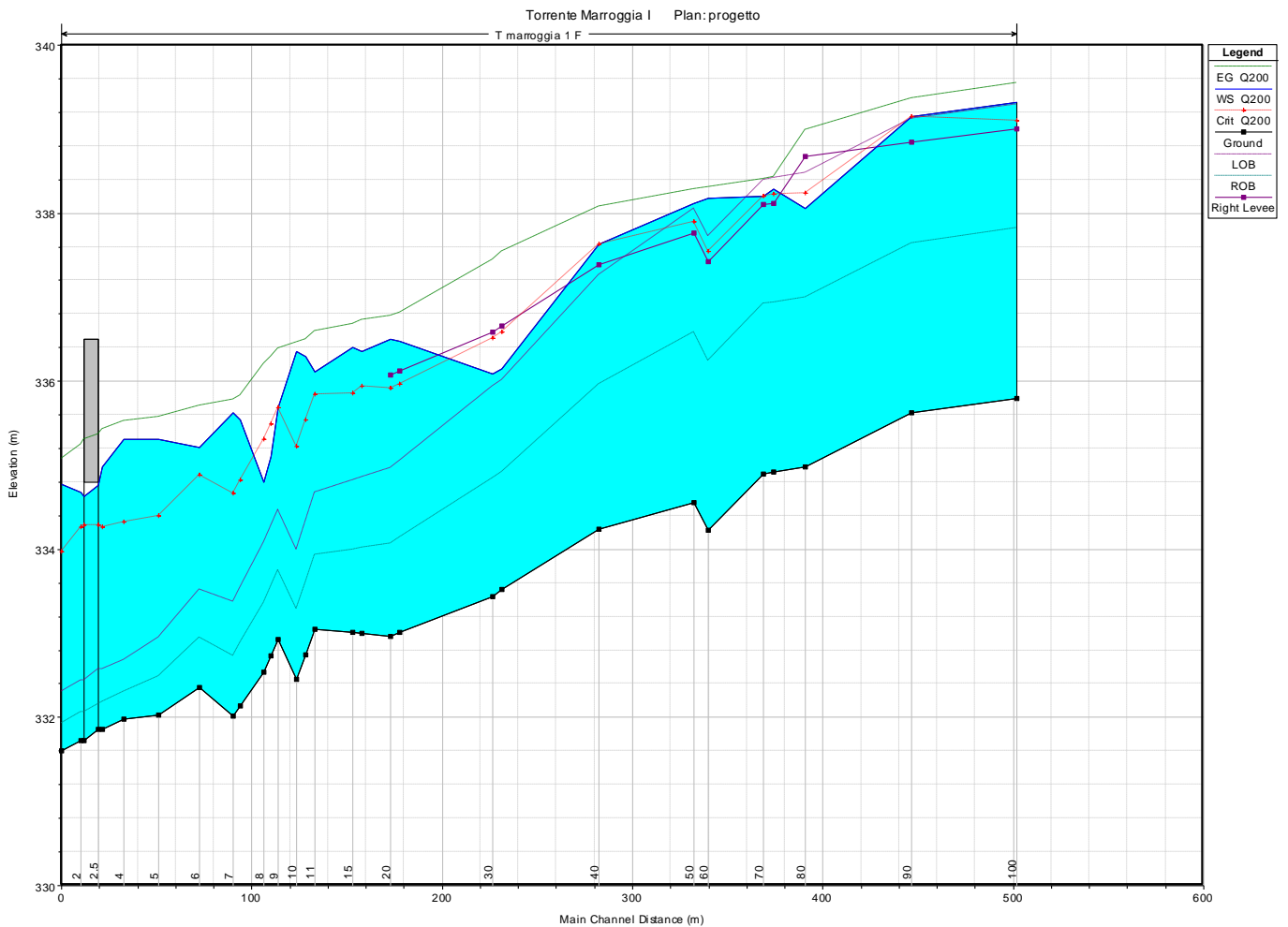
Figura 30 - Profilo della piena duecentennale Q200 = 110 m 3 /s – Stato di Progetto.
