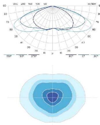
CURVA FOTOMETRICA
