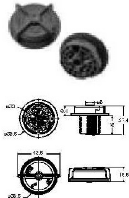
Dispositivo punto-punto
