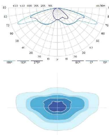
CURVA FOTOMETRICA
