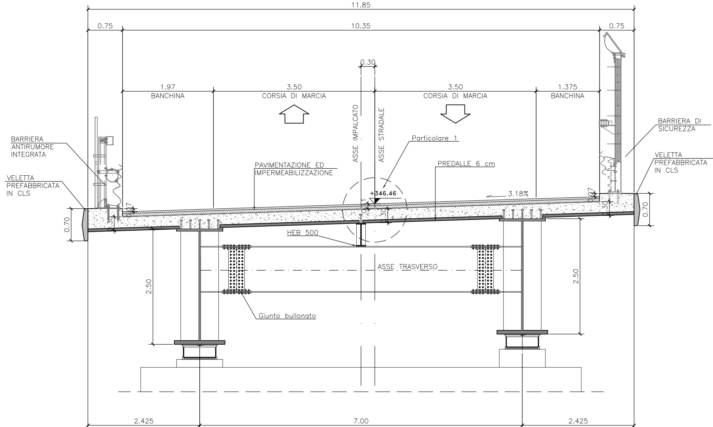
SEZIONE TRASVERSALE PILA 10 SCALA 1:50
