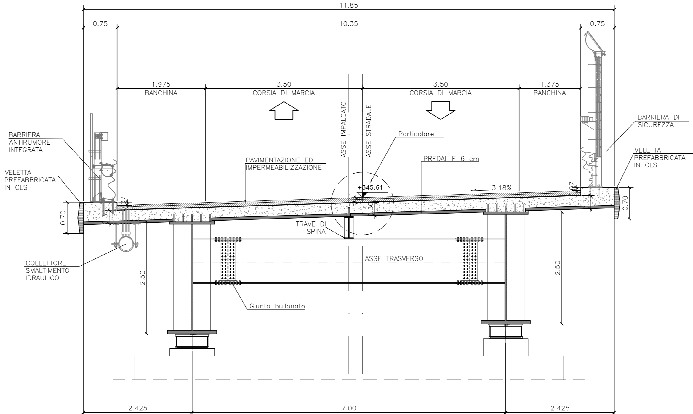
SEZIONE TRASVERSALE PILA 11 SCALA 1:50
