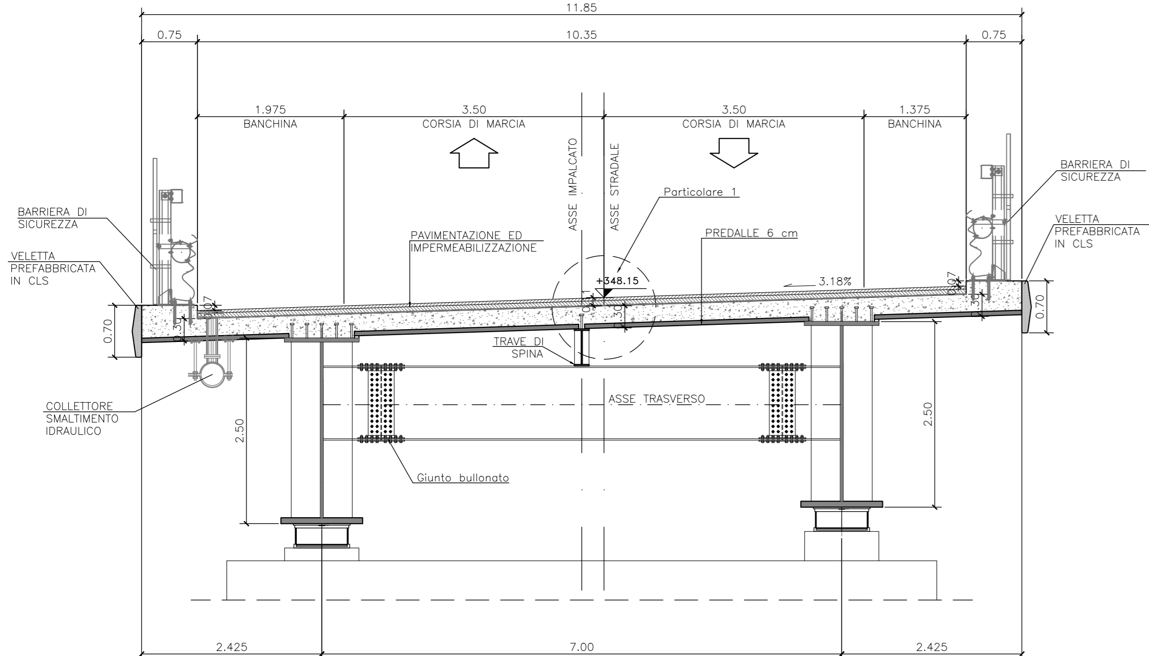
SEZIONE TRASVERSALE PILA 10 SCALA 1:50
