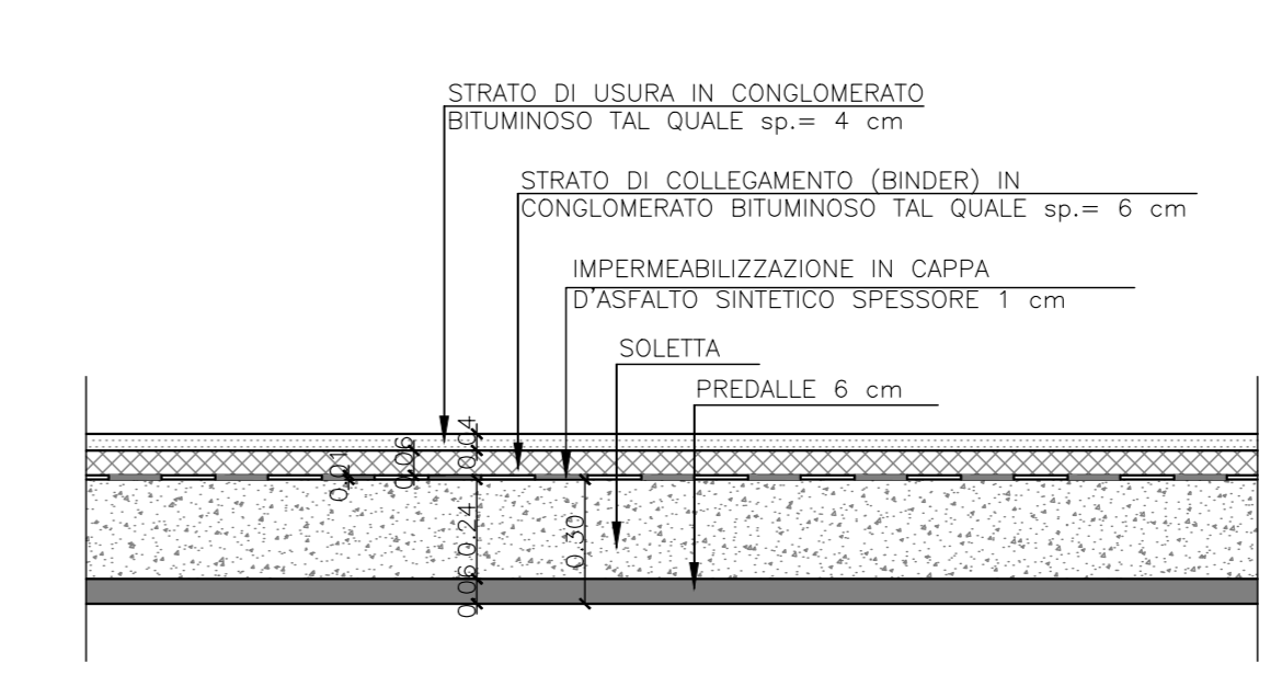
PARTICOLARE 1 SCALA 1:20
