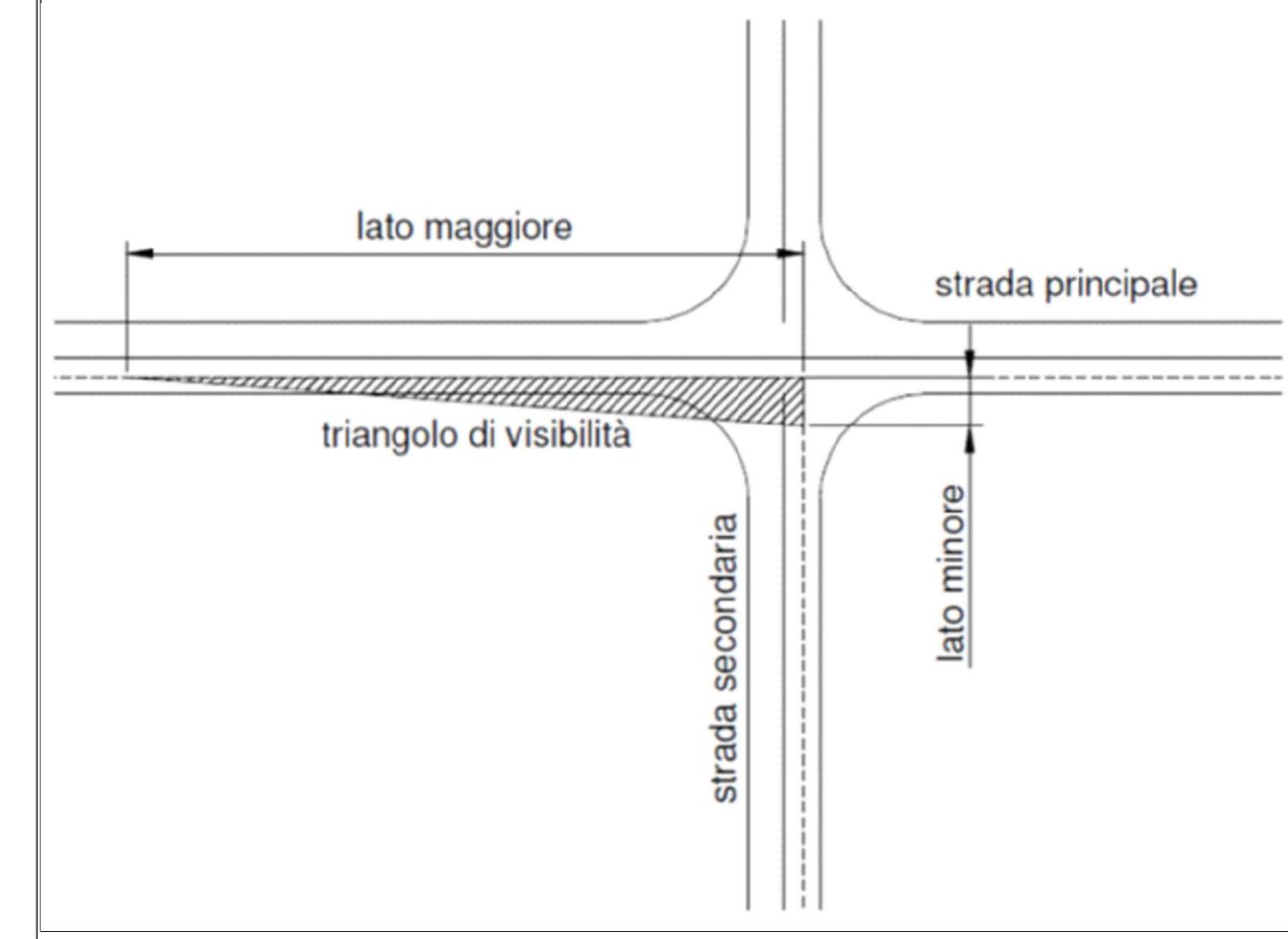
CAMPO DI VISIBILITÀ INTERSEZIONE A T Schema
