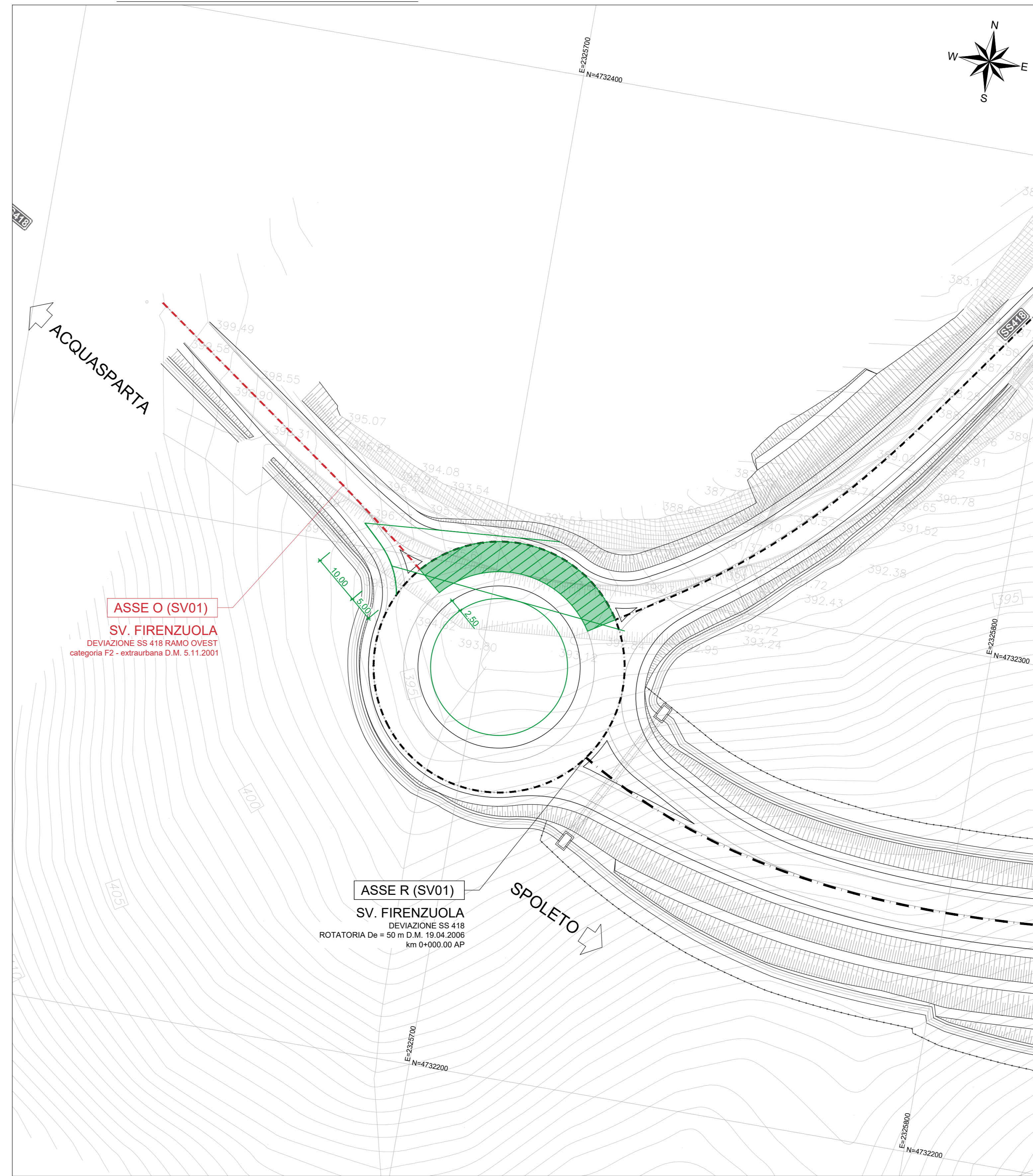
SV01 asse AP - CAMPI DI VISIBILITÀ IN ROTATORIA (asse R)
