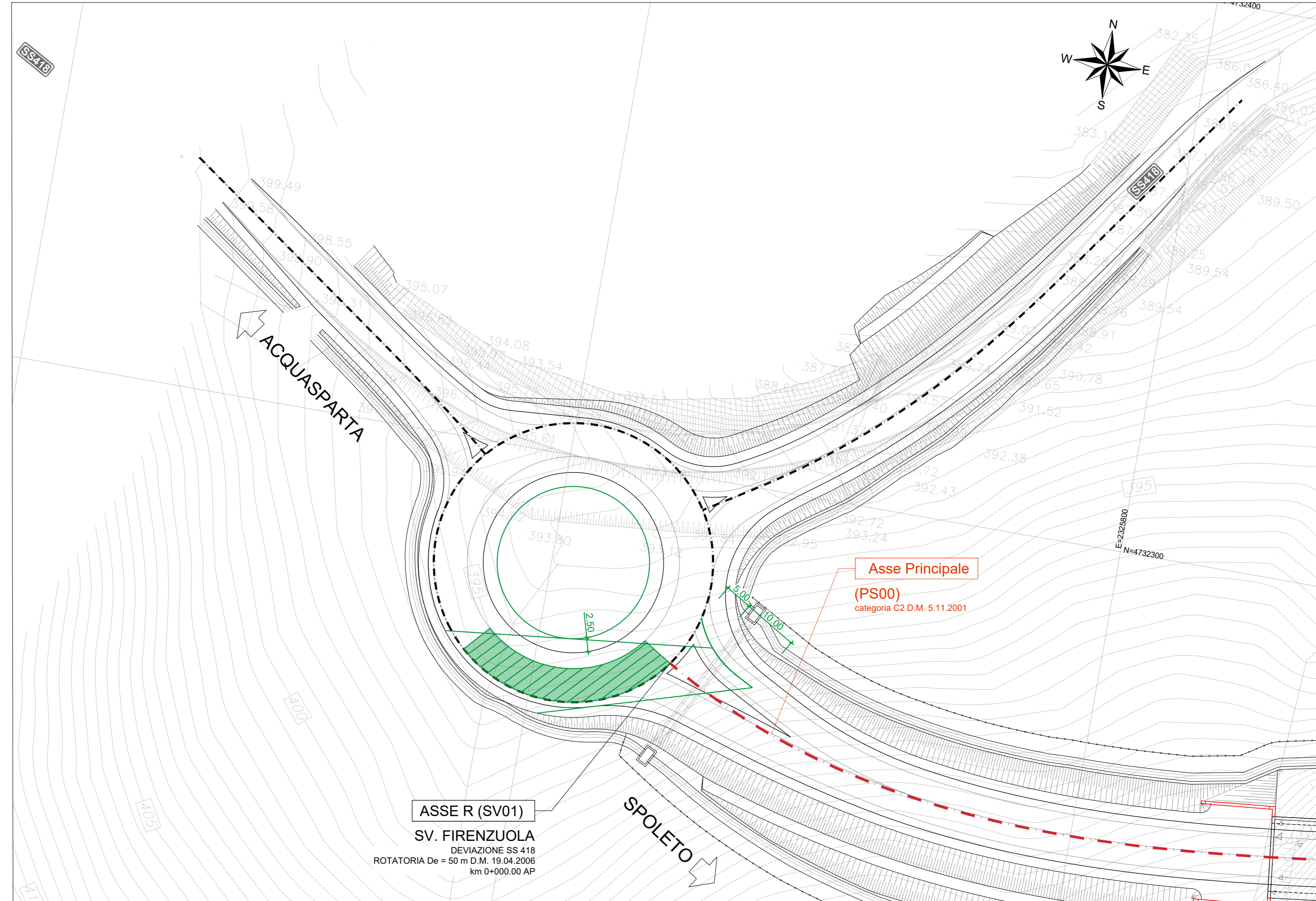
SV01 asse AP - CAMPI DI VISIBILITÀ IN ROTATORIA (asse R)
