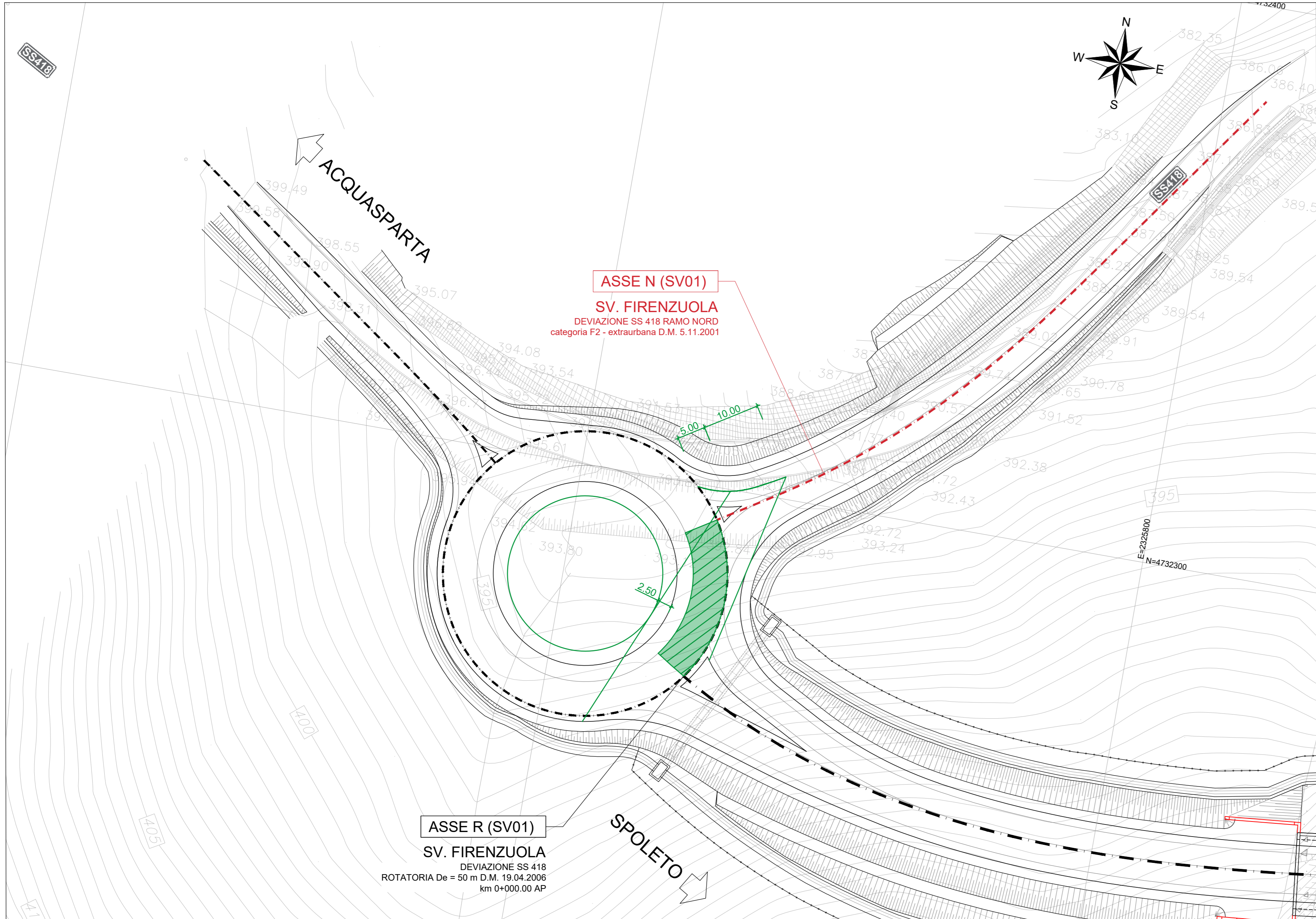
SV01 asse N - CAMPI DI VISIBILITÀ IN ROTATORIA (asse R)
