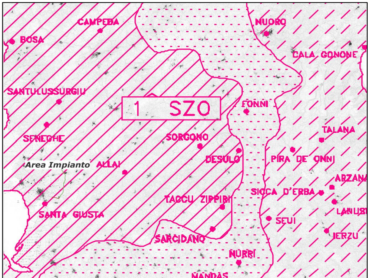
CARTA DELLE ISOIETE - REGIONE SARDEGNA- PIOGGIA INDICE 50 mm
