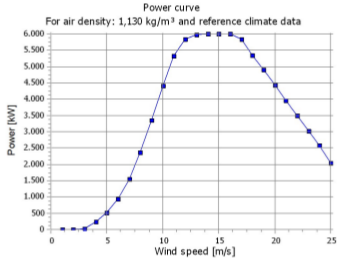
Figura 7: Grafico delle Curve di Potenza dell'aerogeneratore alla densità dell'aria pari a 1,130 \text{ kg/m}^3
