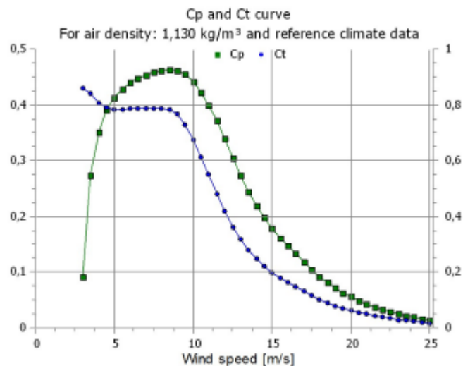
Figura 8: Grafico relativo alla Curva di Potenza ed alla Curva di Spinta dell'aerogeneratore alla densità dell'aria pari a 1,130 \text{ kg/m}^3
