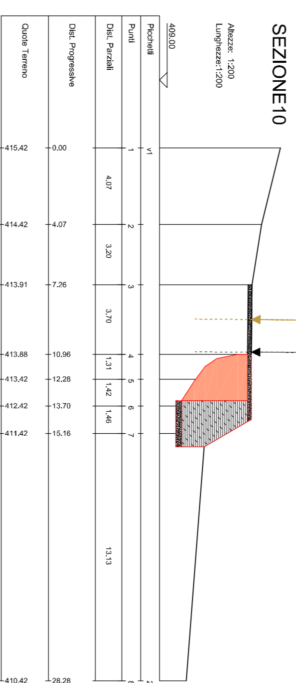
SEZIONE - RIPIIMENTO E SCOGLIERA SCALA 1:200
