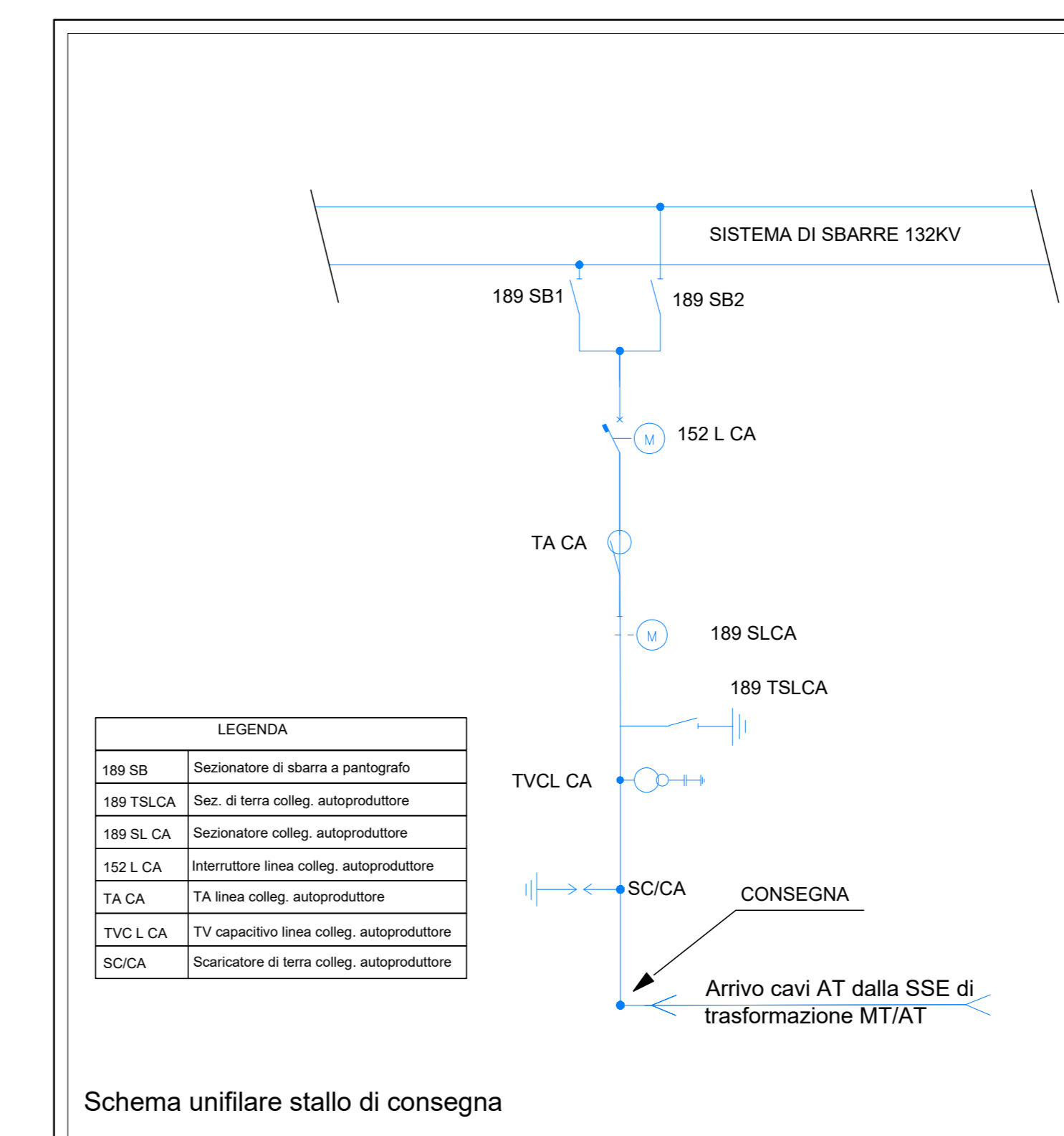
SCHEMA UNIFILARE STALLO IN PROGETTO
