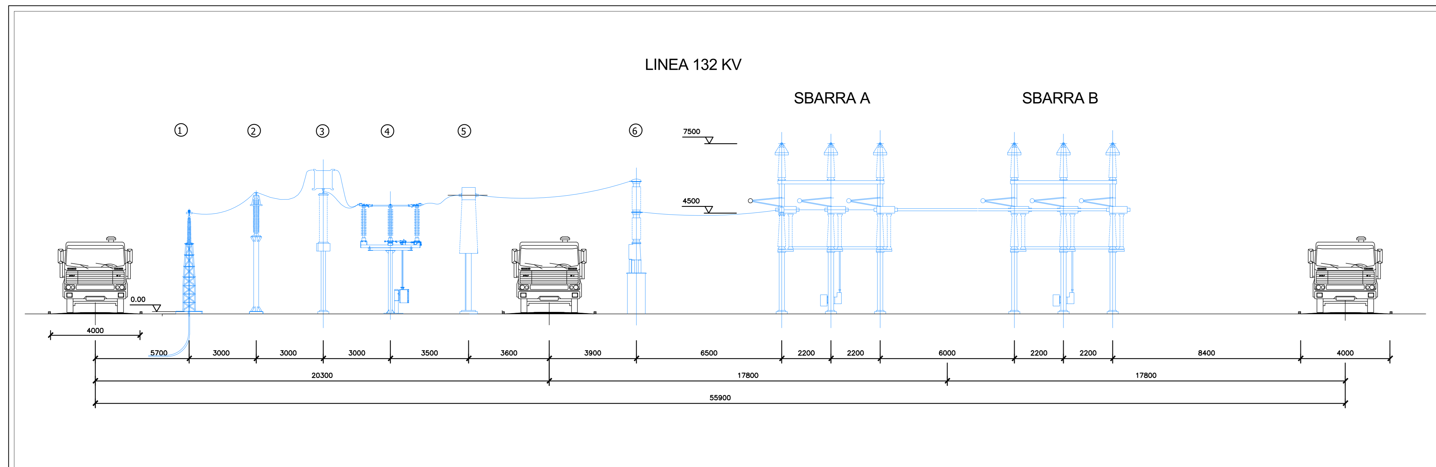
PROSPETTO-SEZIONE STALLO
