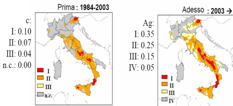
Figura 3.2 -Classificazione (zonazione) sismica della Sicilia secondo l'Ordinanza 3274/03
