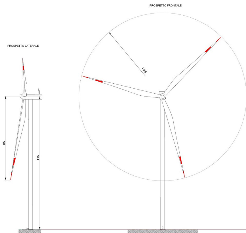
Figura c-1: Struttura aerogeneratore
