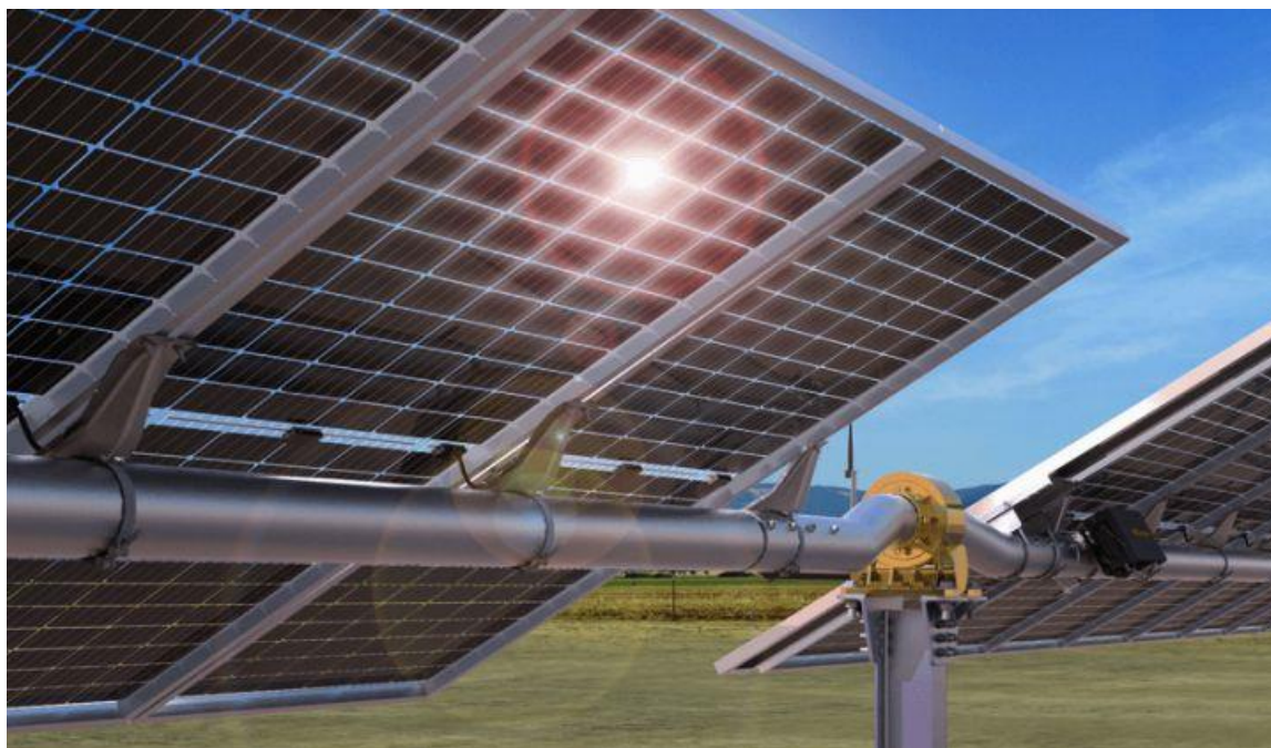
Figura 6 - Particolare strutturale
