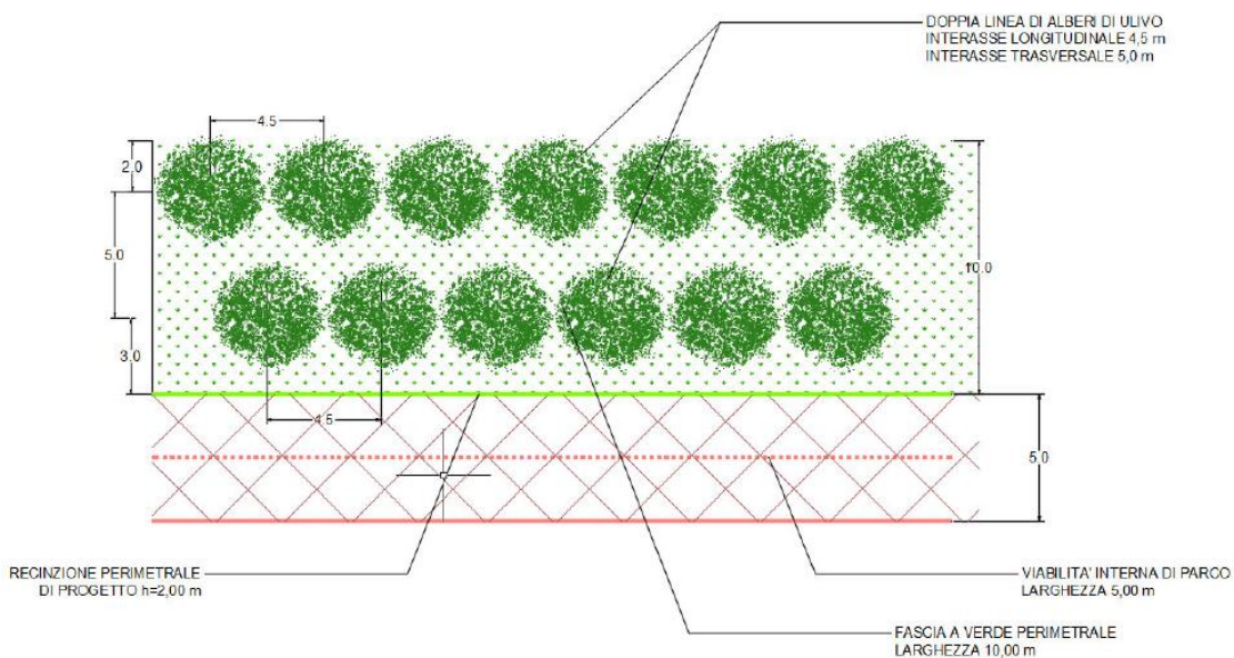
Figura 10 – Caratteristiche doppia filare sfalsato
