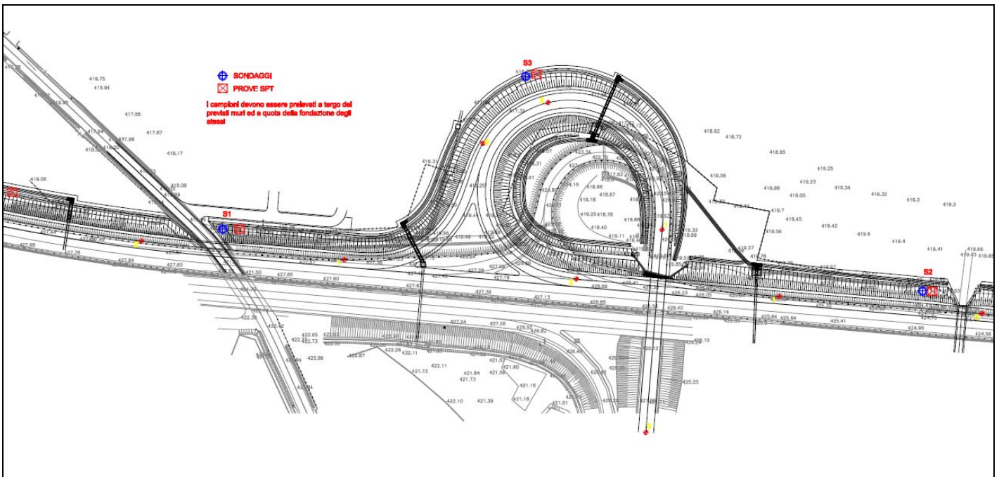
Fig. 6 – Planimetria con ubicazione dei sondaggi geognostici e delle prove STP
