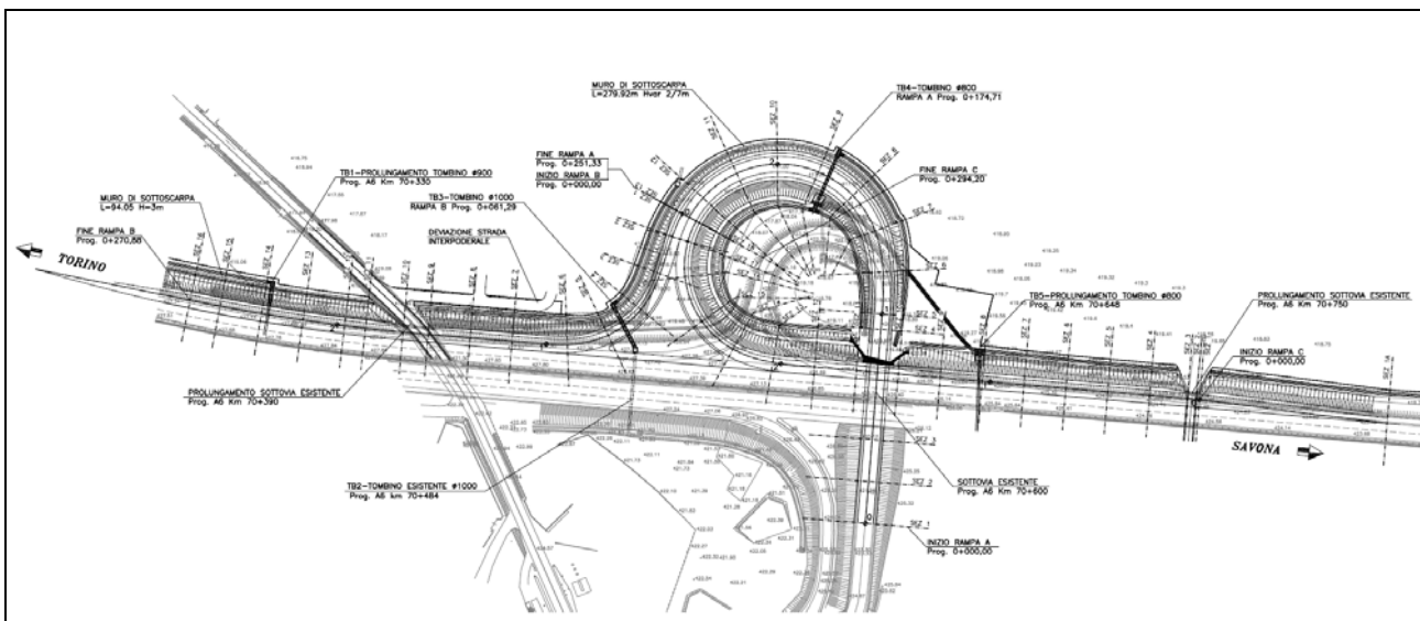
Fig. 2: Planimetria di progetto
