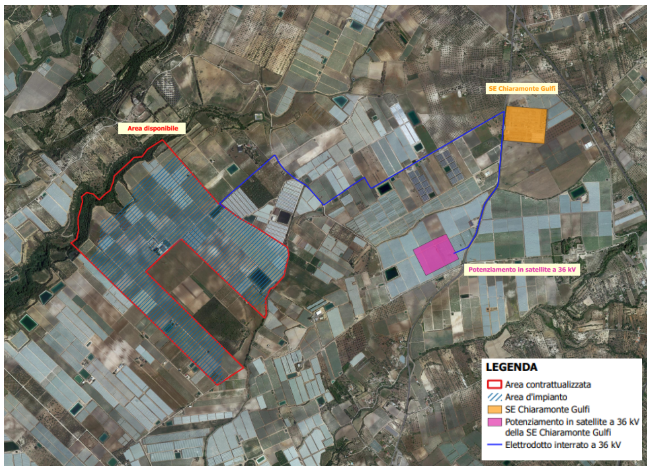
Figura 3 – Sistema agrivoltaico su ortofoto
