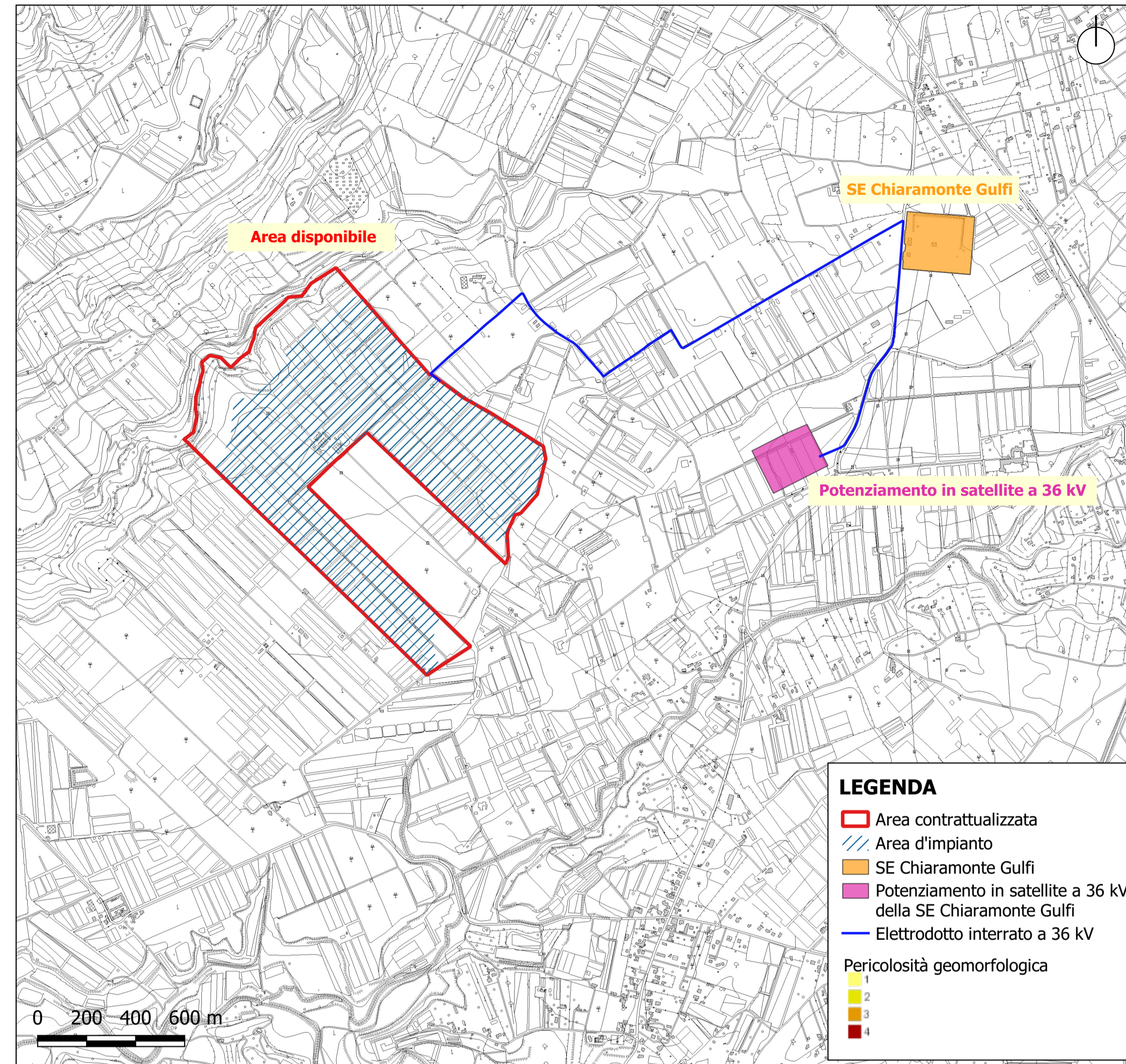
Carta della Pericolosità Geomorfologica - Livelli di Pericolosità - Bac 78 - Fiume Acate Dirillo - Scala 1:15.000
