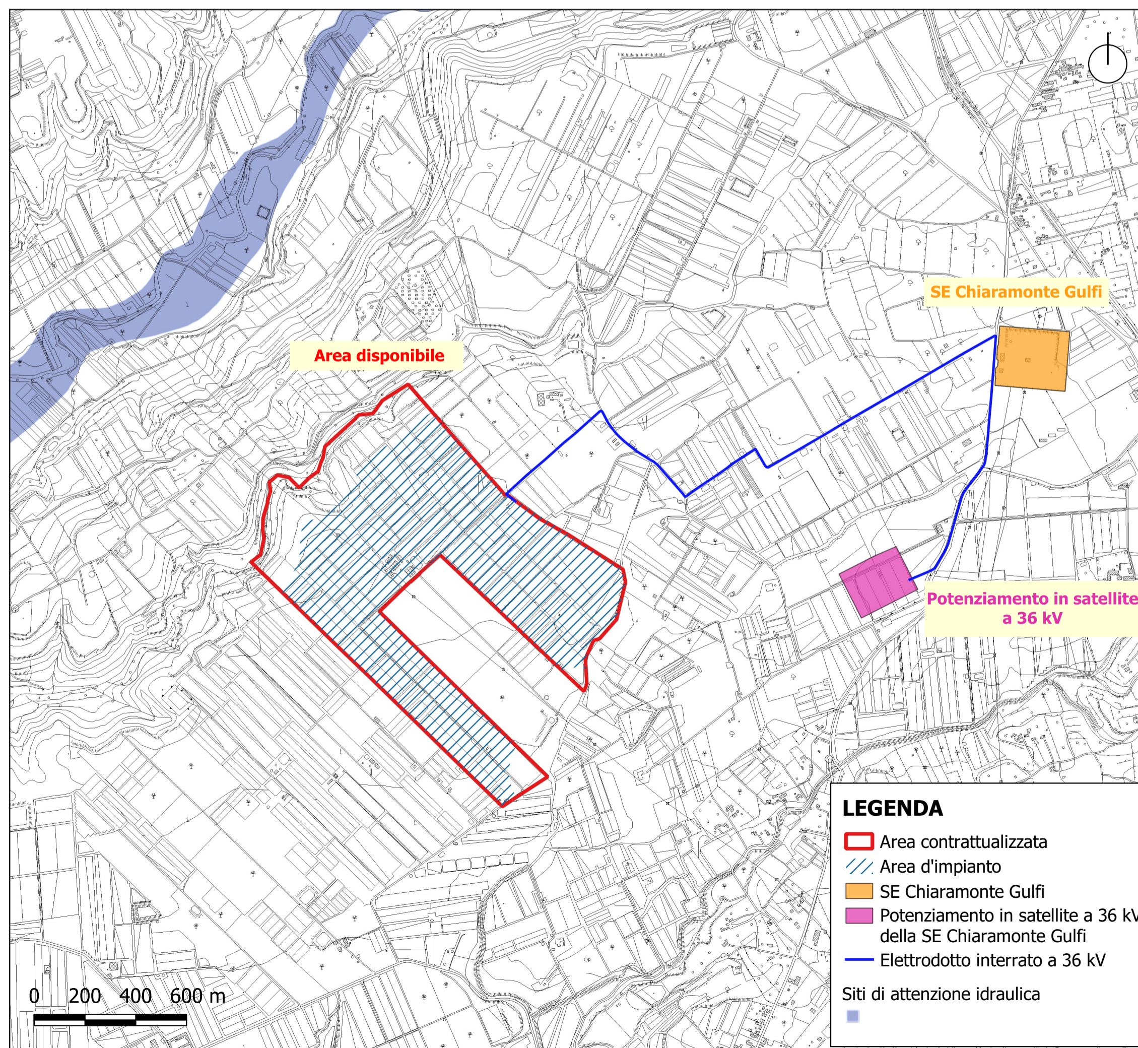
Siti di attenzione - Bac 078 - Fiume Acate Dirillo - Scala 1:15.000
