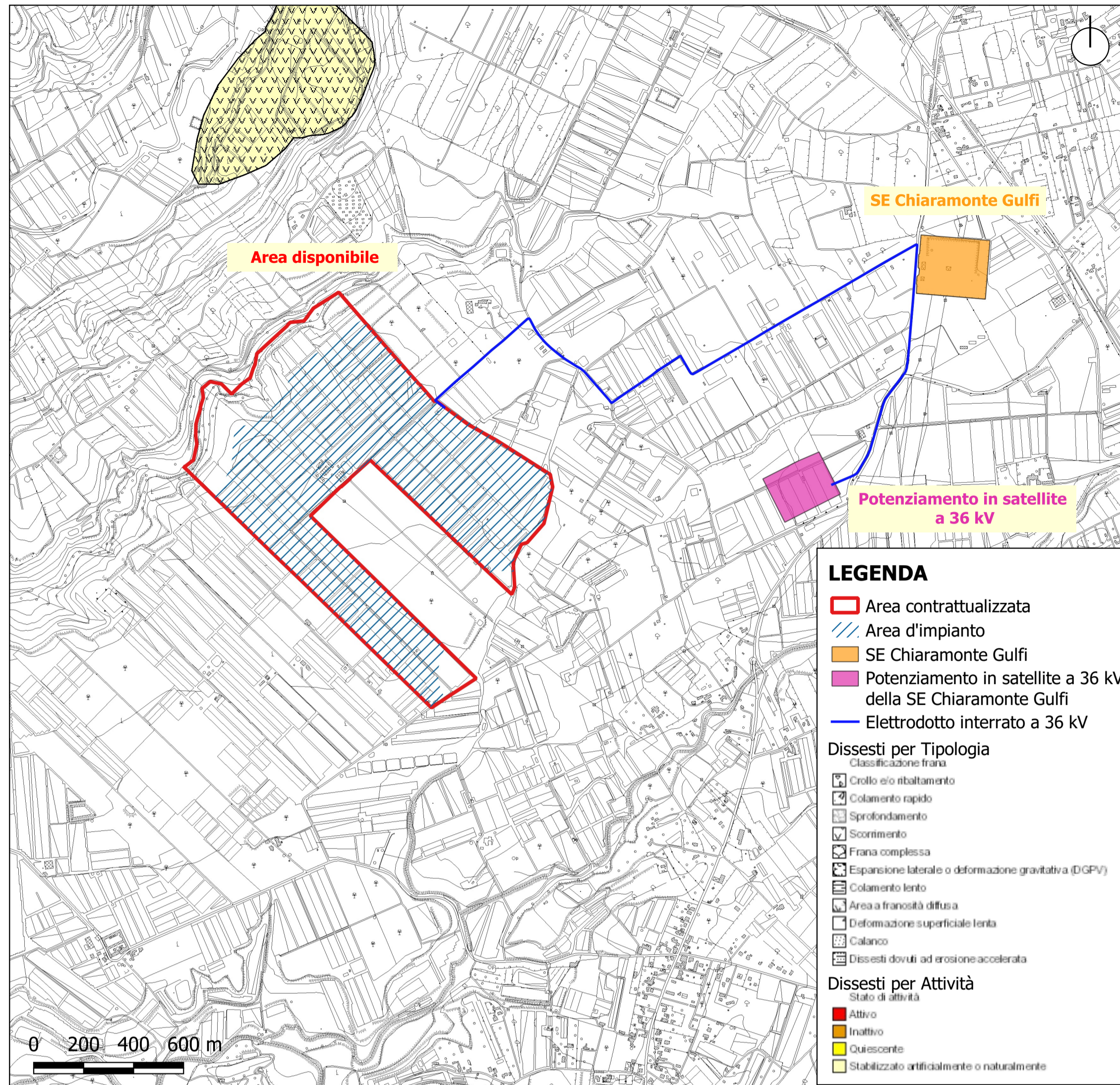
Carta dei Dissesti e Stato di Attività - Bac 078 - Fiume Acate Dirillo - Scala 1:15.000
