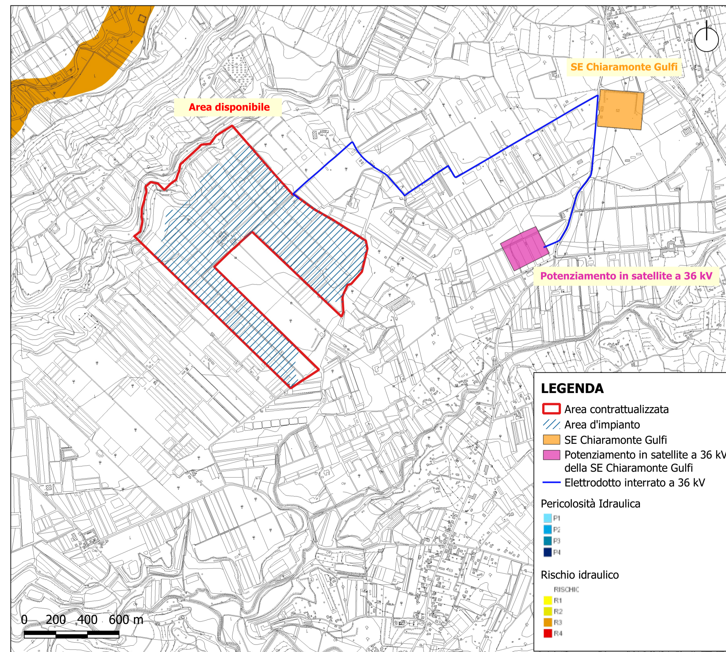
Carta della Pericolosità e del Rischio Idraulico - Bac 078 - Fiume Acate Dirillo - Scala 1:15.000
