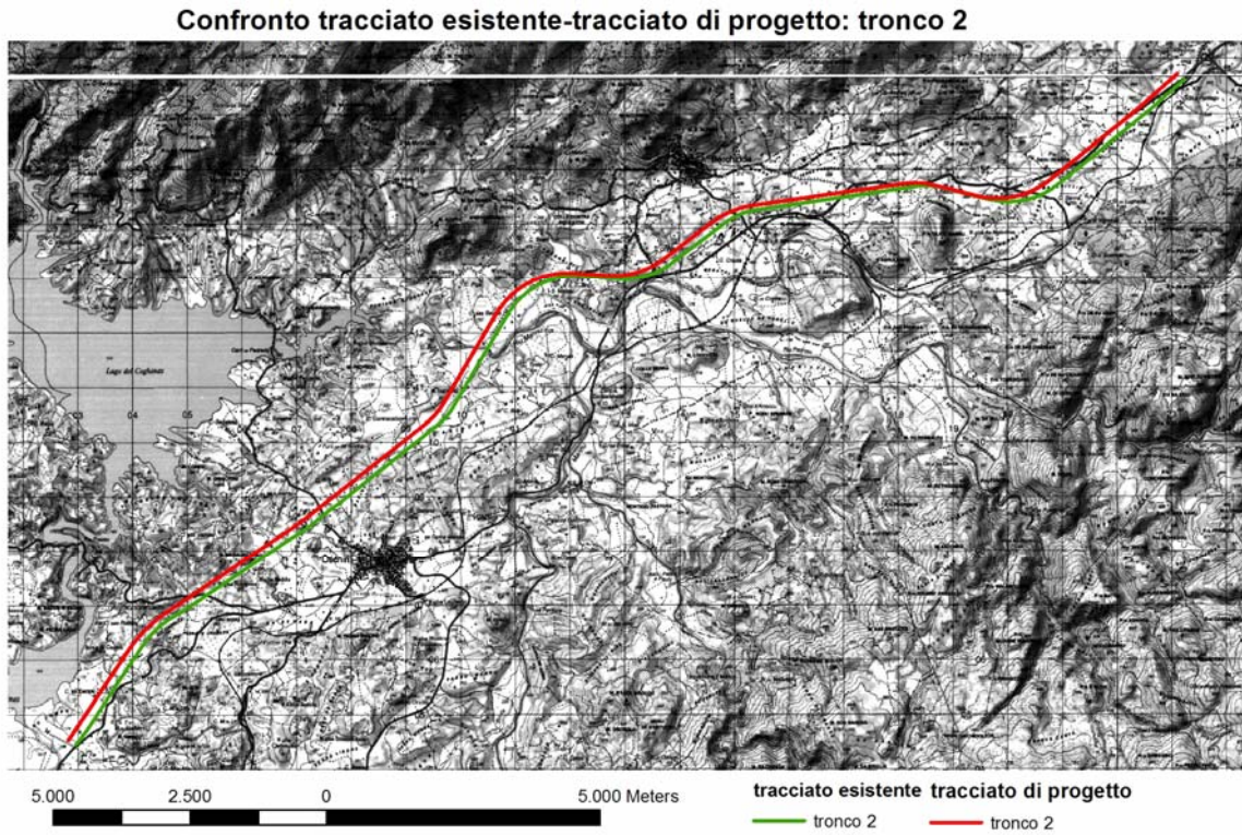
Figura 5 confronto tracciato esistente e di progetto- TRONCO II
