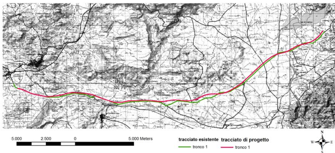
Confronto tracciato esistente-tracciato di progetto: tronco 1
