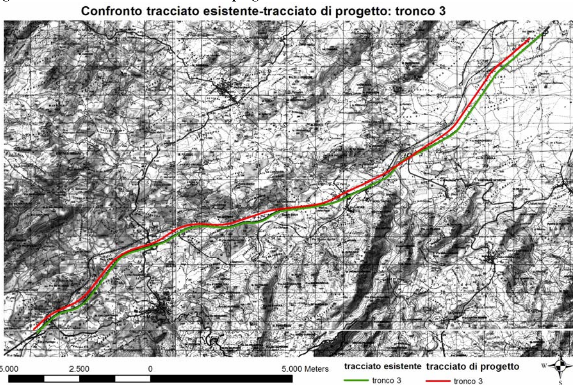
Figura 6 confronto tracciato esistente e di progetto- TRONCO III
