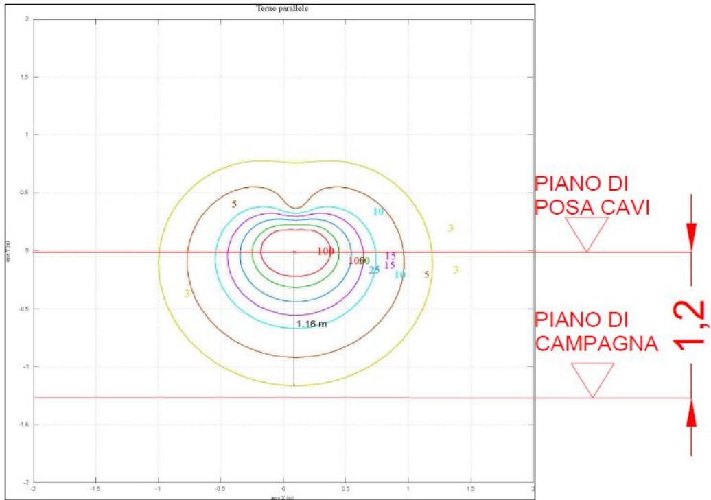
FIGURA 2: CAVIDOTTO AT INTERNO AL CAMPO - CURVE ISOINDUZIONE – 2 LINEE AT INTERRATE
