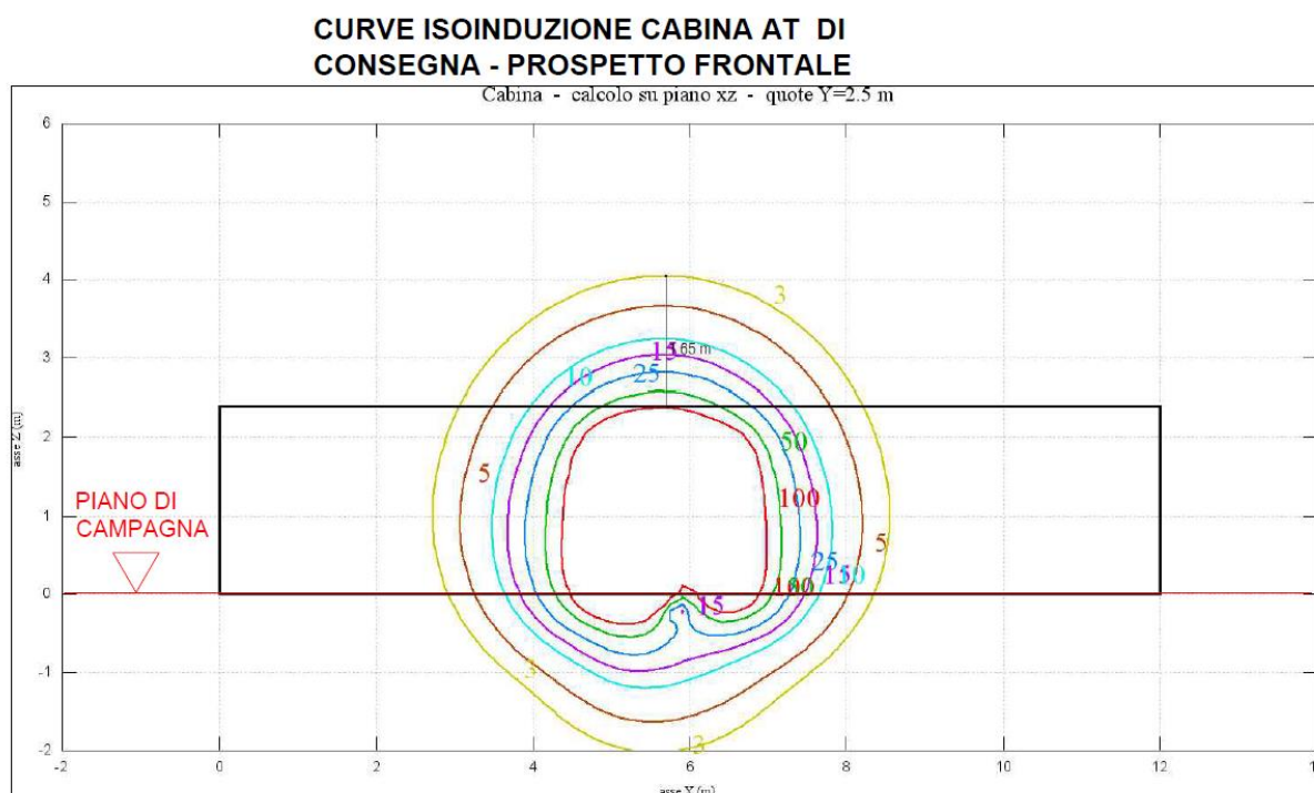
FIGURA 6: CURVE ISOINDUZIONE CABINA AT DI CONSEGNA (PROSPETTO FRONTALE)
