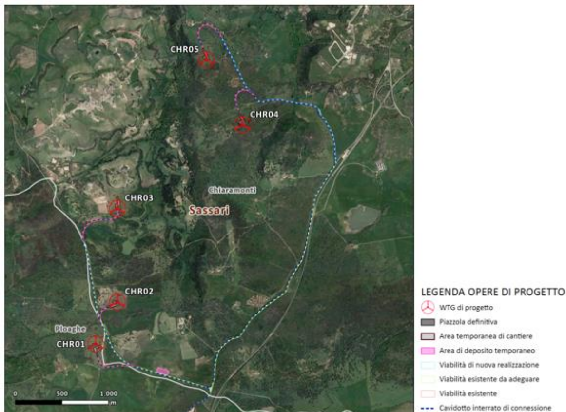
Figura 2.3: Inquadramento della viabilità di progetto interna al campo
