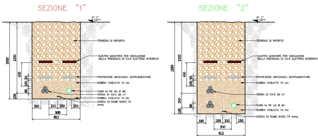
Figura 2.11 – Sezioni tipo posa cavidotti
