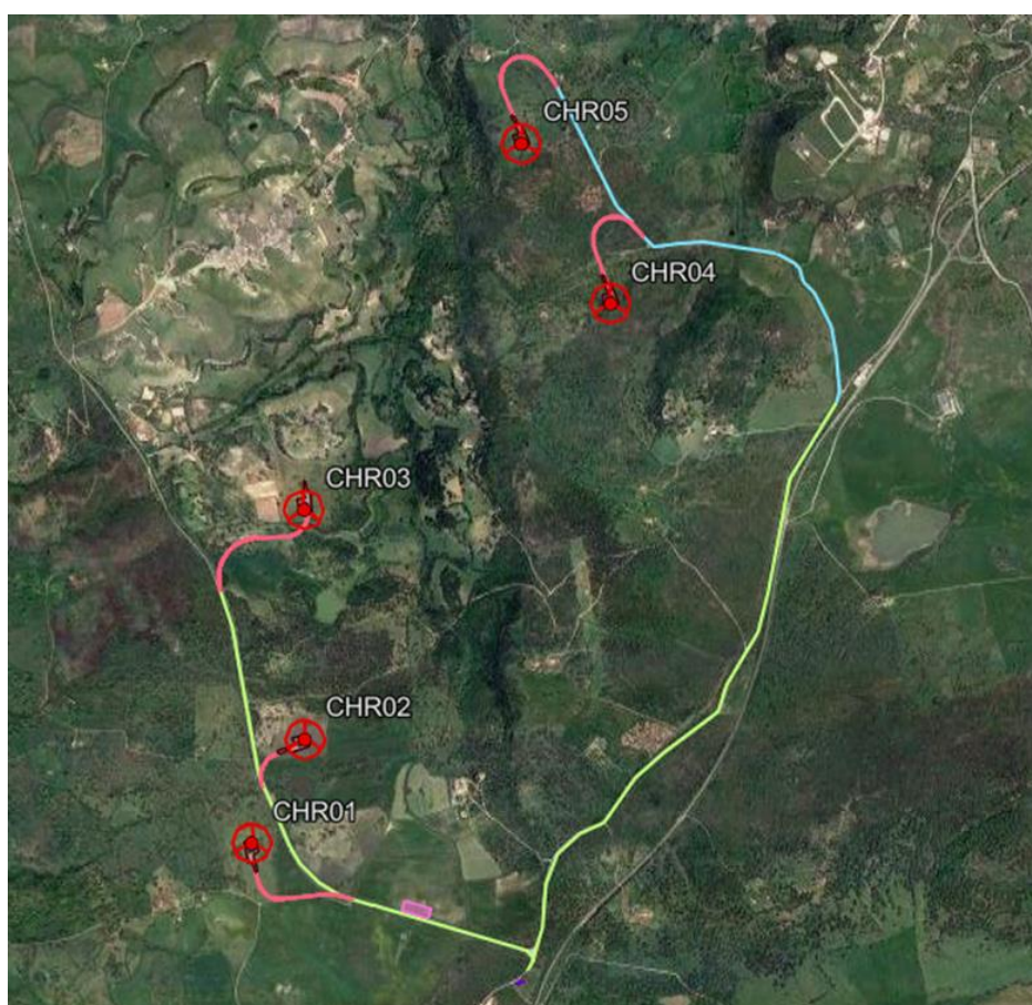
Figura 2.9: viabilità interna al sito
