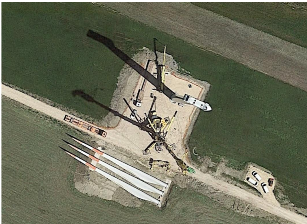
Figura 2.5 – esempio di piazzola in fase di costruzione
