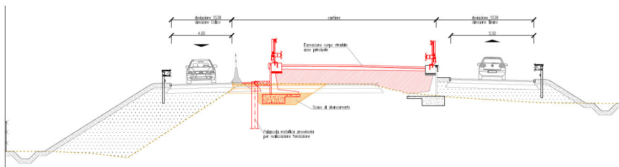
Figura 26 - Sezione A-A
