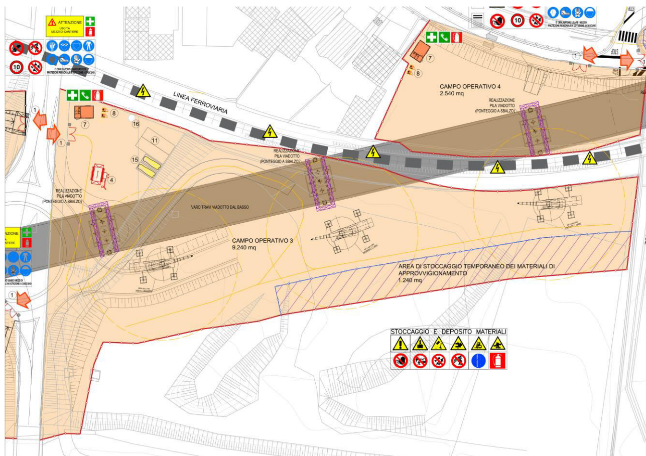
Figura 12 - Layout campo operativo n. 3
