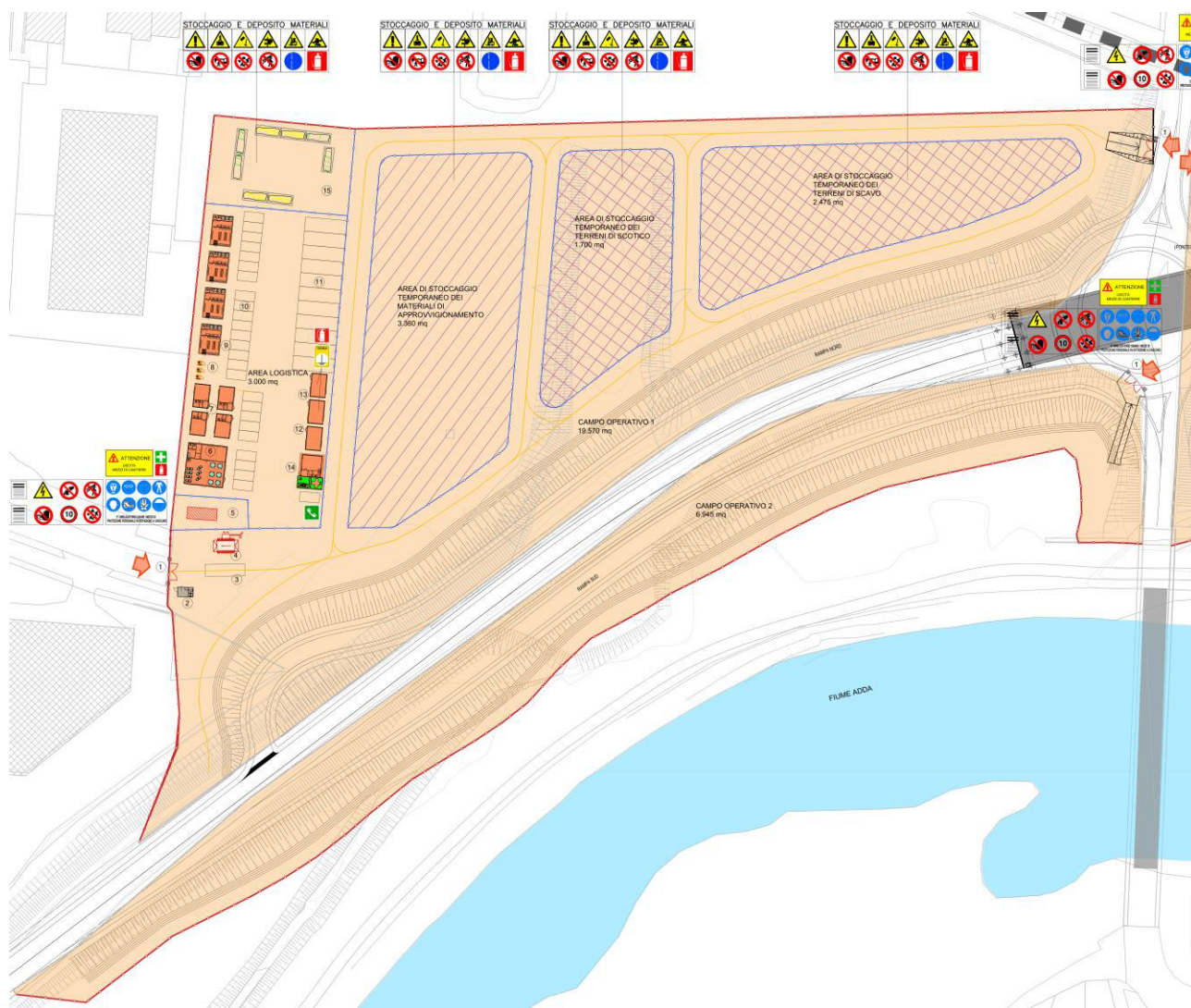
Figura 9 - Layout campo base e campi operativi 1 e 2
