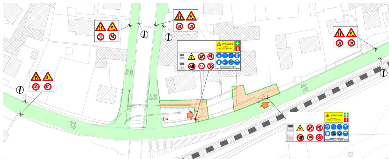
Figura 23 - Rettifica accessi e confini interessati dal bypass
