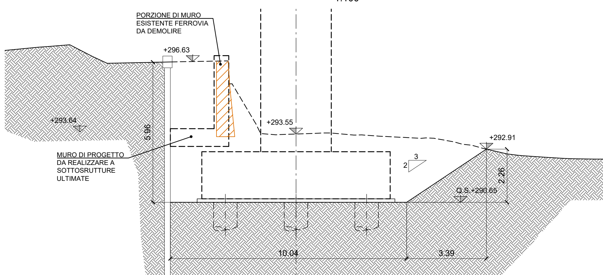
SEZIONE PILA 3
