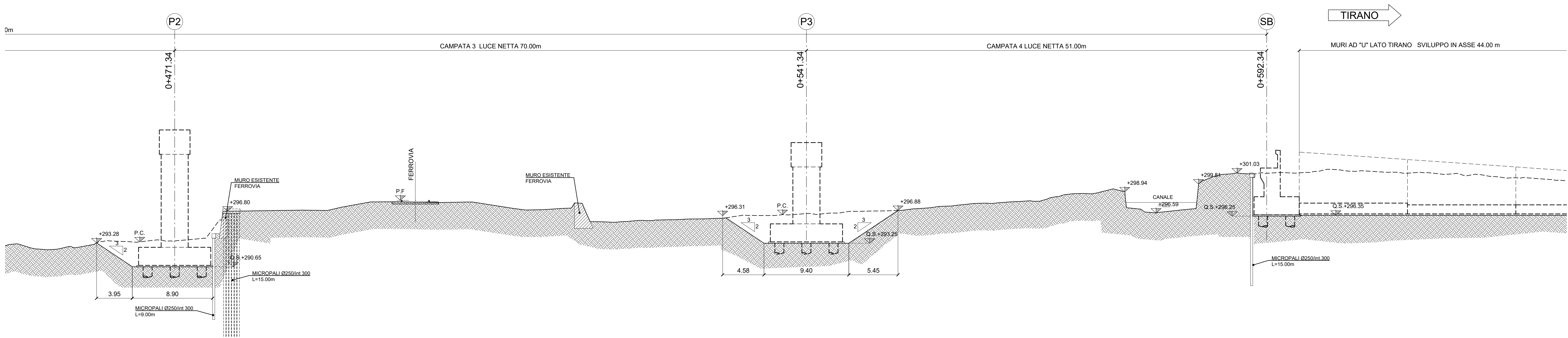
SEZIONE LONGITUDINALE DA SPA A P2 SCALA 1:200
