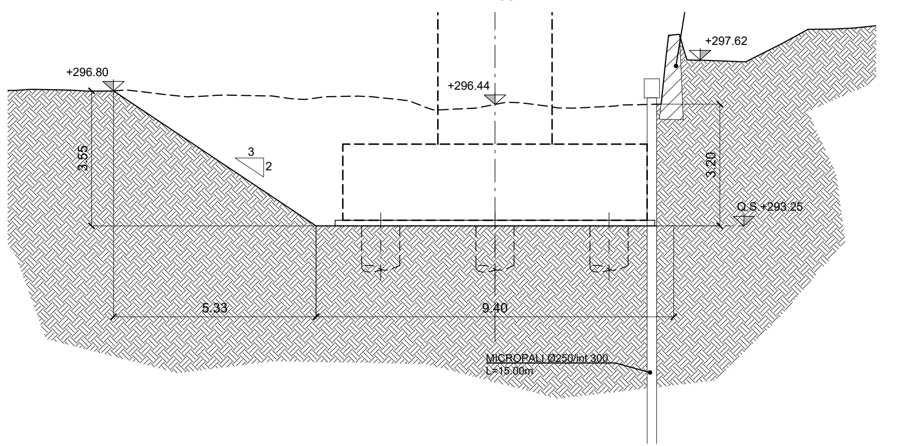
SEZIONE PILA 3
