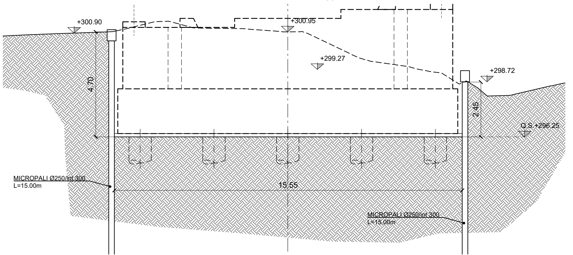
SEZIONE PILA 2
