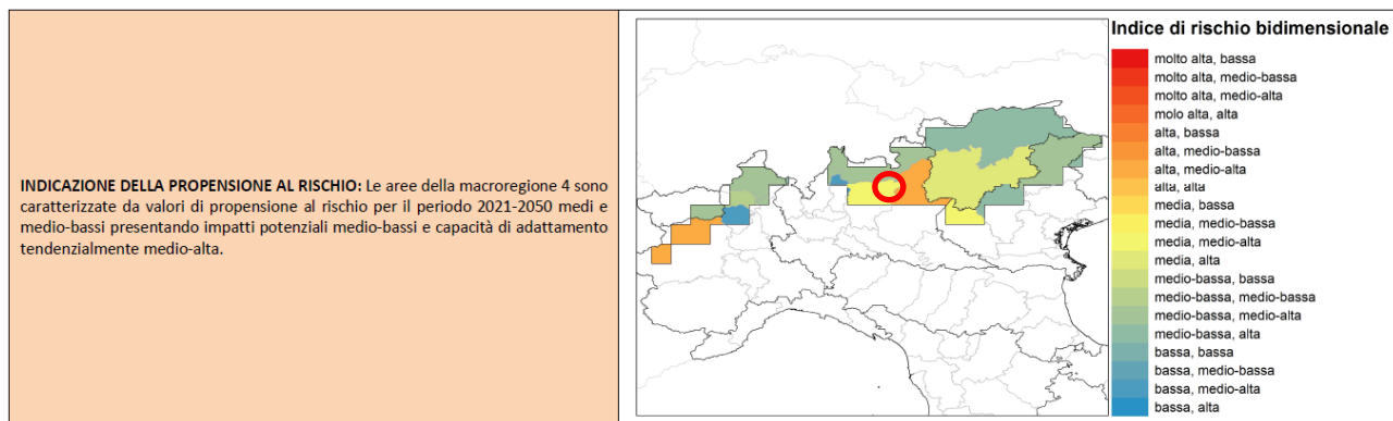
Figura 23 - Indice di rischio per la macroregione 2: Prealpi e Appennino Settentrionale. Pianura Padana, alto versante adriatico e aree costiere dell'Italia centro-meridionale. Cerchiata in blu l'area di intervento.
