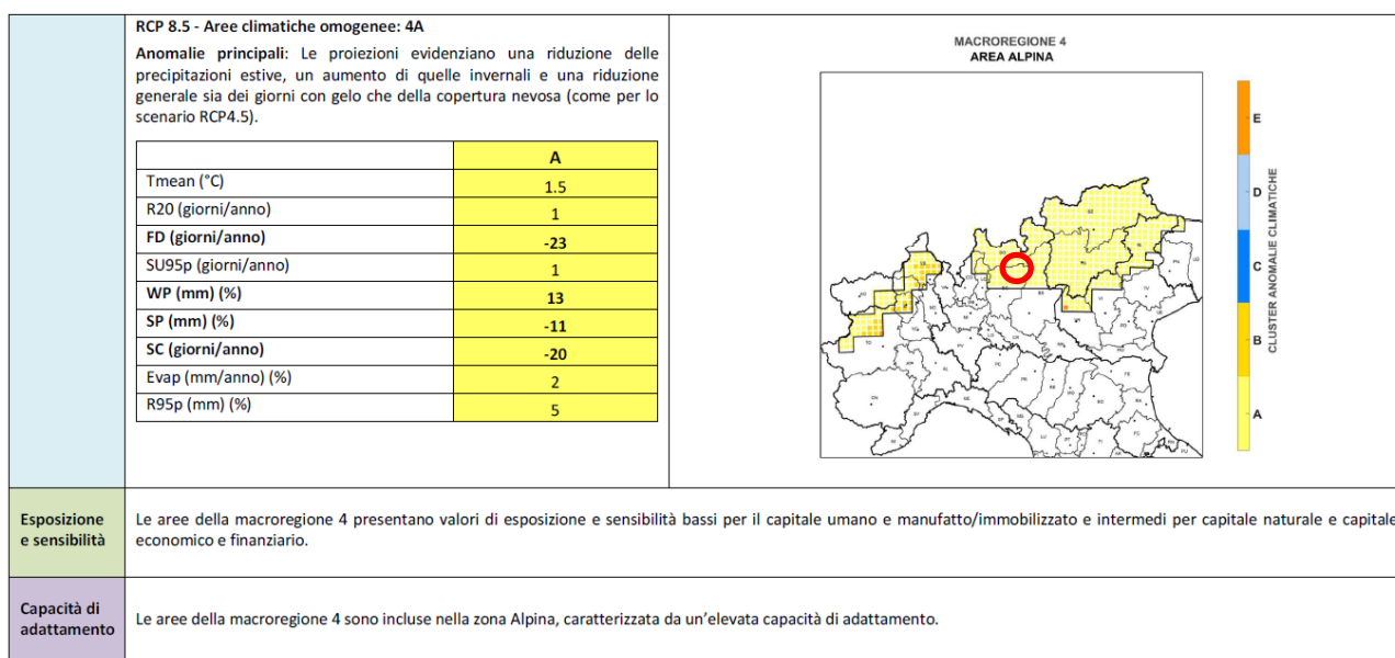
Figura 22 - Macroregione 4: Area alpina nello scenario RCP 8.5. Cerchiata in rosso l'area di intervento.
