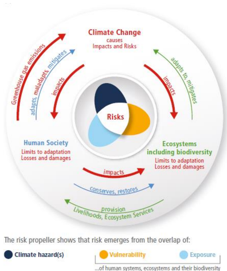
Figura 15 Schema concettuale del processo per la resilienza climatica e l'adattamento ai cambiamenti climatici
