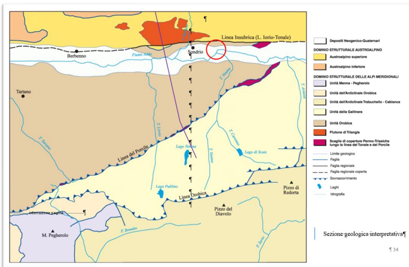
Figura 4 – MODELLO GEOLOGICO - SCHEMA TETTONICO (Foglio CARG 1:50.000 056 SONDRIO)
