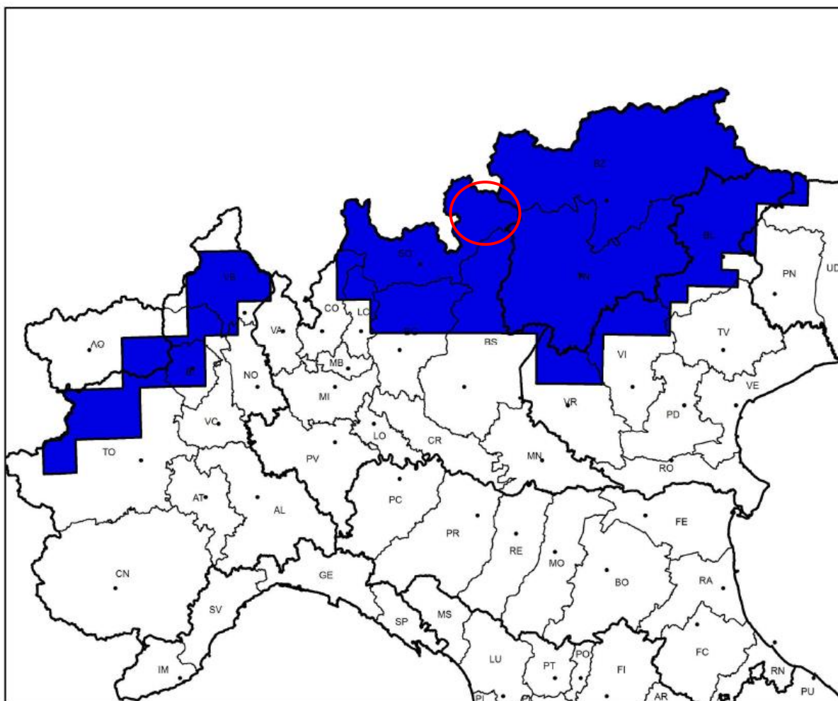
Figura 18 - Macroregione climatica 4 – Area alpina (cerchiata in rosso l'area di progetto)
