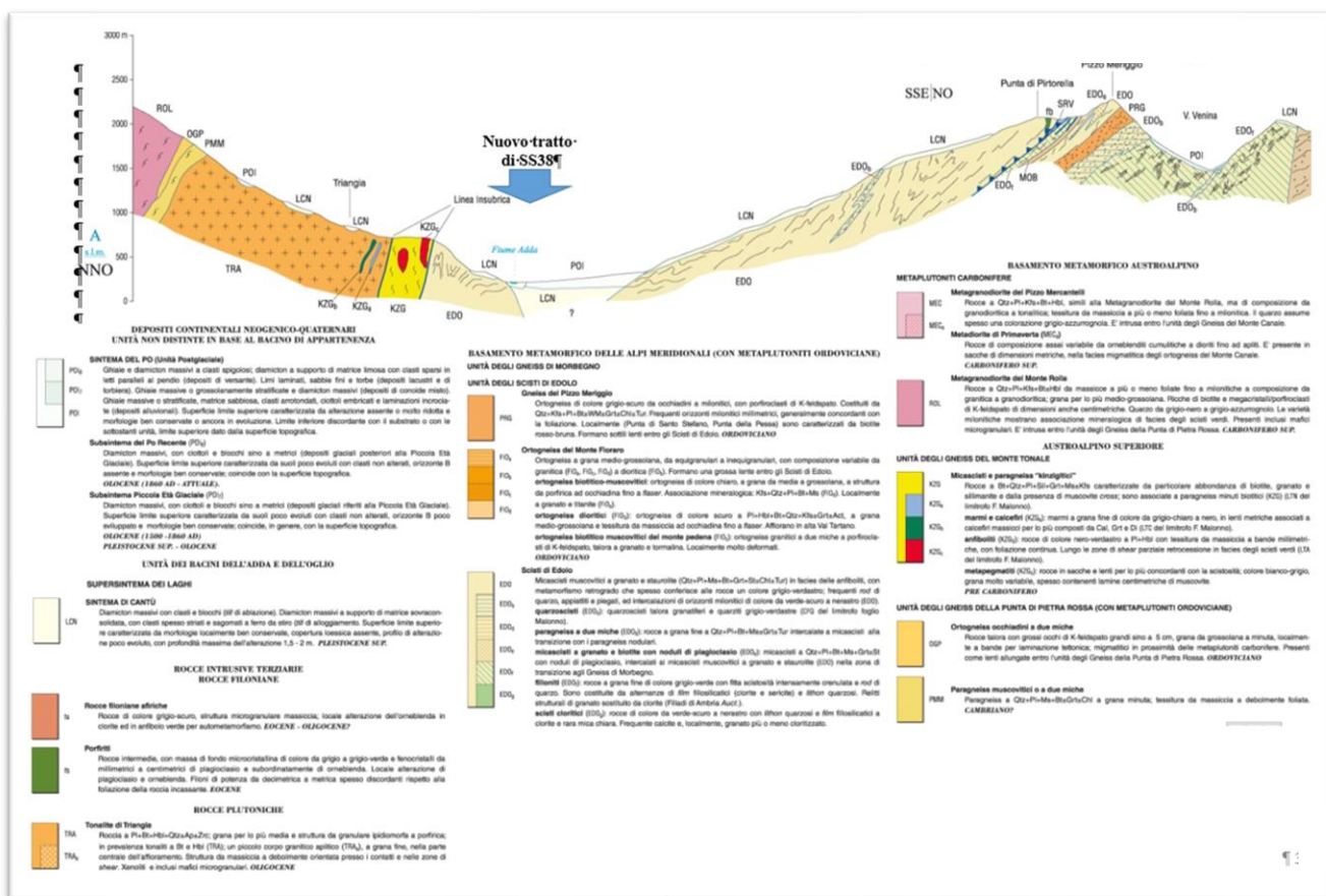
Figura 31 - MODELLO GEOLOGICO - SEZIONE GEOLOGICA INTERPRETATA (CARG 1:50.000 056 SONDRIO)
