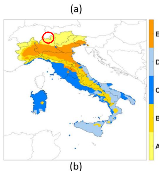
Figura 20 - Cluster anomalie (scenario RCP8.5)
