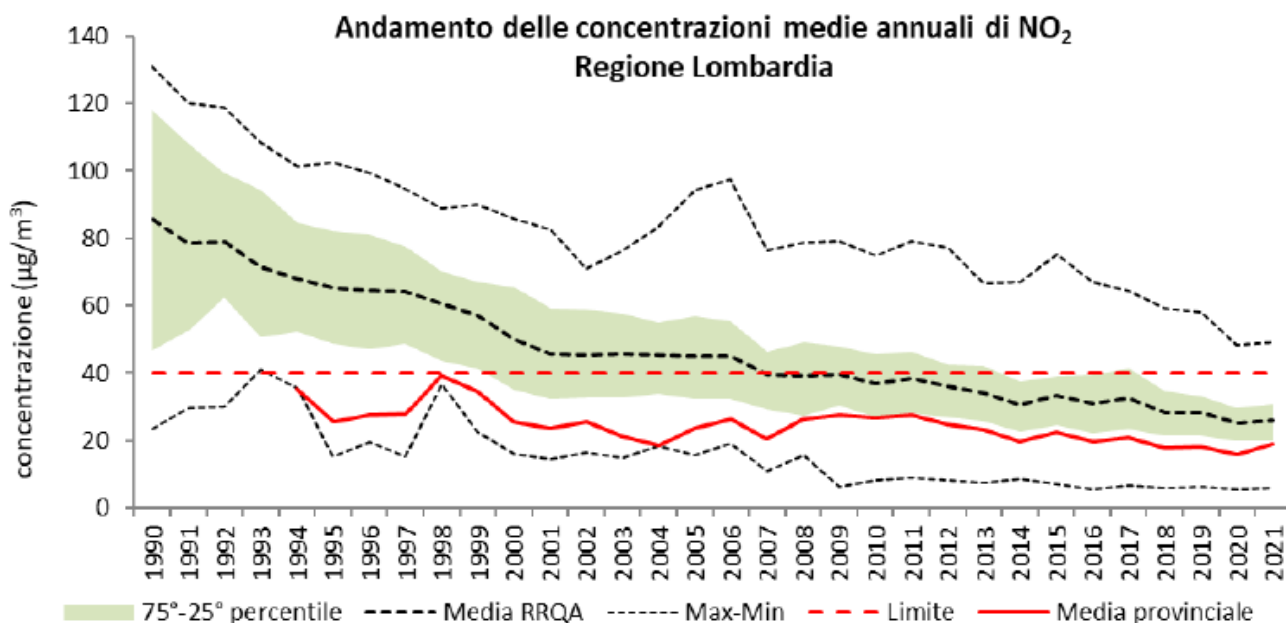
Figura 10 - Andamento delle concentrazioni medie annuali di NO 2 della regione confrontato con il trend della provincia di Sondrio
