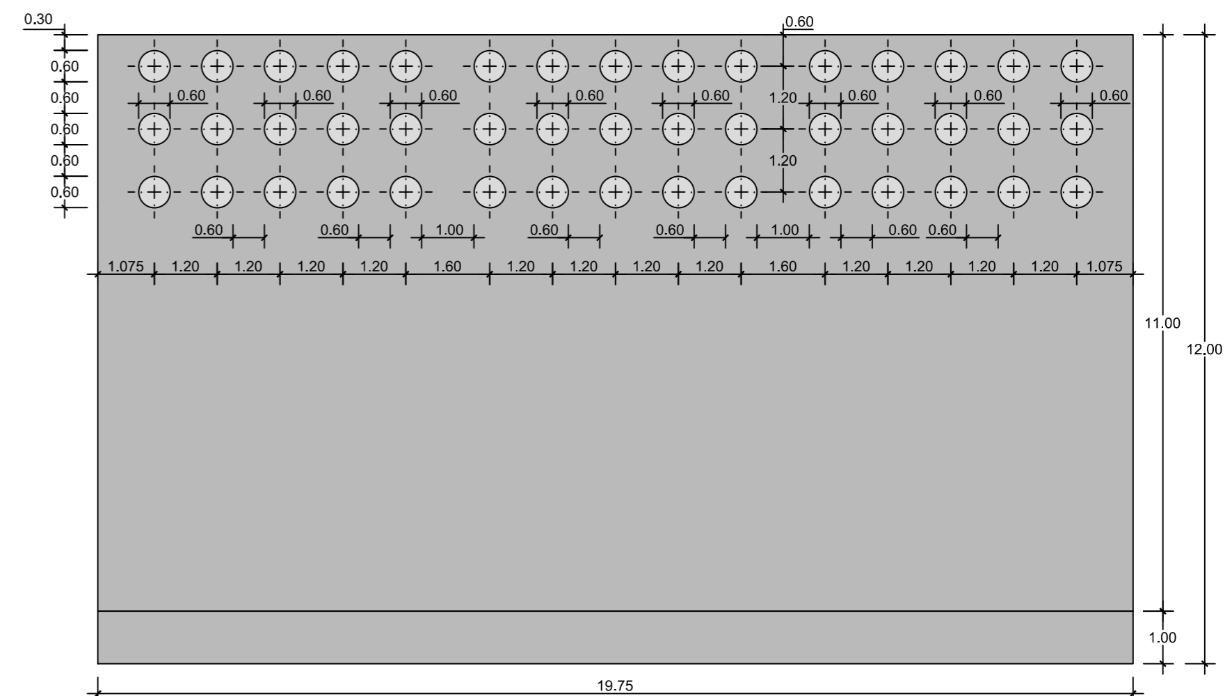
Vista frontale
