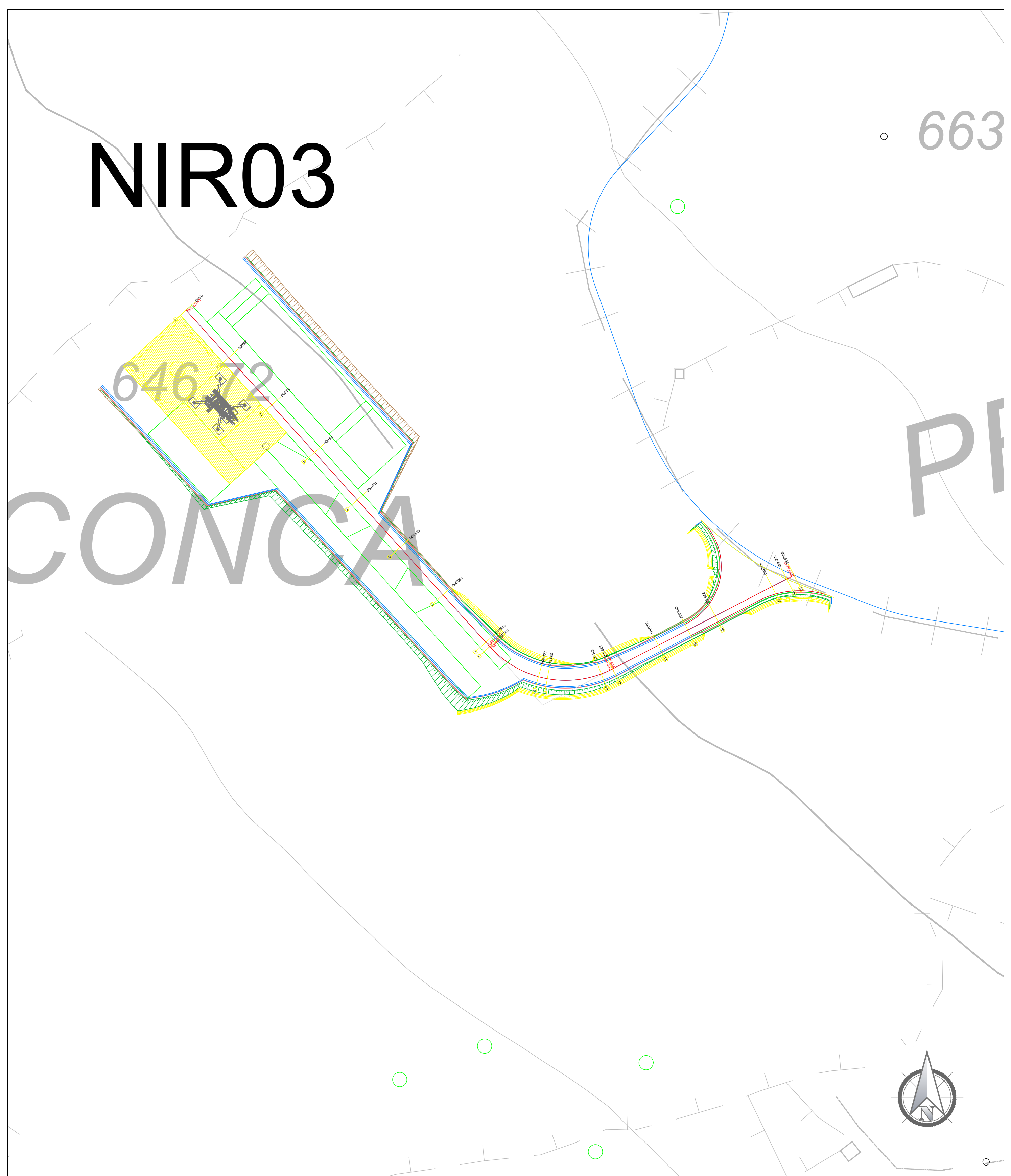
PLANIMETRIA VIABILITA' DI SERVIZIO AEROGENERATORE E RELATIVA PIAZZOLA Scala 1:1'000
