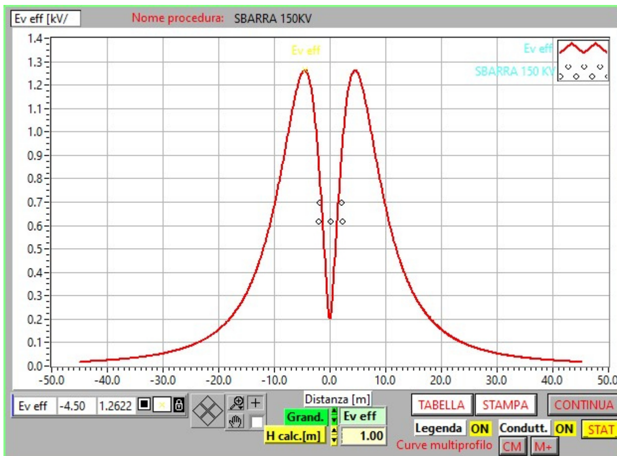
Campo elettrico generato dalla sbarra sempre inferiore a 2.5 kV/m.
