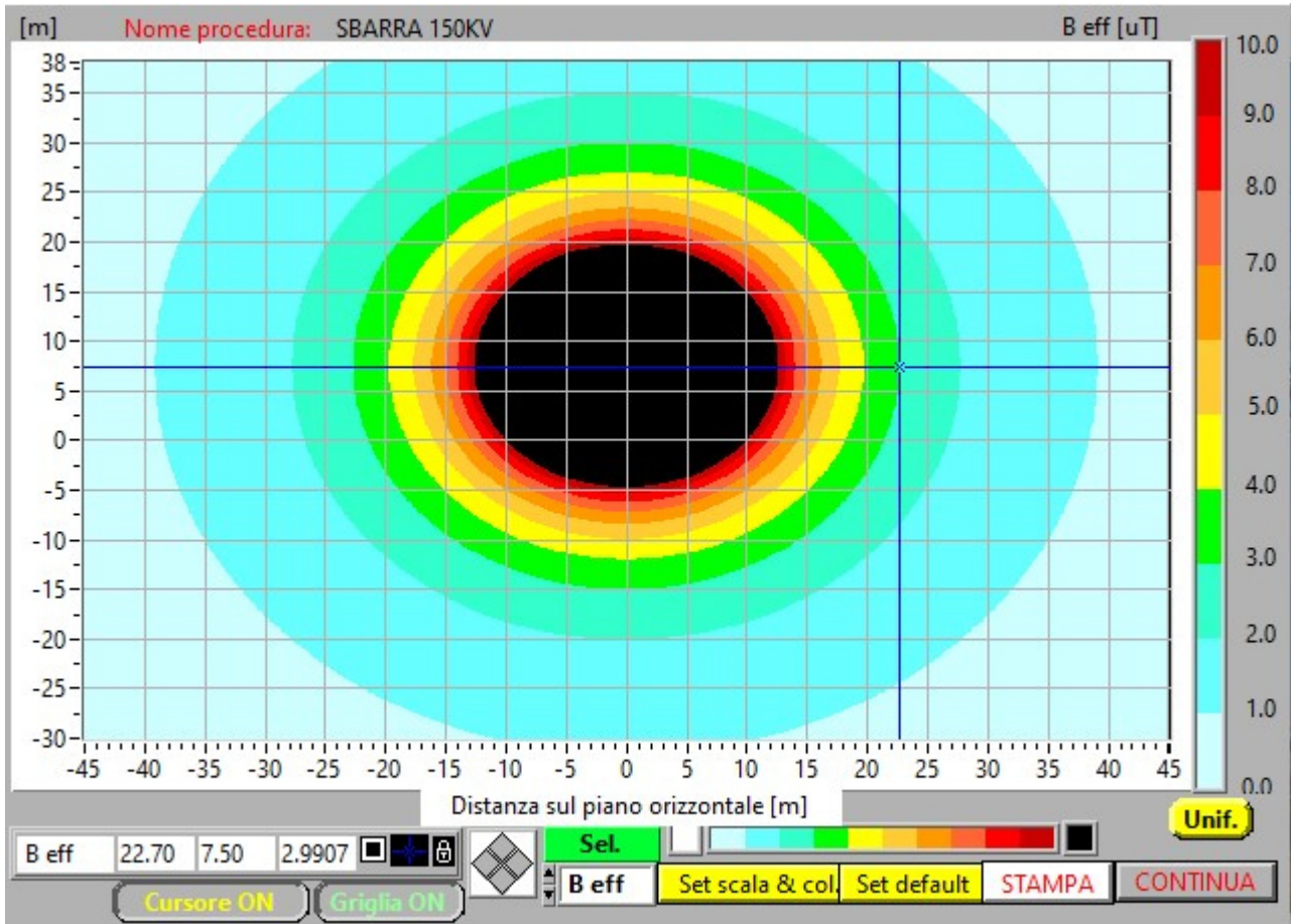
Campo elettromagnetico generato dalla sbarra
