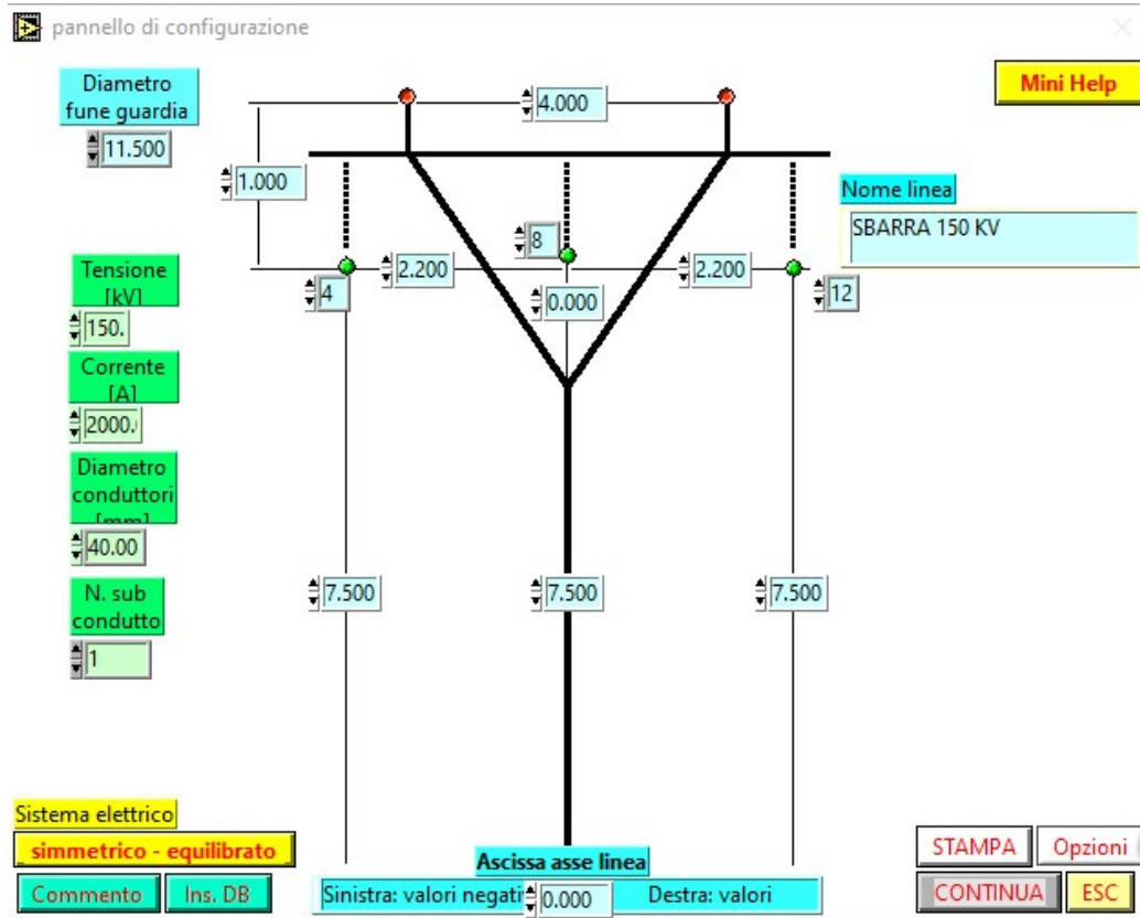
Configurazione geometrica sbarra
