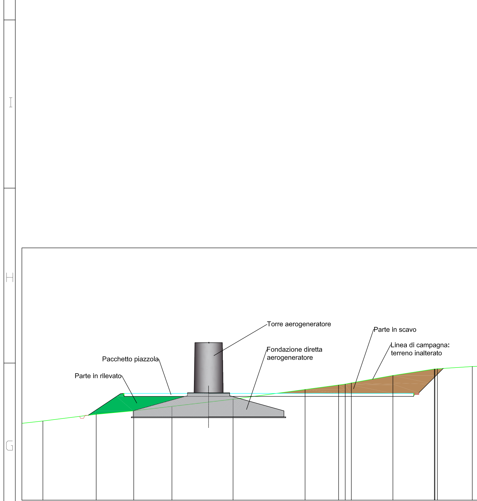
LEGENDA LAVORAZIONI SEZIONI TRASVERSALI
