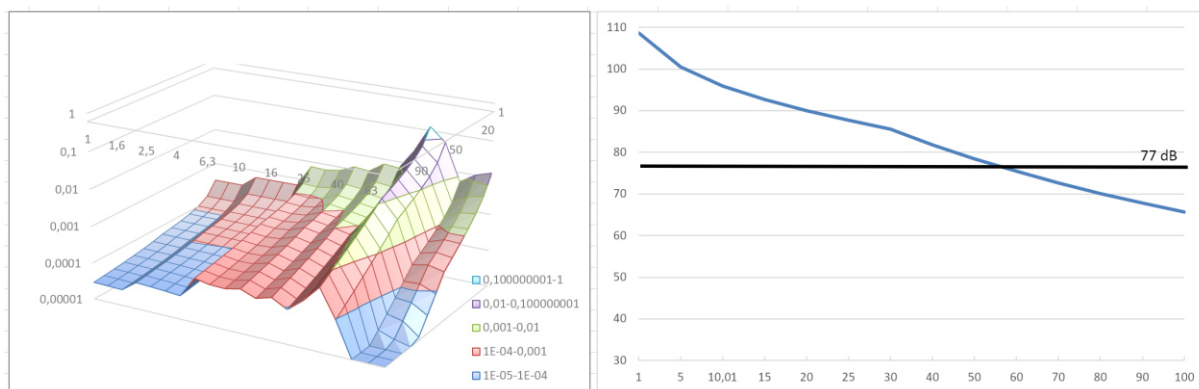
Figura 31 Modifica dello spettro dell'accelerazione ponderata in funzione della distanza e della frequenza e curva di propagazione delle vibrazioni
