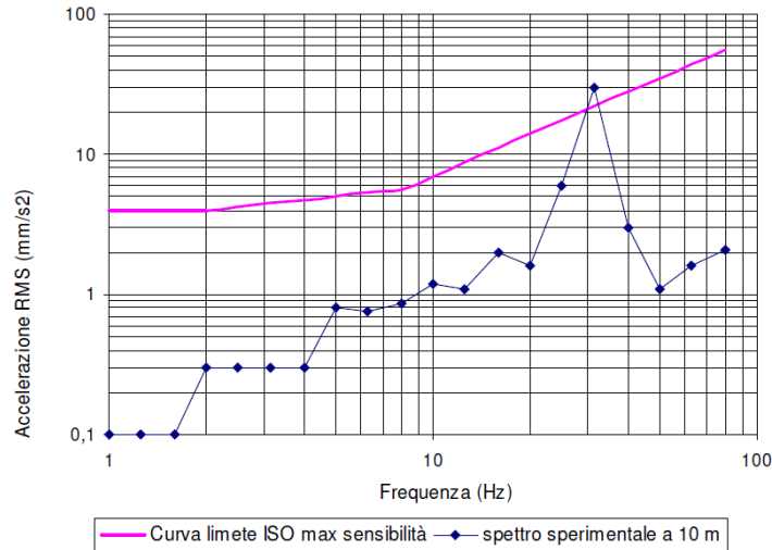
Figura 22 Spettro di emissione della sorgente di un rullo vibrante a 10m dall'asse di cantiere
