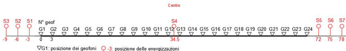
Figura 13 Geometria di acquisizione - MASW con 24 geofoni, interdistanza di 3,0 m, lunghezza complessiva 69,0
