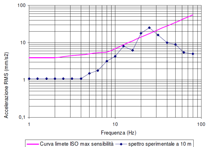
Figura 24 Spettro di emissione della sorgente di una pala cingolata a 10m dall'asse di cantiere
