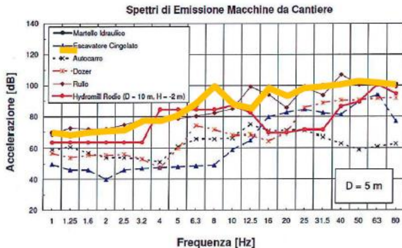
Figura 30 Spettro di emissione della sorgente di un martello idraulico 5m dall'asse di cantiere
