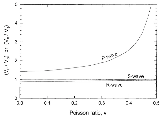
Figura 16 - rapporto tra le velocità di propagazione V_p e V_r
