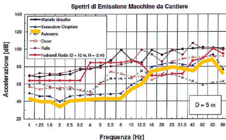
Figura 28 Spettro di emissione della sorgente di un escavatore cingolato 5m dall'asse di cantiere
