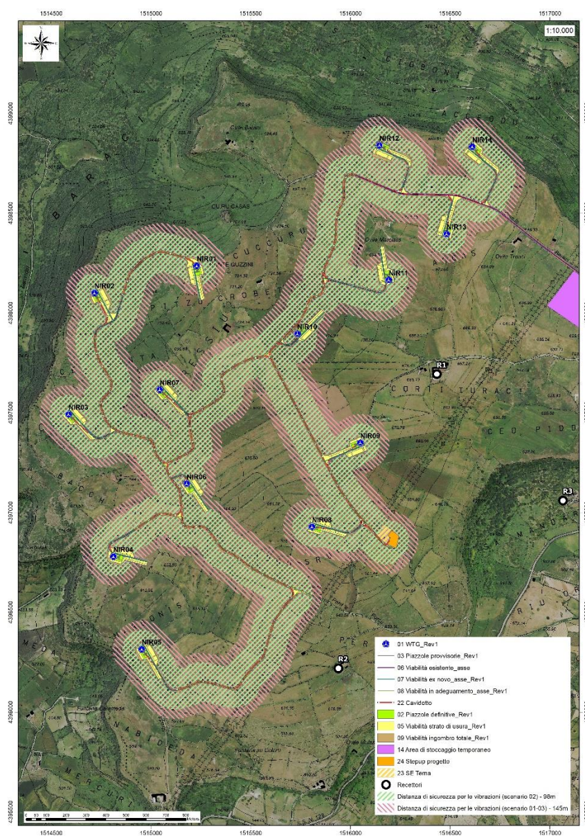
Figura 17 Distanze di sicurezza per le vibrazioni nei vari scenari
