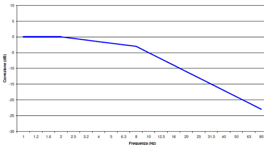
Figura 14 - Curva di ponderazione asse generico
