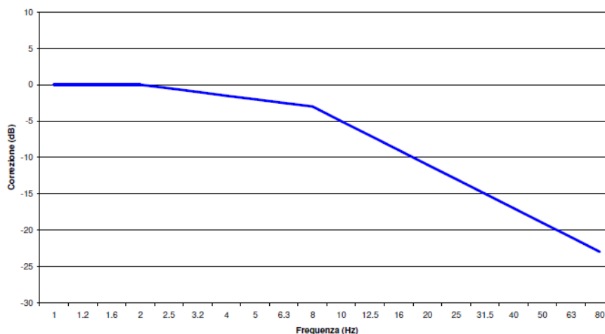
Figura 20 Curva di ponderazione per un asse generico - UNI 9614
