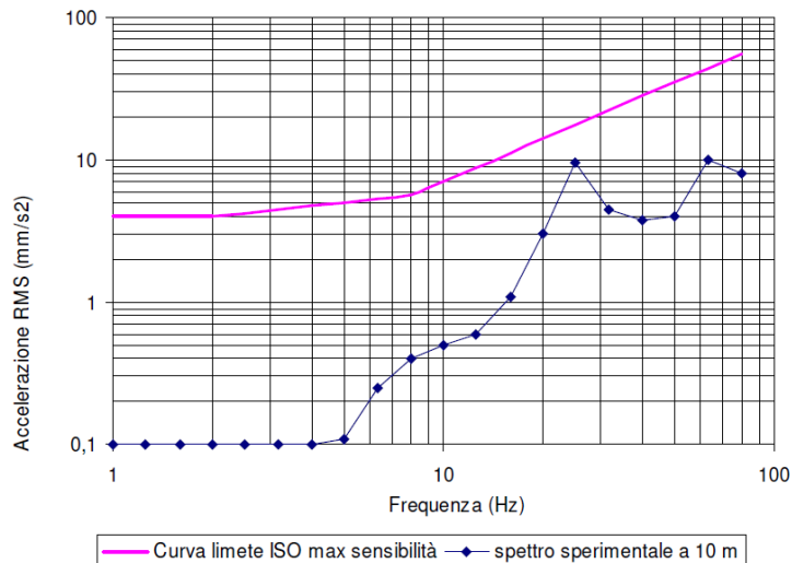
Figura 26 Spettro di emissione della sorgente di un autocarro 10m dall'asse di cantiere
