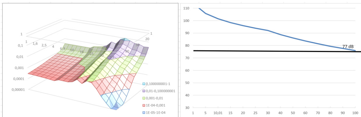
Figura 29 Modifica dello spettro dell'accelerazione ponderata in funzione della distanza e della frequenza e curva di propagazione delle vibrazioni
