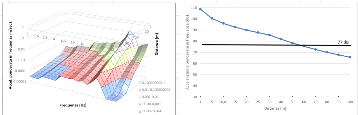
Figura 22 Spettro di emissione della sorgente di un rullo vibrante a 10m dall'asse di cantiere
