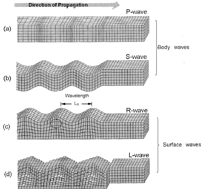
Figura 15 - Tipologia di onde: a) e b) onde di volume, c) e d) onde di superficie
