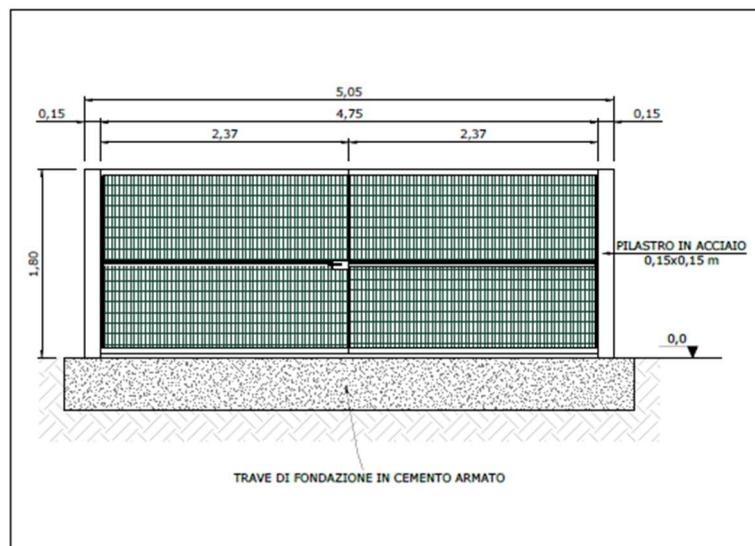
Fig. 17 – Cancello carrabile
