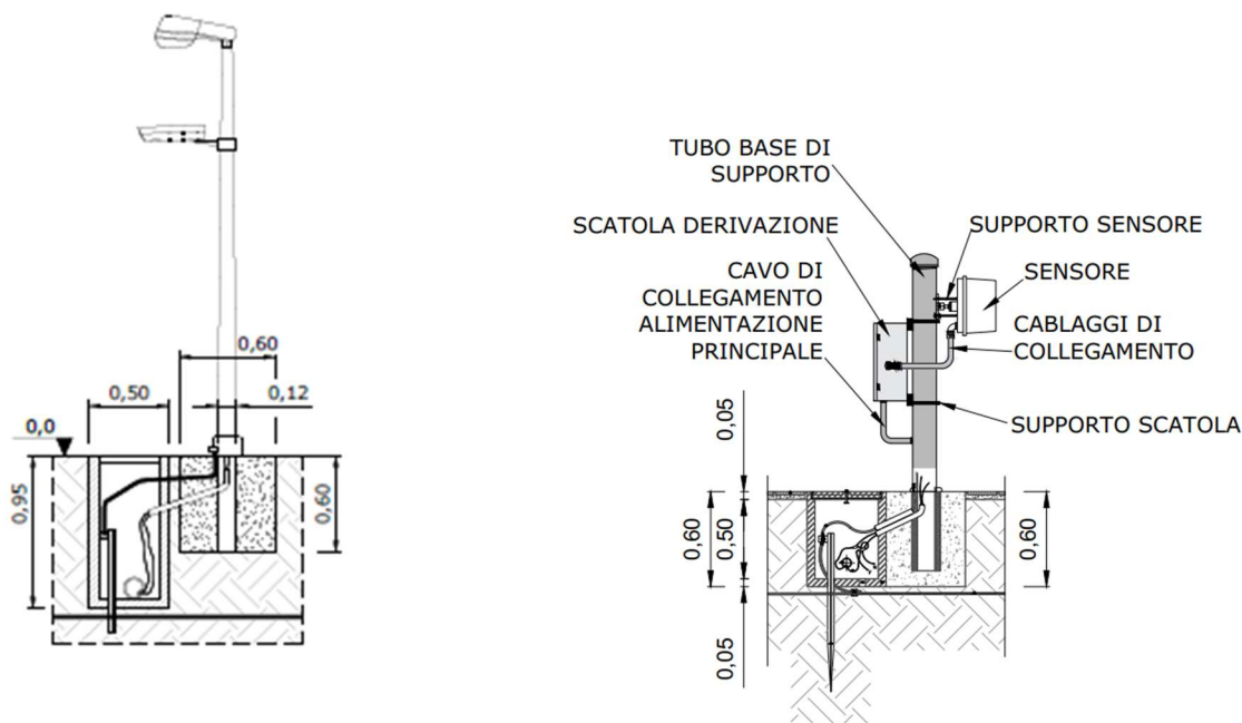
Fig. 19 – Sistema antintrusione
