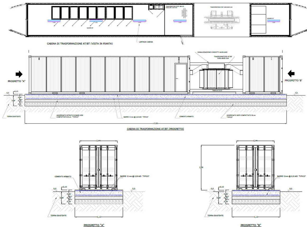
Fig. 12 - Cabina di trasformazione BT/AT
