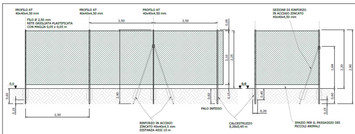
Fig. 16 – Particolare della recinzione
