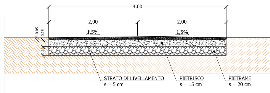
SEZIONE TIPO VIABILITA' INTERNA / ESTERNA
