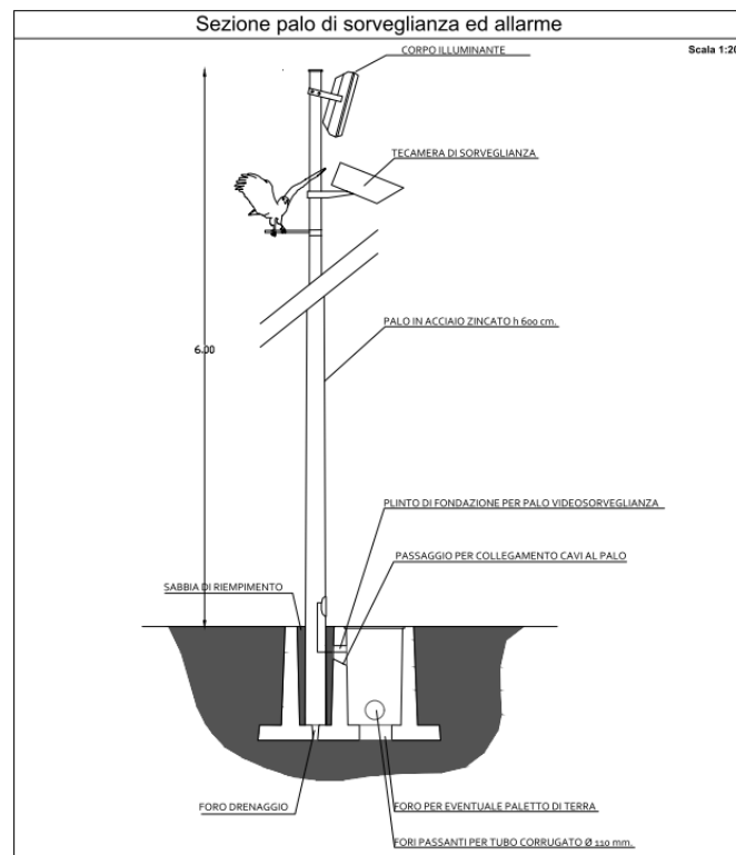
Figura 10: Sezione tipo palo di sorveglianza ed allarme
