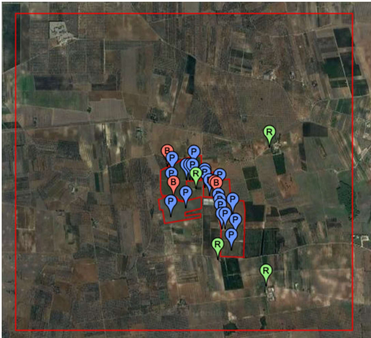
SORGENTI DI RUMORE e RECETTORI
