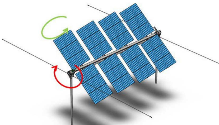
Figura 30: struttura in acciaio che sostiene i pannelli verticali e ne permette la rotazione.
