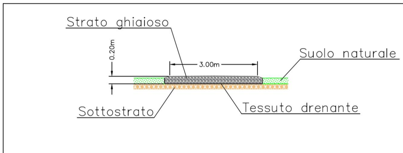
Figura 23: particolare costruttivo viabilità.
