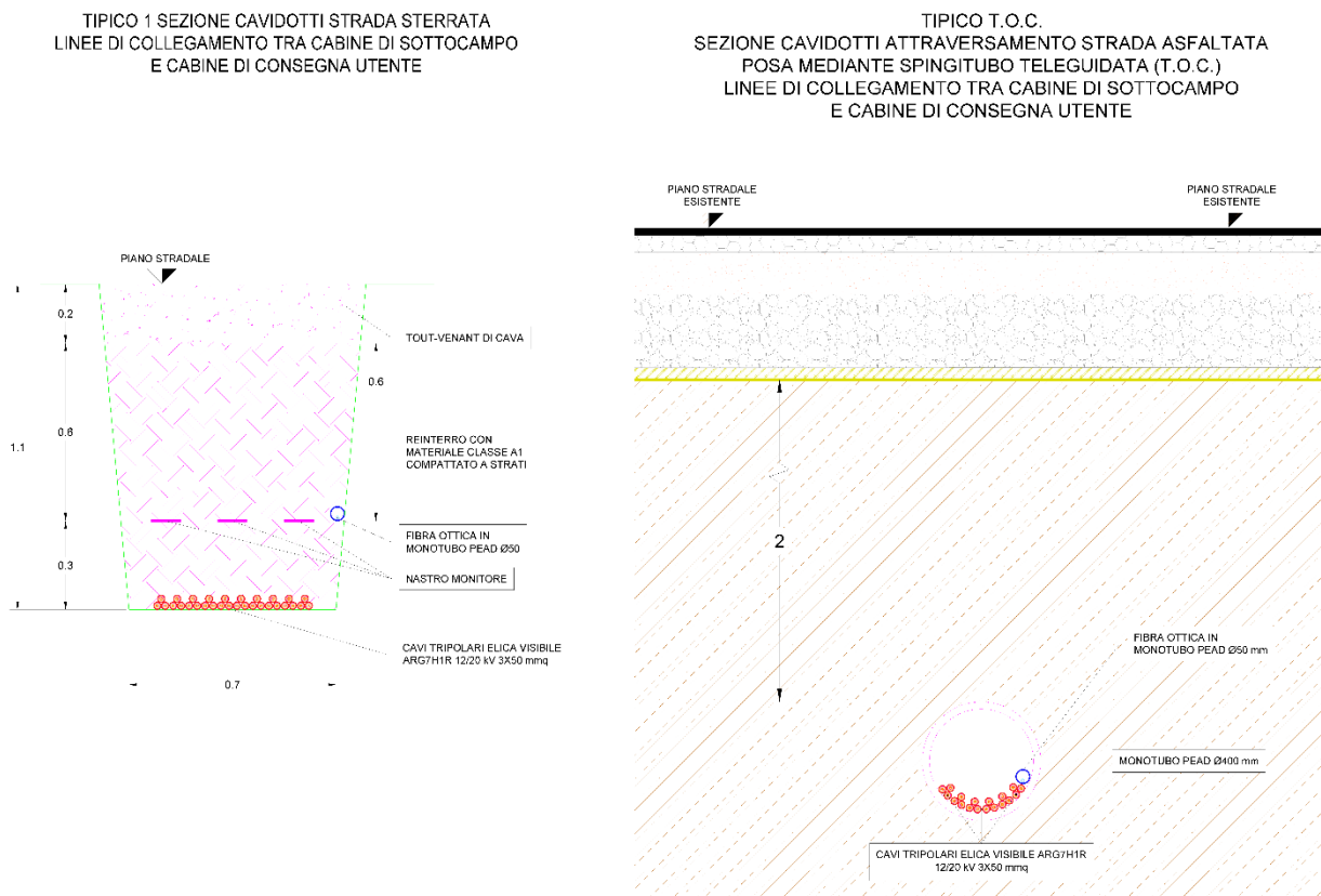
Figura 20: sezioni tipo dei cavidotti interrati
