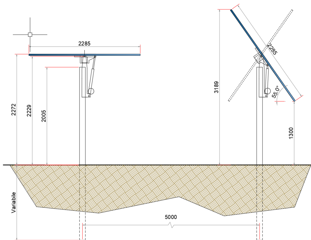
Figura 14: sezione trasversale di un tracker.
