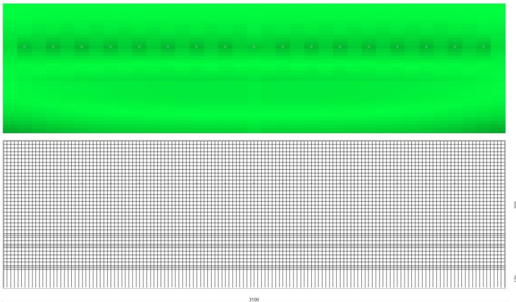
Fig. 15 - Piastra paramento dir. Y (Inviluppo)
