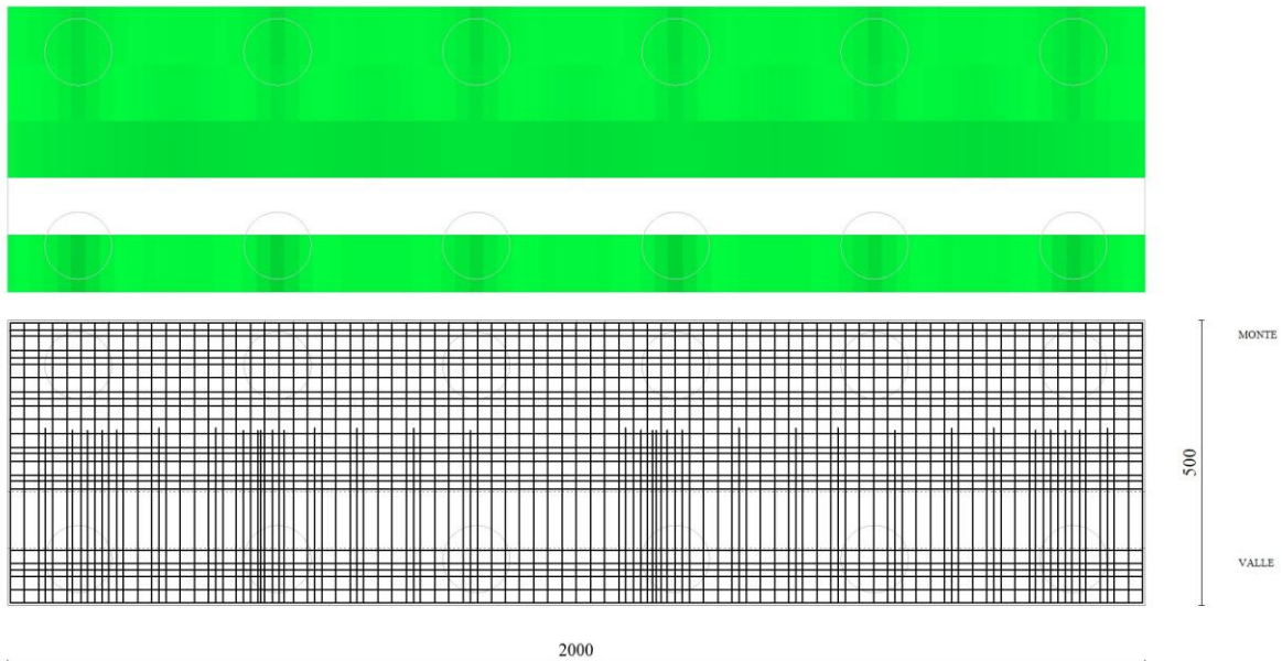
Fig. 13 - Piastra fondazione dir. X (Inviluppo)
