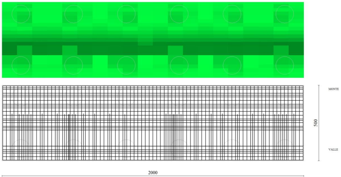
Fig. 9 - Piastra fondazione dir. Y (Inviluppo)
