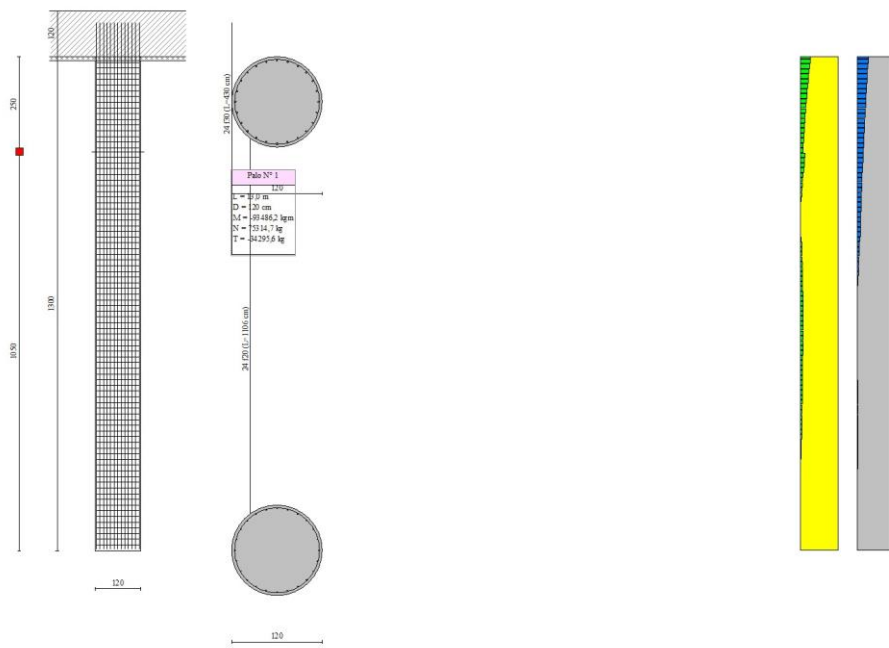
Fig. 15 - Pali (Palo n° 1) (Inviluppo)
