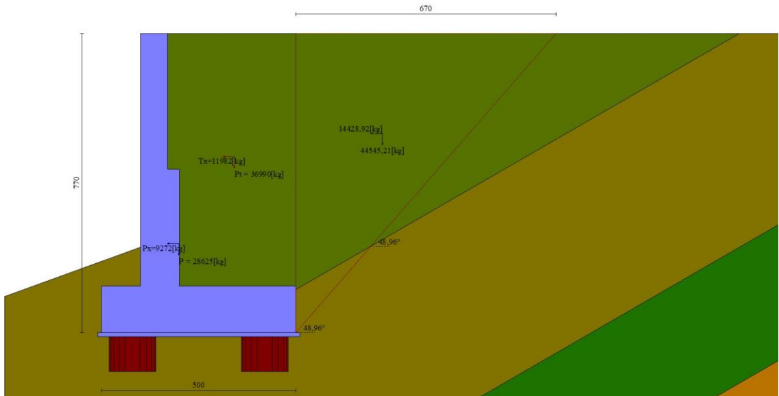
Fig. 4 - Cuneo di spinta (combinazione sismica) (Combinazione n° 2)
