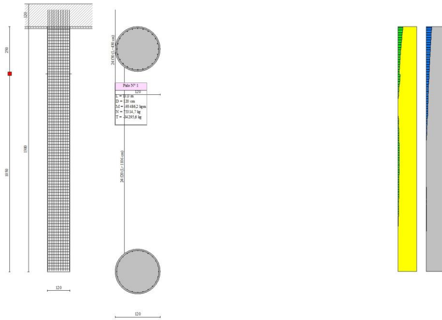
Fig. 10 - Pali (Palo n° 1) (Inviluppo)
