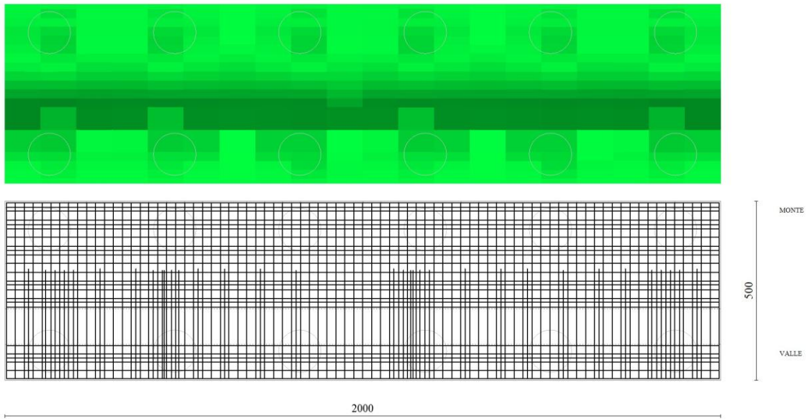
Fig. 14 - Piastra fondazione dir. Y (Inviluppo)
