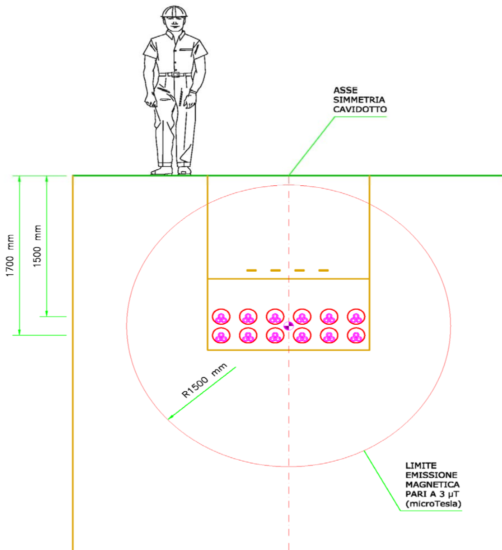
Volume di rispetto campo magnetico delle linee AT interrato in cavo elicordato.
