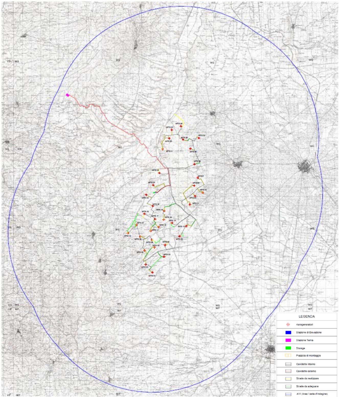
Inquadramento su IGM, scala 1:50.000
