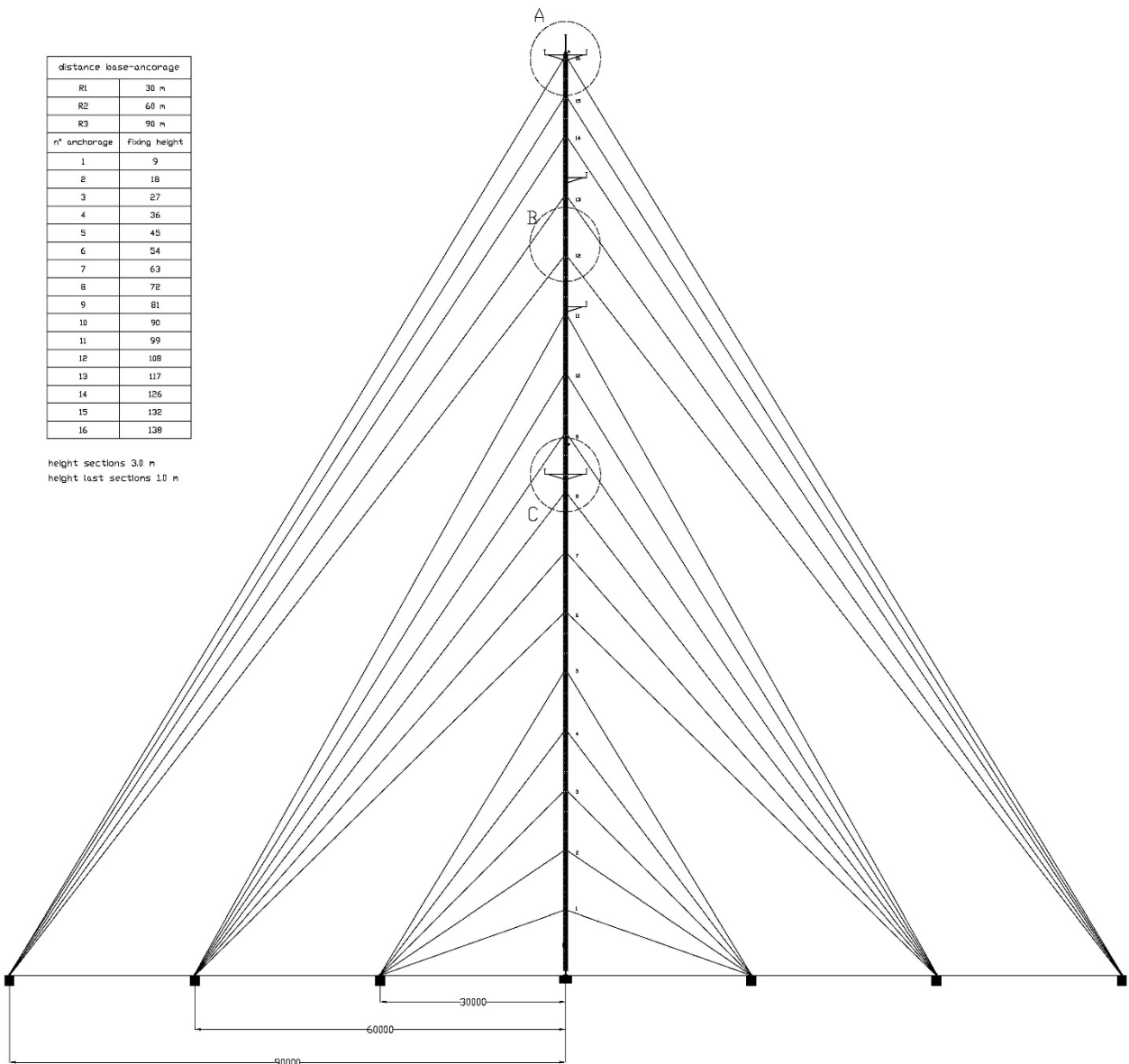
Torre anemometrica
