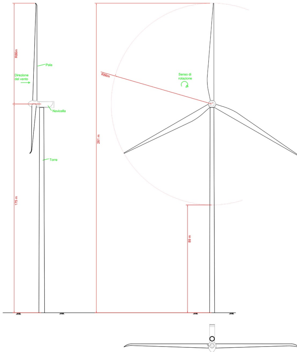
Aerogeneratore tipo: pianta, prospetto frontale e prospetto laterale
