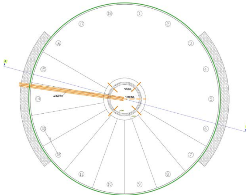
Sezione AA' - Concio di fondazione D=36m
