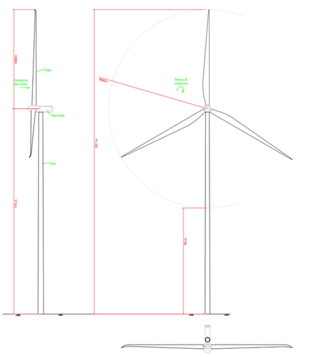
Aerogeneratore tipo: prospetto laterale, prospetto frontale e pianta
