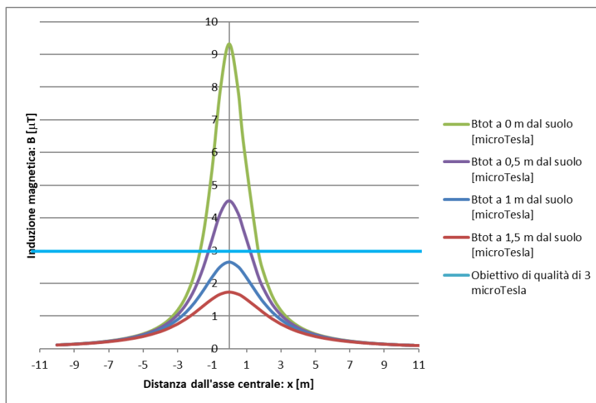
Figura 3: Andamento del campo magnetico generato dal cavidotto, composto da due terne da 630 mm 2 e una da 400 mm 2
