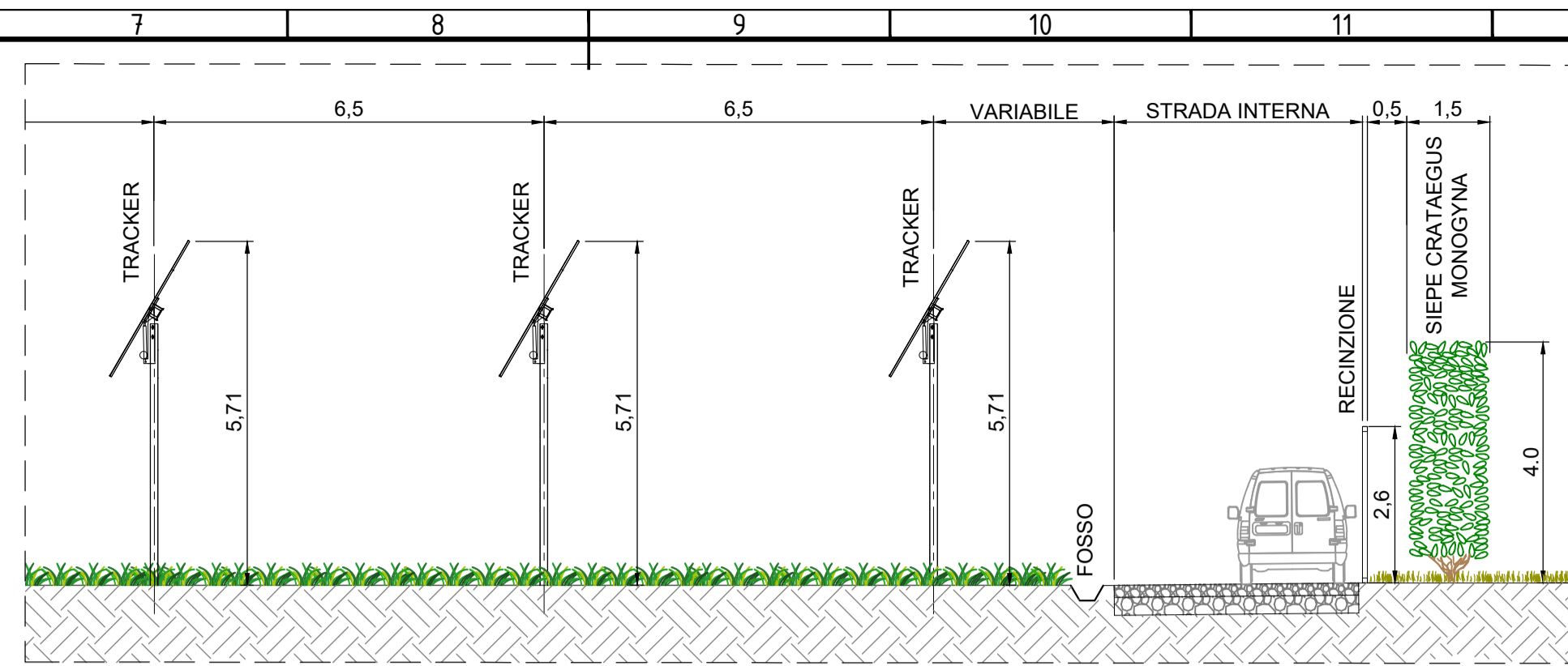
SEZIONE TIPO IN CORRISPONDENZA PANNELLI FOTOVOLTAICI CON TIPOLOGIA AD INSEGUIMENTO (TRACKER) Scala 1:100
