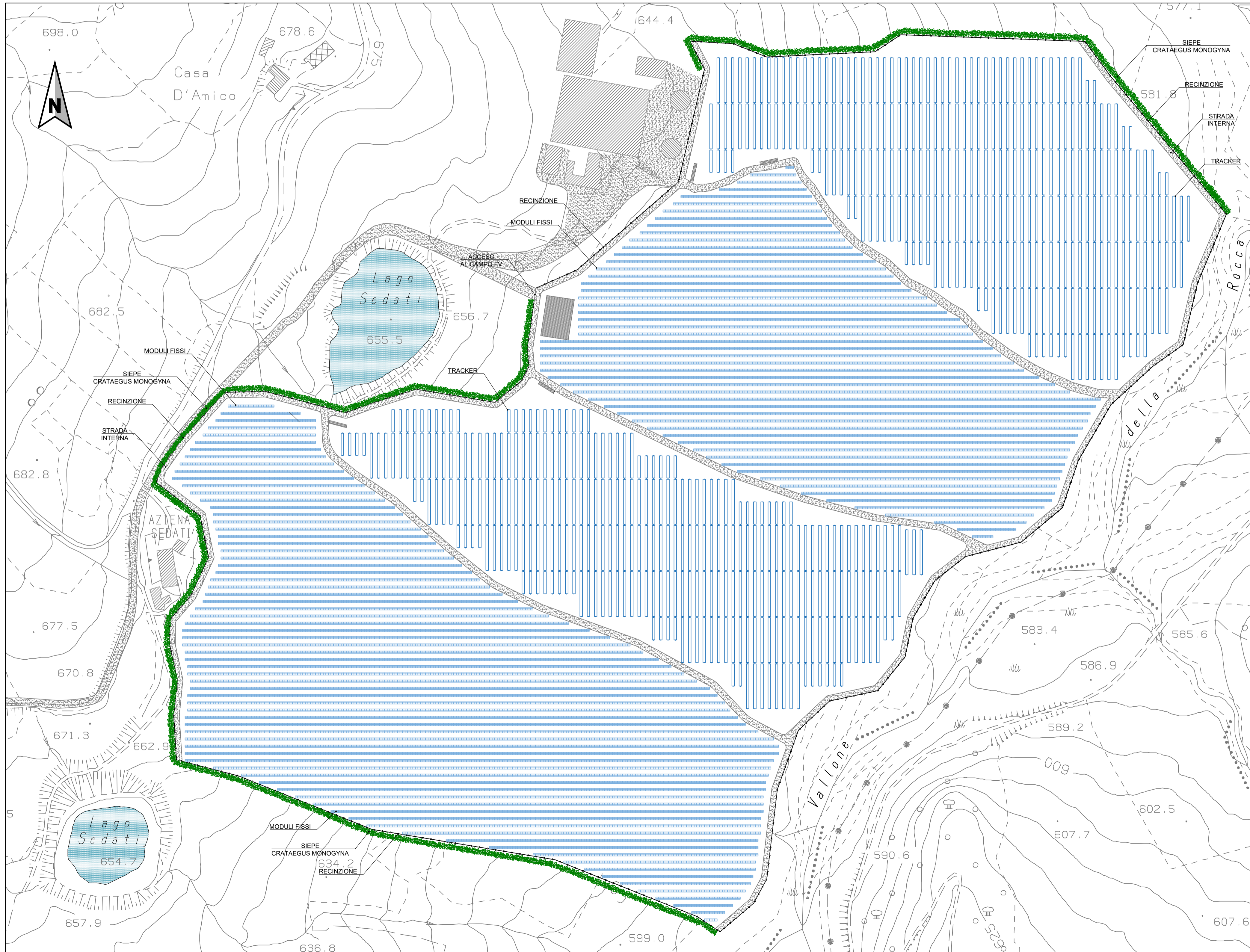
ESTRATTO PLANIMETRICO Scala 1:2000
