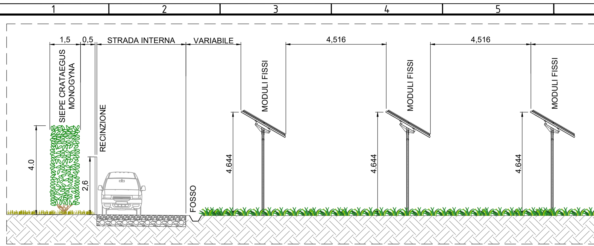
SEZIONE TIPO IN CORRISPONDENZA PANNELLI FOTOVOLTAICI IN TIPOLOGIA FISSA Scala 1:100
